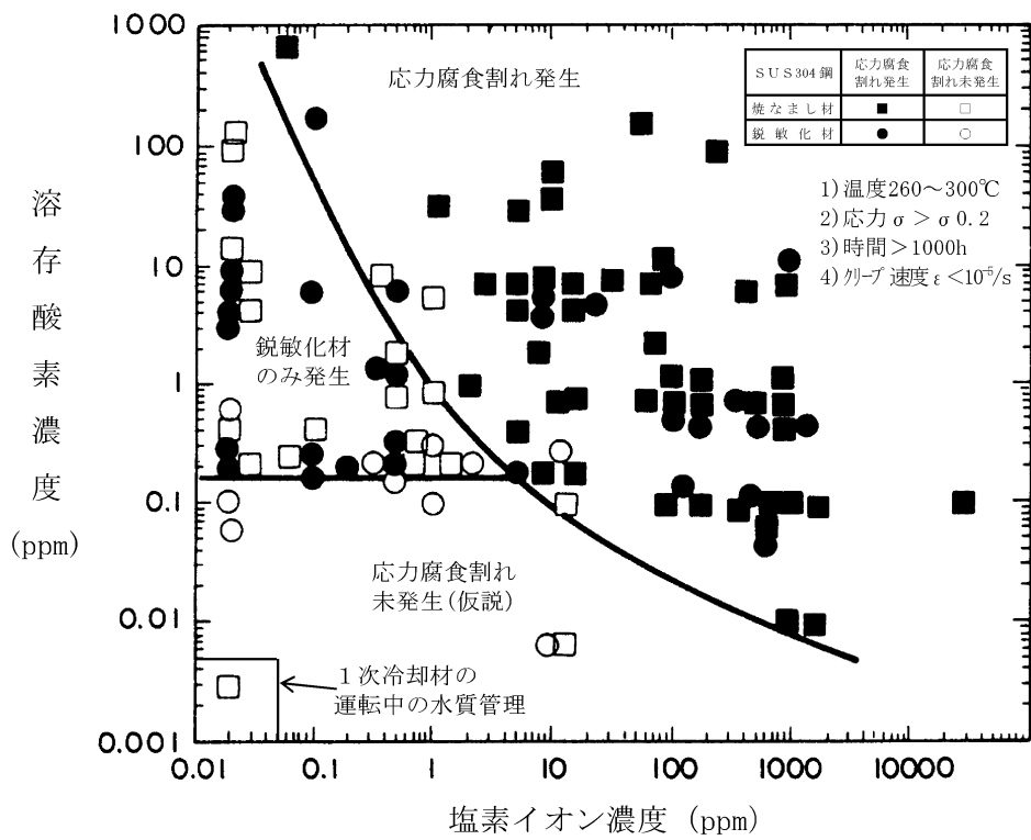
図 8-5 SUS304 鋼の応力腐食割れ発生におよぼす塩素イオン濃度及び溶解酸素濃度の限界量 (65)
