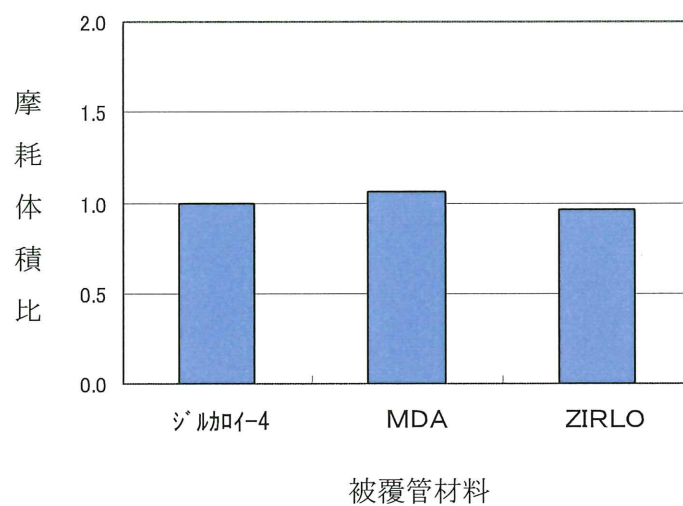
図 3-38 ジルカロイ-4 支持格子との組合せにおける被覆管材料の摩耗体積比の比較
