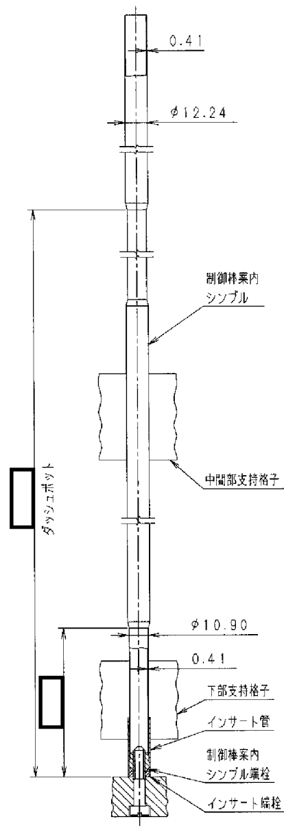
制御棒案内シンプル
