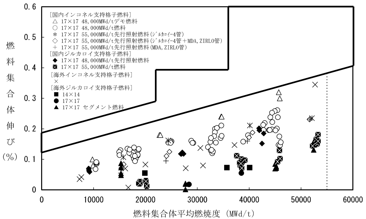
図 3-32 燃料集合体伸び (11)、(53) ~ (56)、(58)
