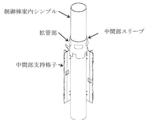
(b) 制御棒案内シンプル と中間部支持格子の結合
