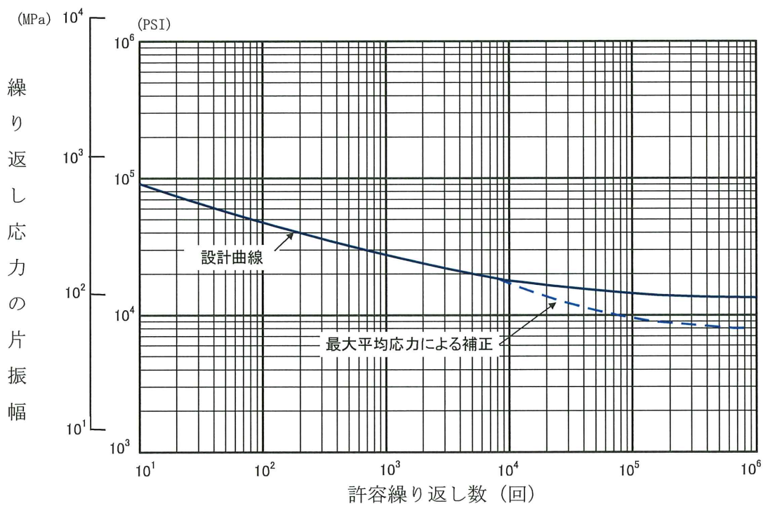
図 3-25 ジルカロイ-4 の設計疲労曲線 (50)
