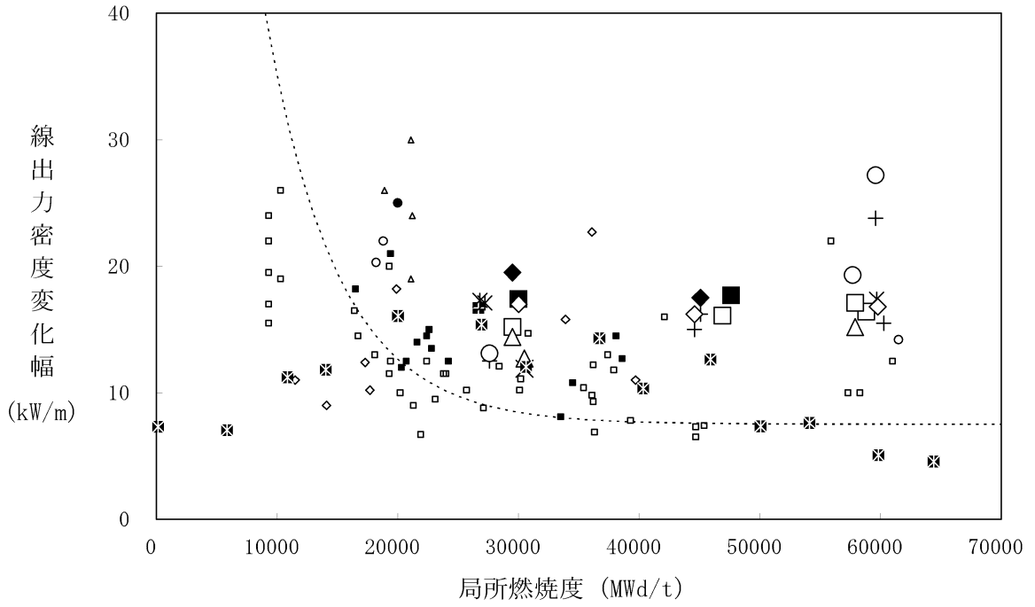
図 3-36 (2) 被覆管の出力ランプ試験結果 (9)、(11)、(16)、(57) (線出力密度変化幅が最大の場合の出力変化)
