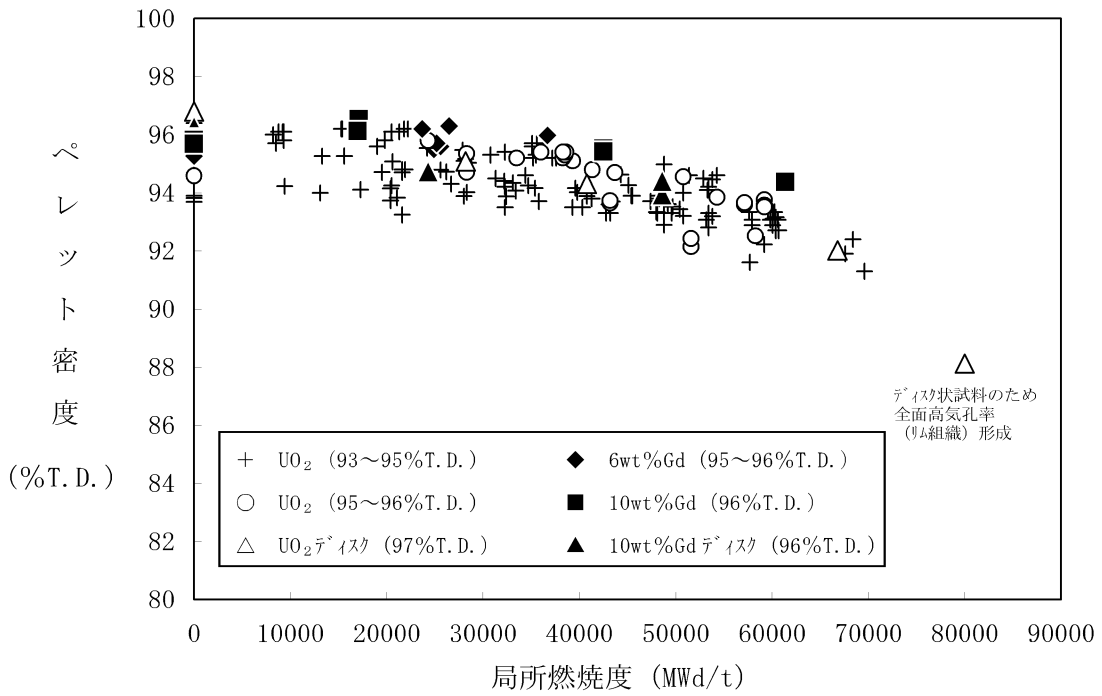
図 3-2 ペレット密度の燃焼に伴う変化 (8)~(16)
