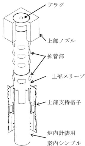
(d) 炉内計装用案内シンプル と上部ノズル及び 上部支持格子の結合
