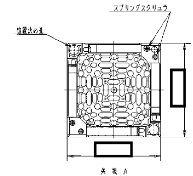
矢視 A
