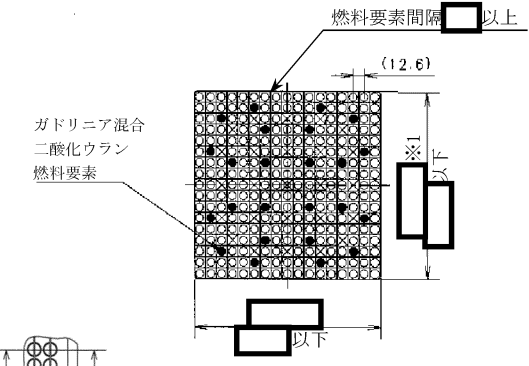
断面 B-B (ガドリニア混合二酸化ウラン燃料要素配置)
