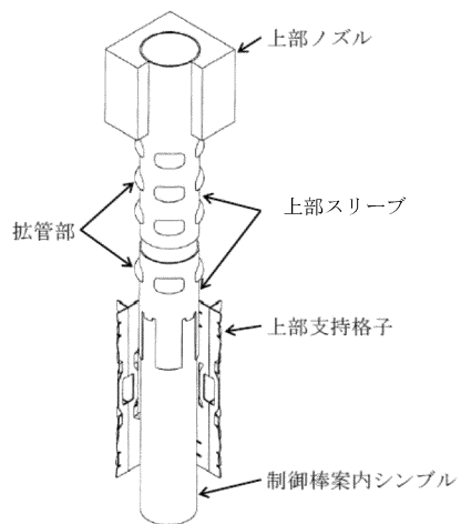
(a) 制御棒案内シンプルと上部ノズル 及び上部支持格子の結合
