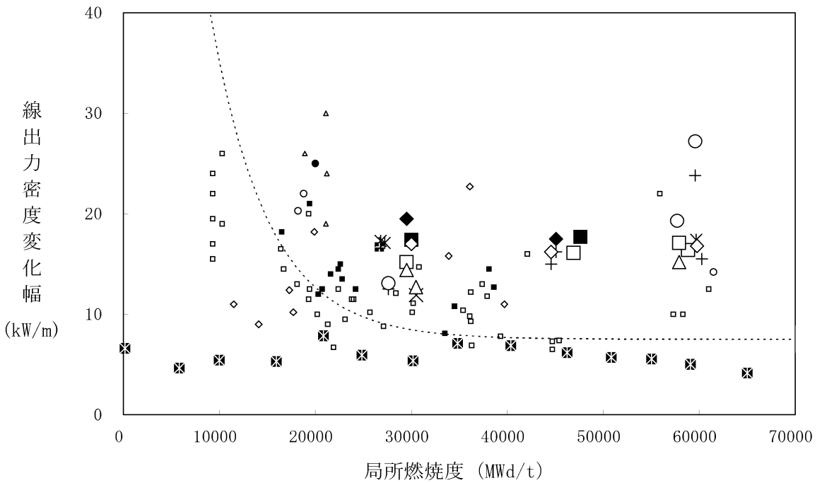
図 3-36 (1) 被覆管の出力ランプ試験結果 (9)、(11)、(46)、(57)
