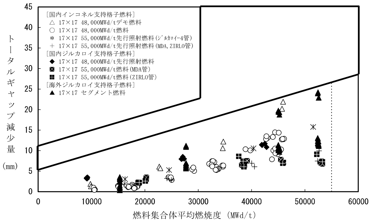
図 3-33 トータルギャップ減少量 (11)、(58)
