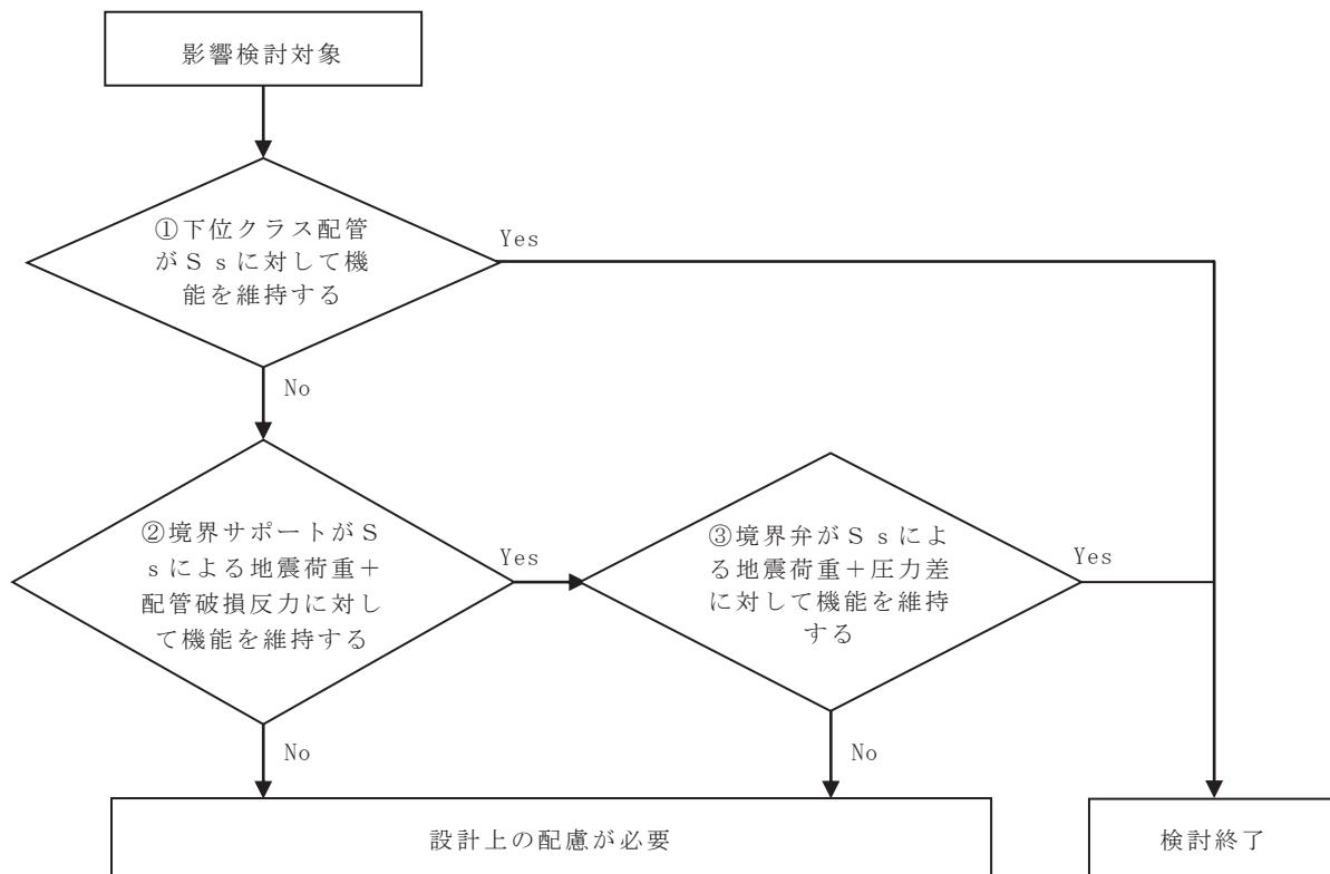
添付 8-3 図 下位クラス施設損傷に伴う機械的荷重の影響検討フロー
