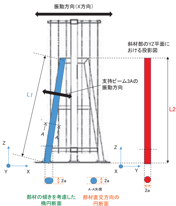
添付9-5図 斜材（支持ビーム3A）に対する付加質量算出の考え方
