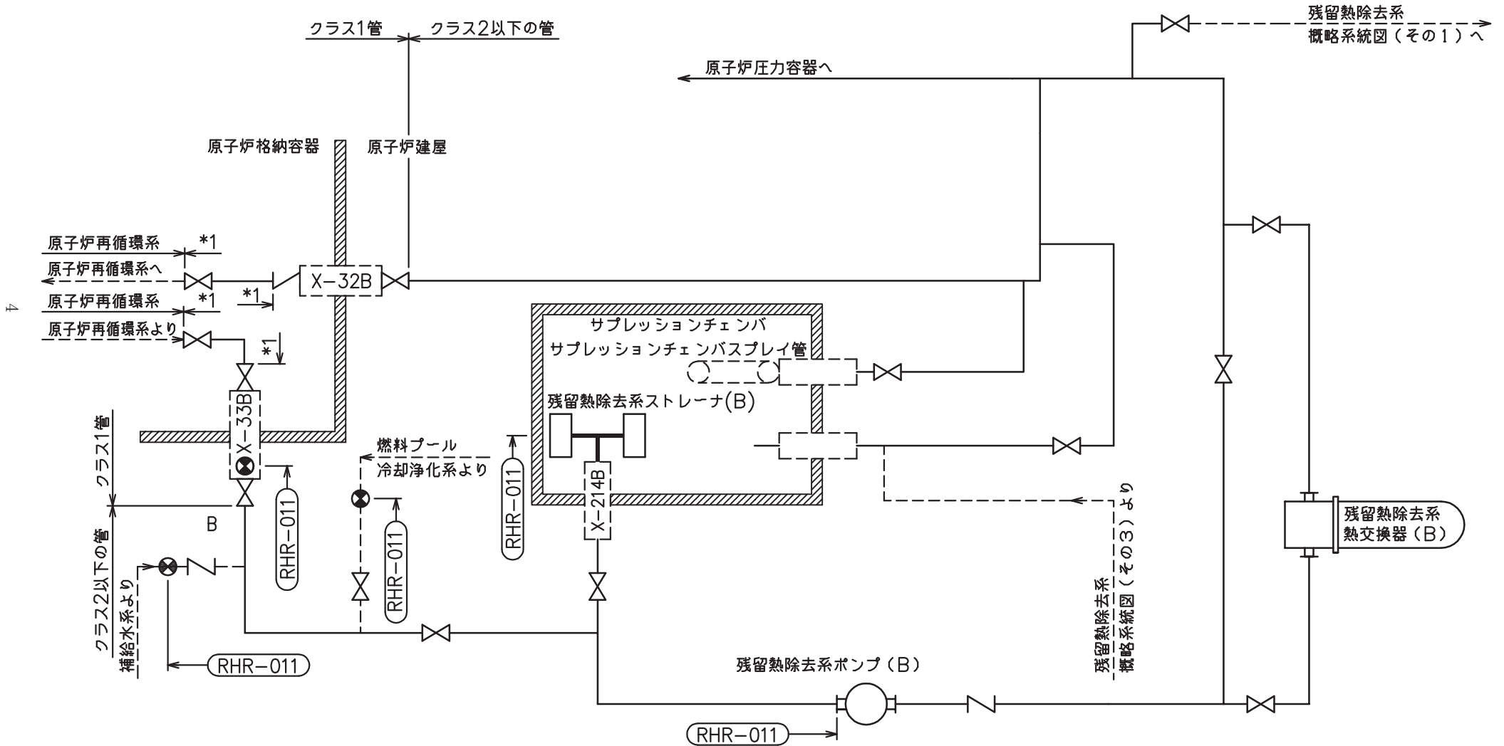
残留熱除去系概略系統図(その2)
