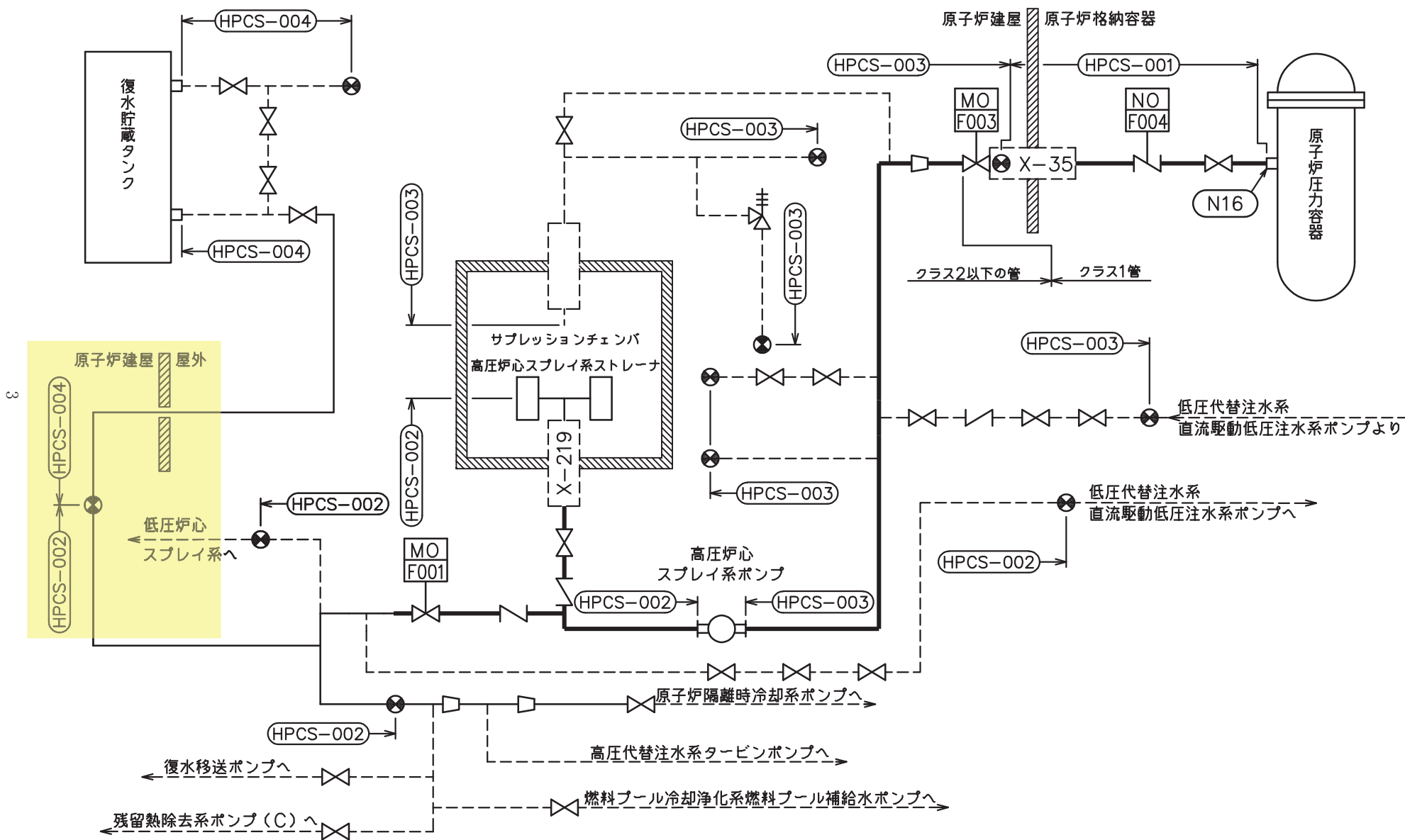
高圧炉心スプレー系概略系統図
