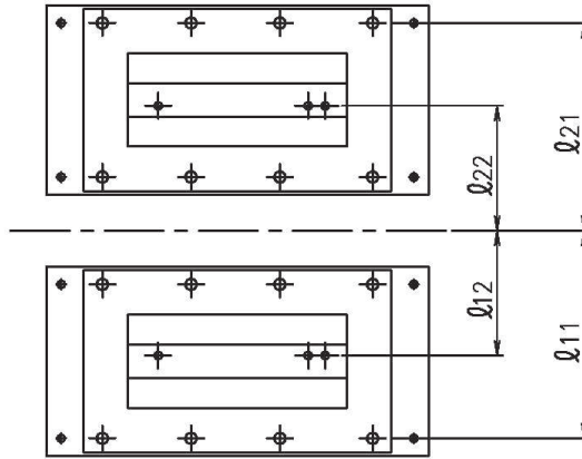
A~A矢視図
