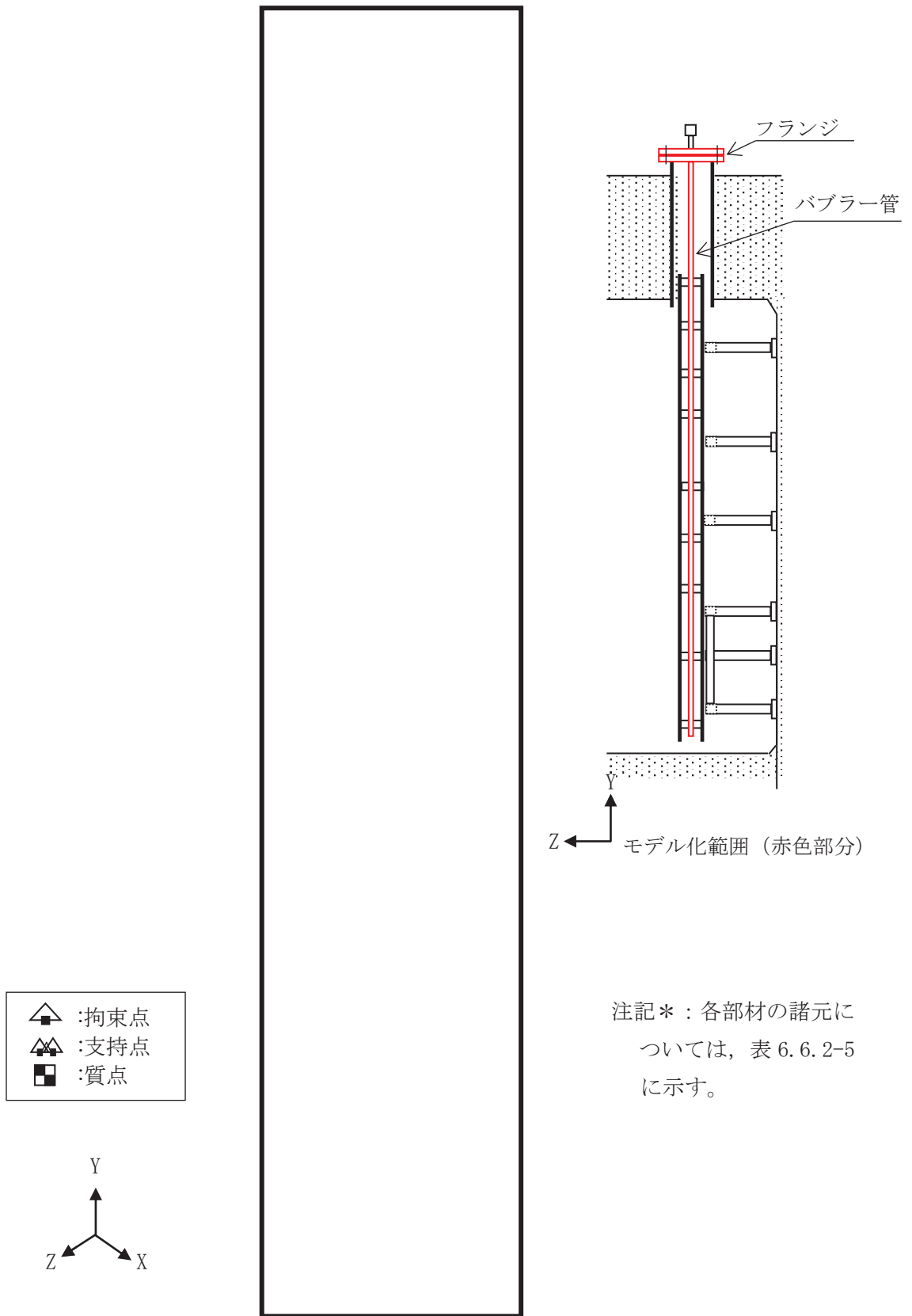
図 6.6.2-7 バブラー管解析モデル
