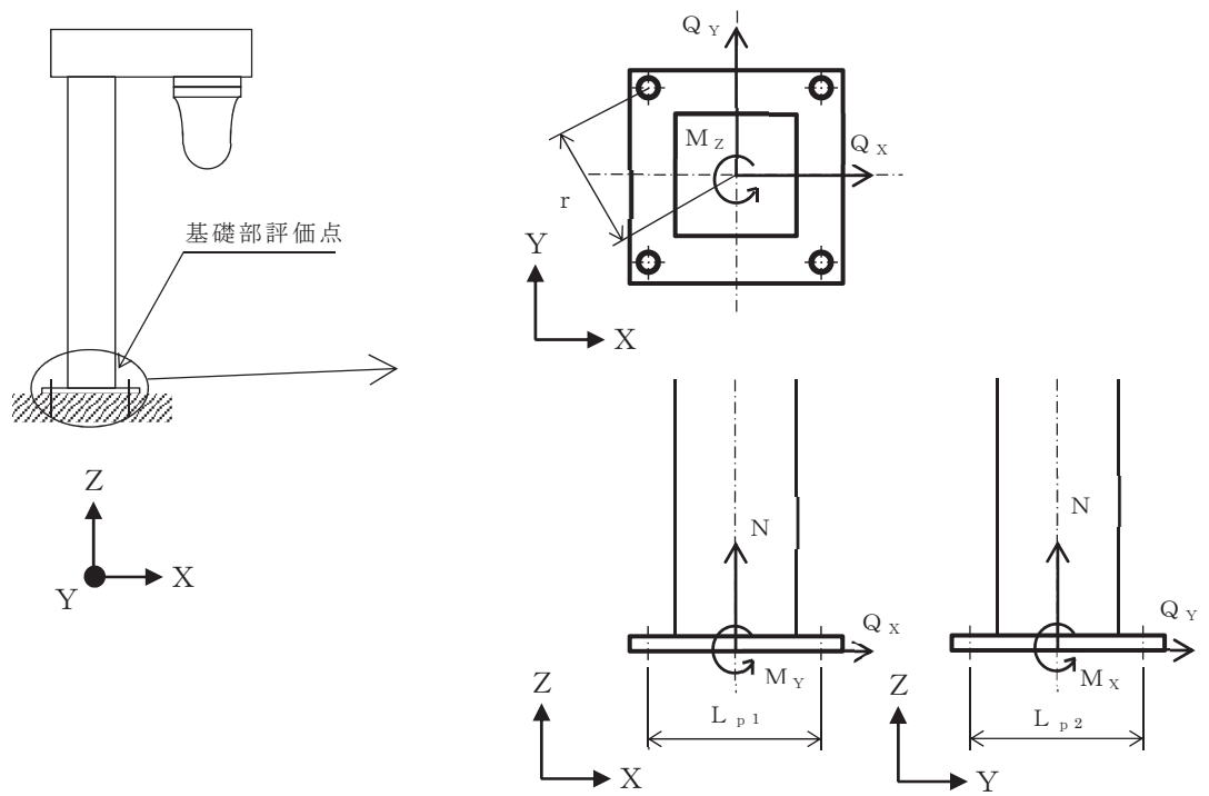
図 6.6.1-9 計算モデル（防潮堤 基礎ボルト）
