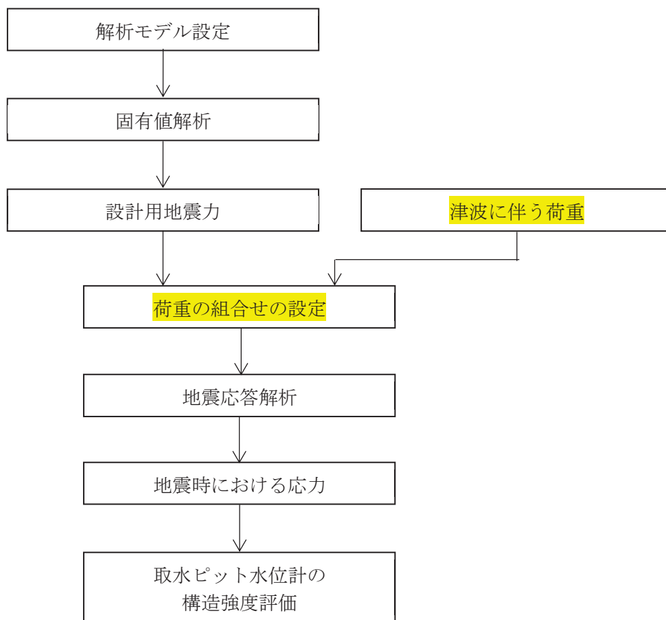
図 2-2 取水ピット水位計の強度評価フロー
