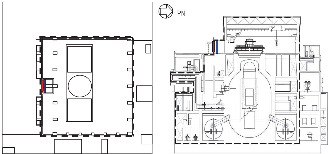
原子炉建屋原子炉棟地上 3 階概略平面図
