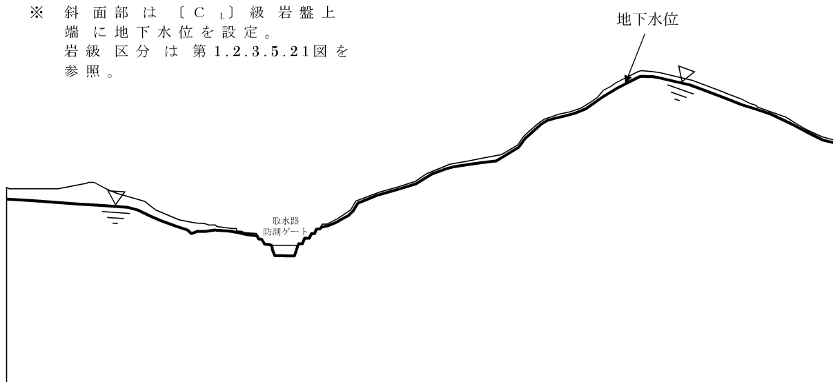
第1.2.3.5.22図 解析用地下水位 (K-K')
