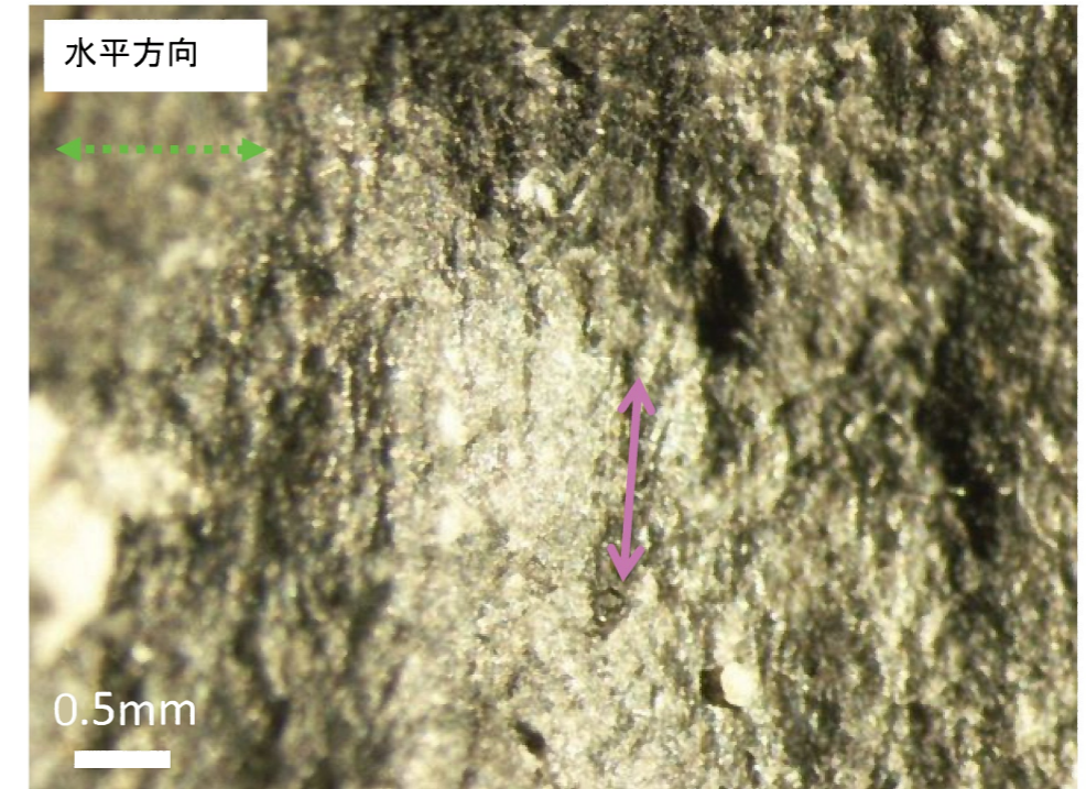
下盤側でみた条線方向 断層面の走向
