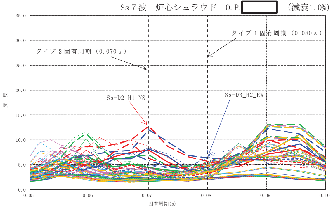
図 2-15 炉心シュラウド支持ロッド固有周期における床応答曲線最大値
