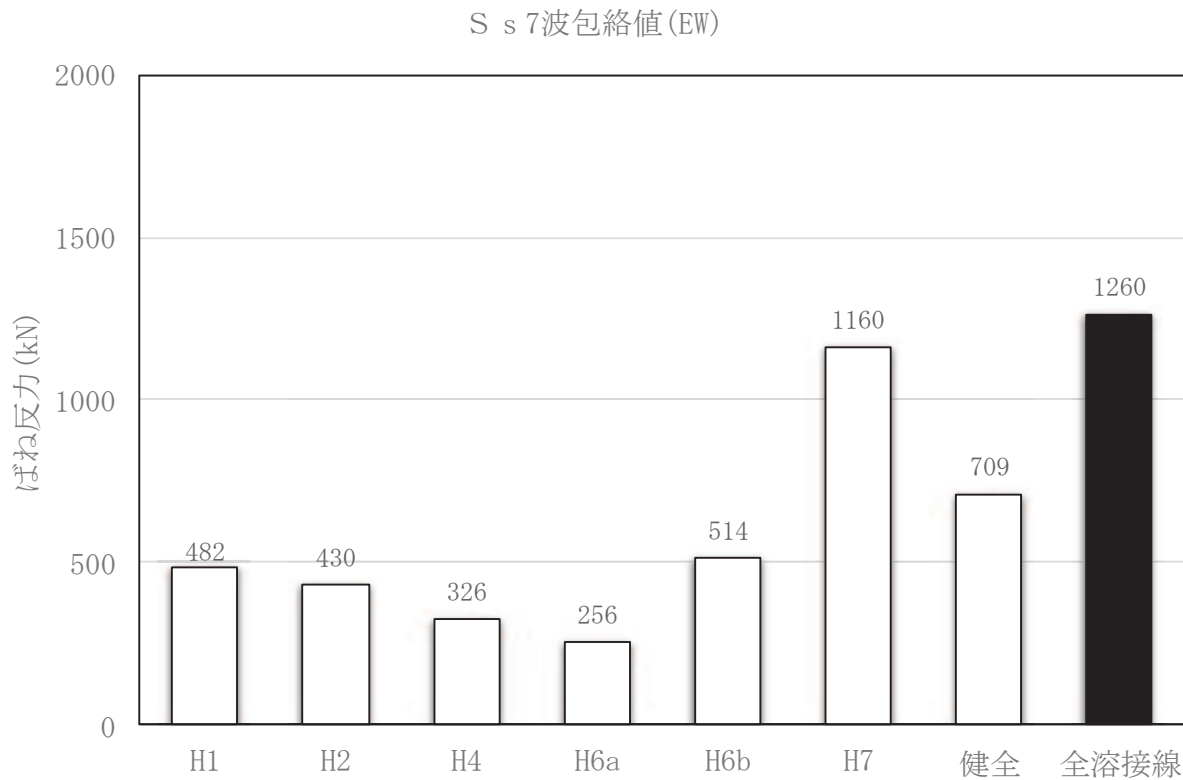
図 2-18 下部スタビライザ反力最大値の比較
