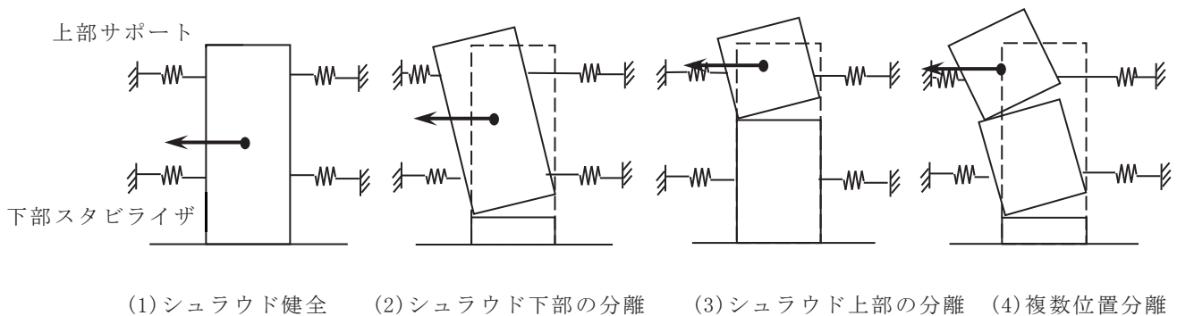
図 2-16 炉心シュラウドの分離想定概念図
