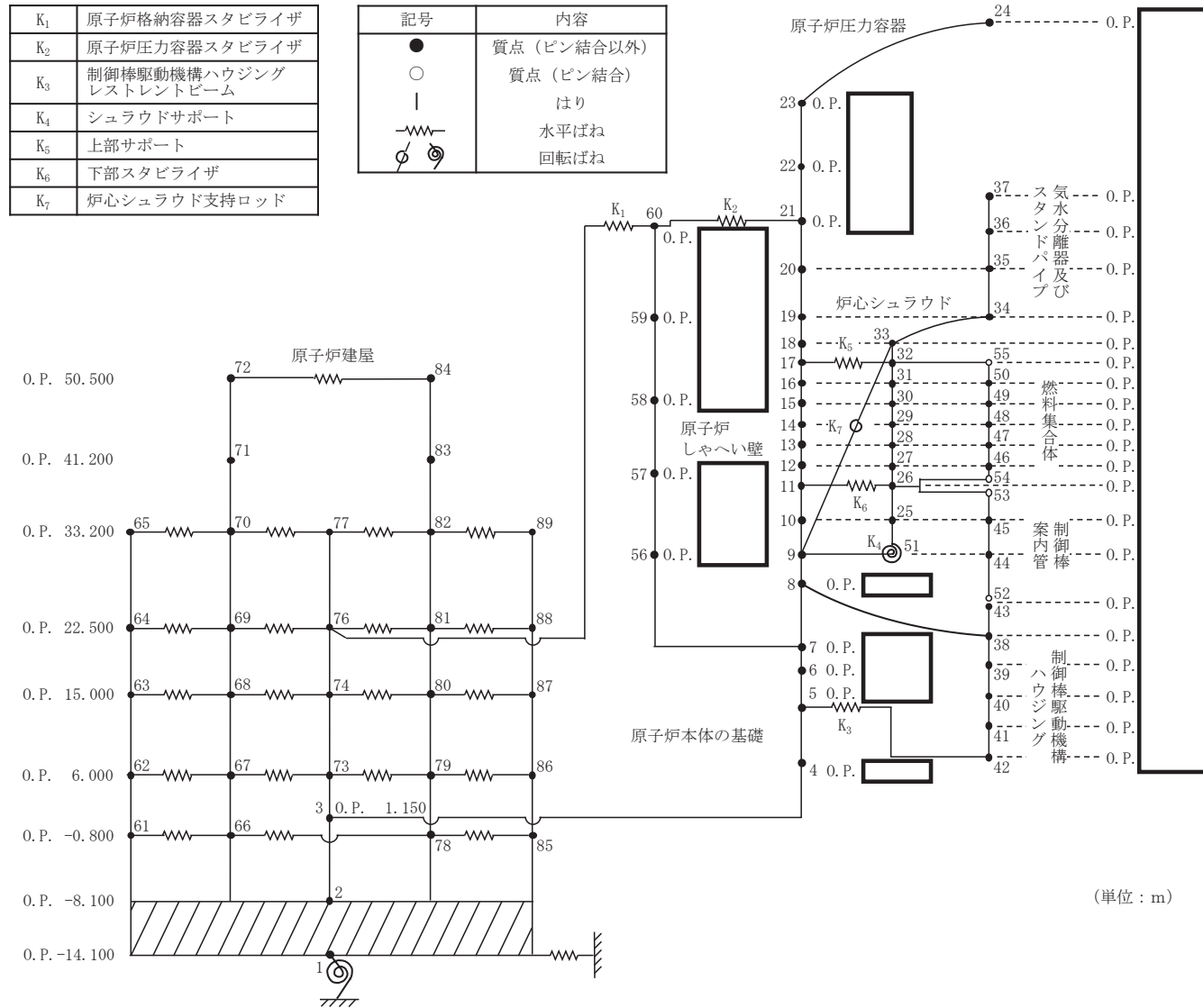
図 1-3 水平方向地震応答解析モデル (炉内構造物系, NS 方向)
