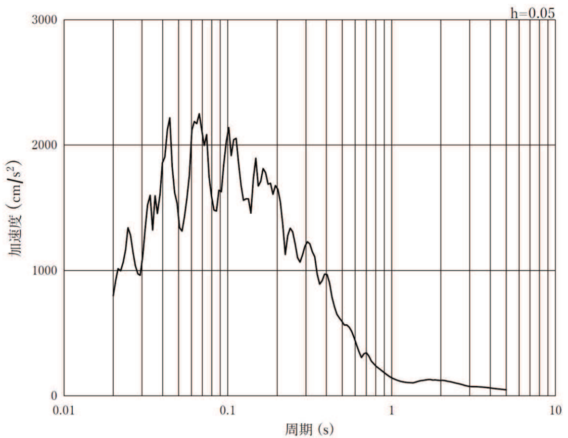
(b)加加速度応答スペクトル
