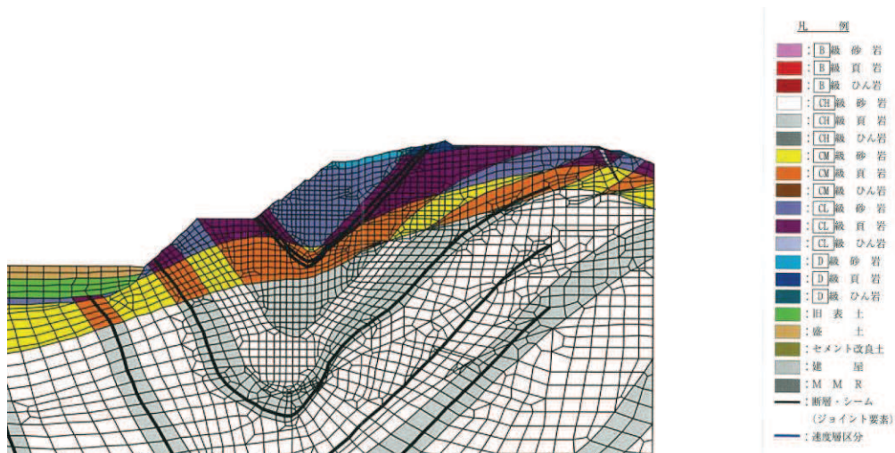
図 5.1-1 地質断面図
