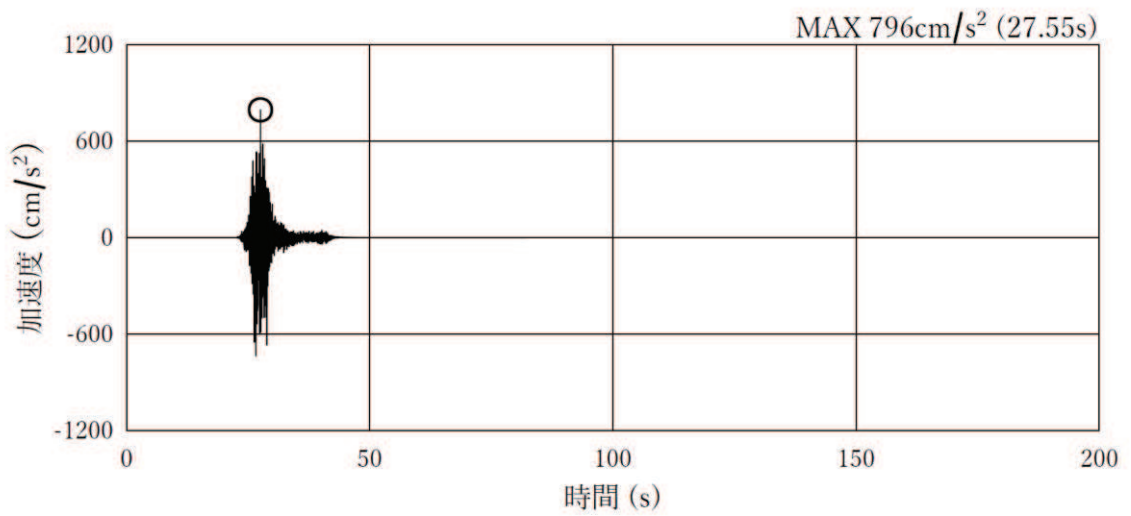
(a)加加速度時刻歴波形
