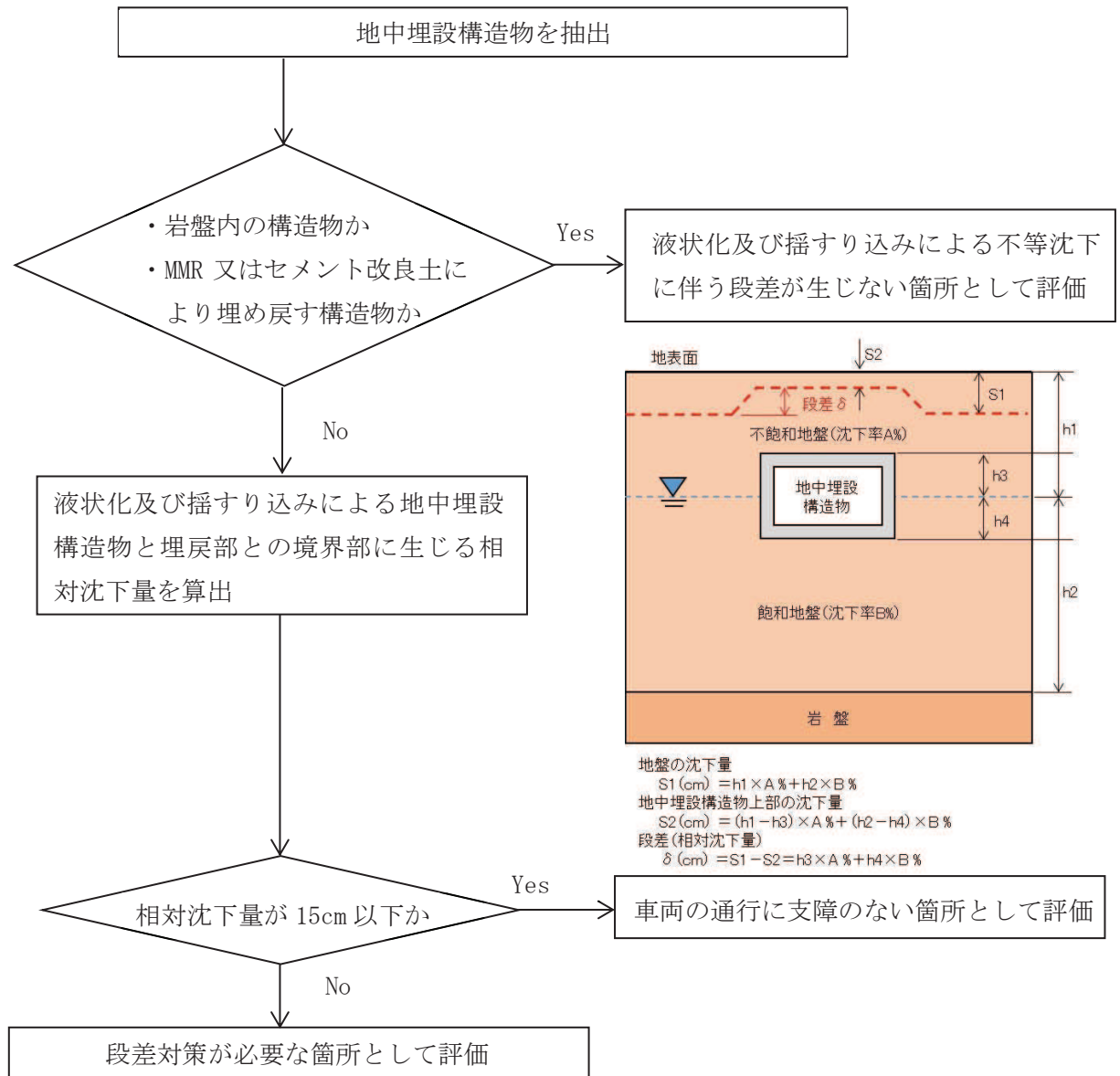
図 3.3.3-2 地中埋設構造物と埋戻部との境界部における不均等沈下に伴う段差評価のフロー
