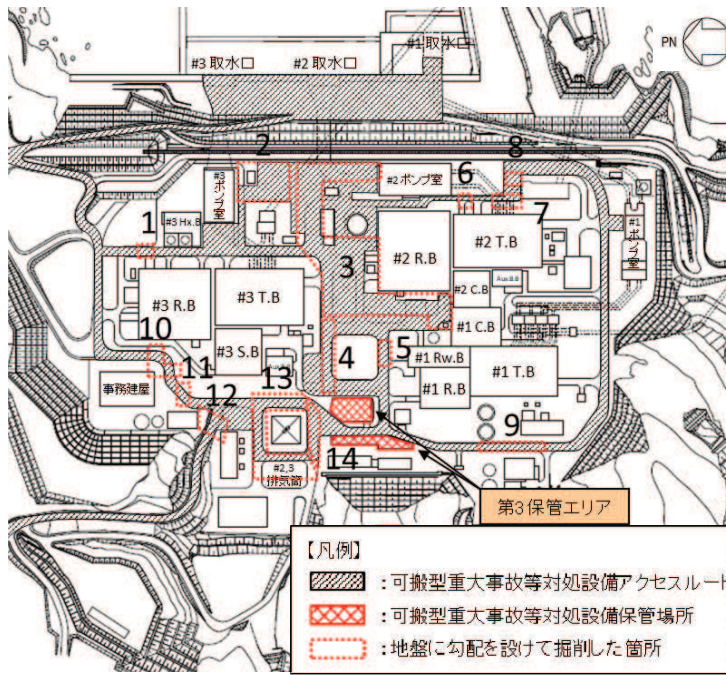
図 3.3.3-10 地山に勾配を設けて掘削した箇所の抽出結果
