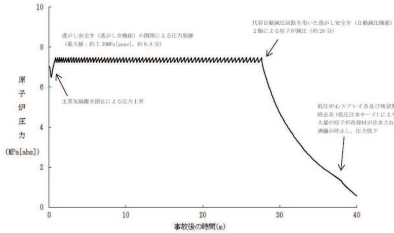
(原子炉圧力の推移)
