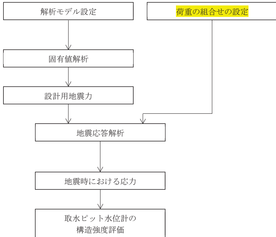
図 2-2 取水ピット水位計の耐震評価フロー
