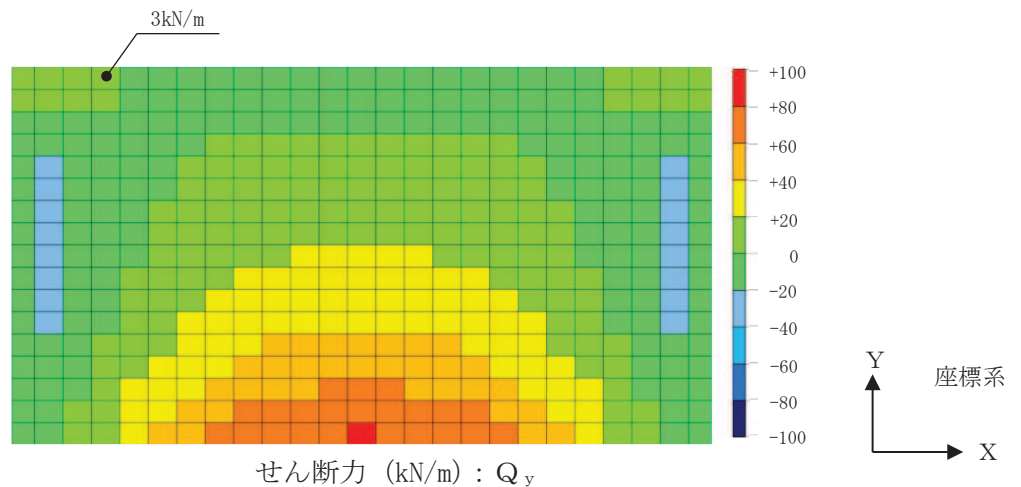
図 3-6 せん断破壊に対する最大照査値ケースの断面力分布図 (解析ケース 1, 隔壁①)
