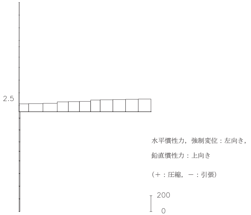
図 4-9(2) 最大照査値を示す解析ケースにおける断面力図 (軸力 (kN)) (解析ケース 4, トレンチ②)
