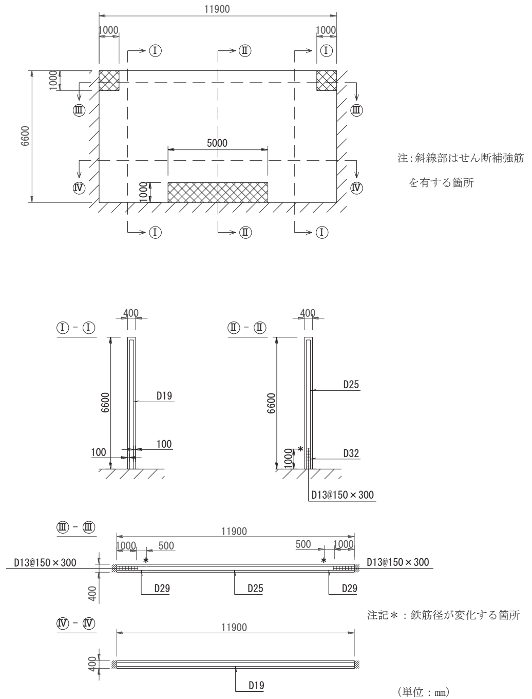
図 3-1(1) 概略配筋図 (隔壁①)
