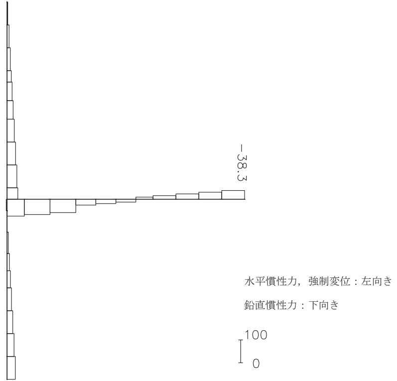
図 4-10(3) 最大照査値を示す解析ケースにおける断面力図 (せん断力 (kN)) (地震時, 解析ケース 3, トレンチ②)
