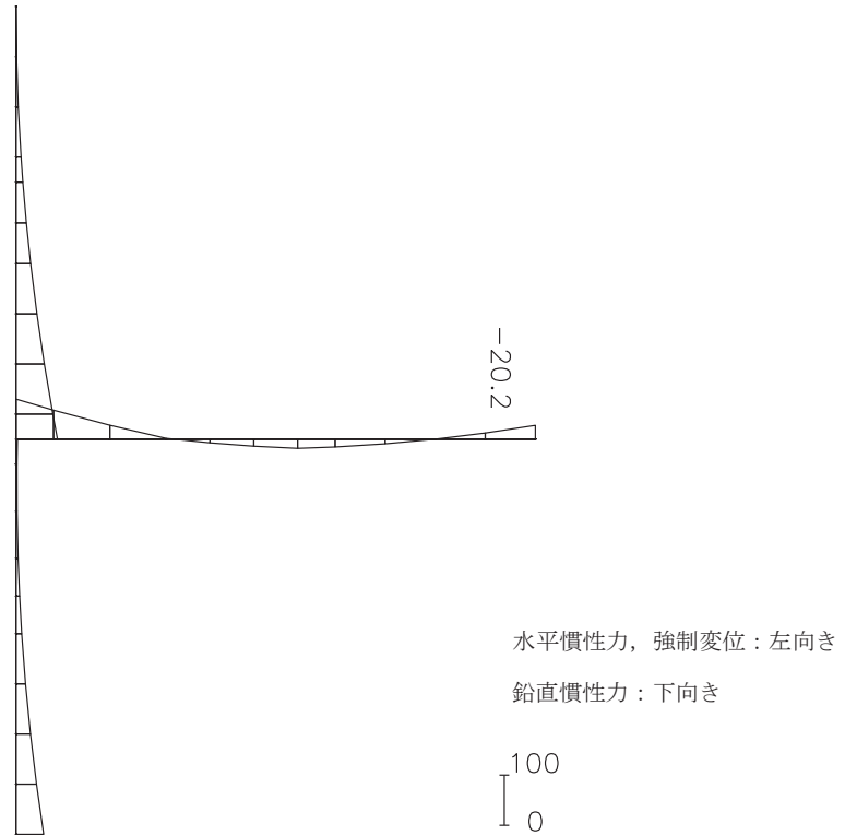
図 4-10(1) 最大照査値を示す解析ケースにおける断面力図（曲げモーメント (kN・m)） （地震時，解析ケース 3，トレンチ②）
