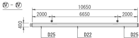
図 3-1(4) 概略配筋図 (隔壁④)
