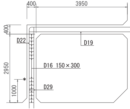
図 4-1(1) 概略配筋図 (トレンチ①)
