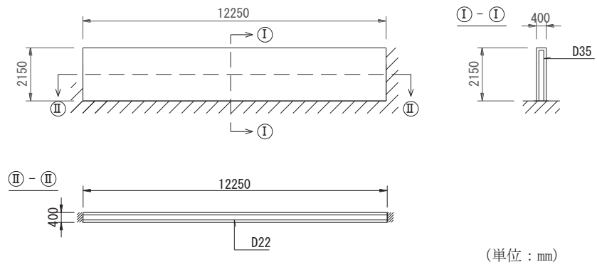
图3-1(6) 概略配筋图 (隔壁⑥)
