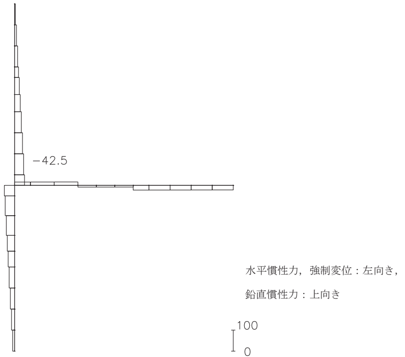
図 4-9(3) 最大照査値を示す解析ケースにおける断面力図 (せん断力 (kN)) (解析ケース 4, トレンチ②)
