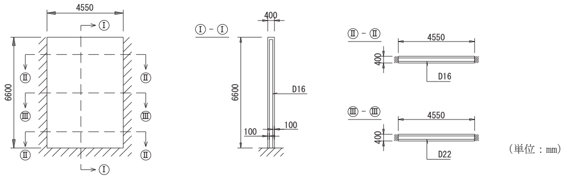
图 3-1(5) 概略配筋图 (隔壁⑤)
