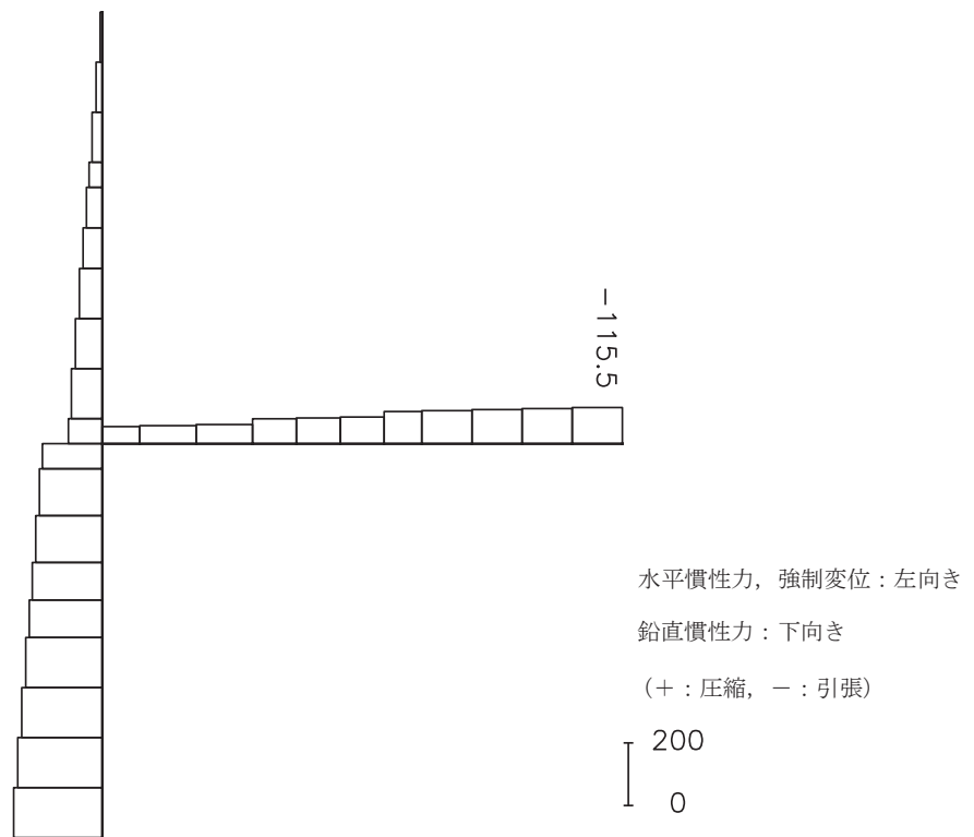
図 4-10(2) 最大照査値を示す解析ケースにおける断面力図（軸力 (kN)） （地震時，解析ケース 3，トレンチ②）
