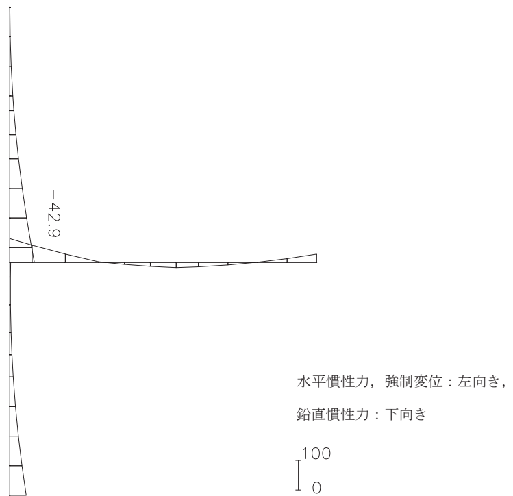
図 4-14(1) 最大照査値を示す解析ケースにおける断面力図 (曲げモーメント (kN・m)) (解析ケース 3, トレンチ②)
