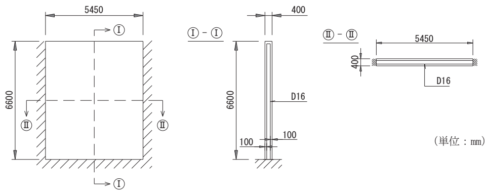
図 3-1(3) 概略配筋図 (隔壁③)
