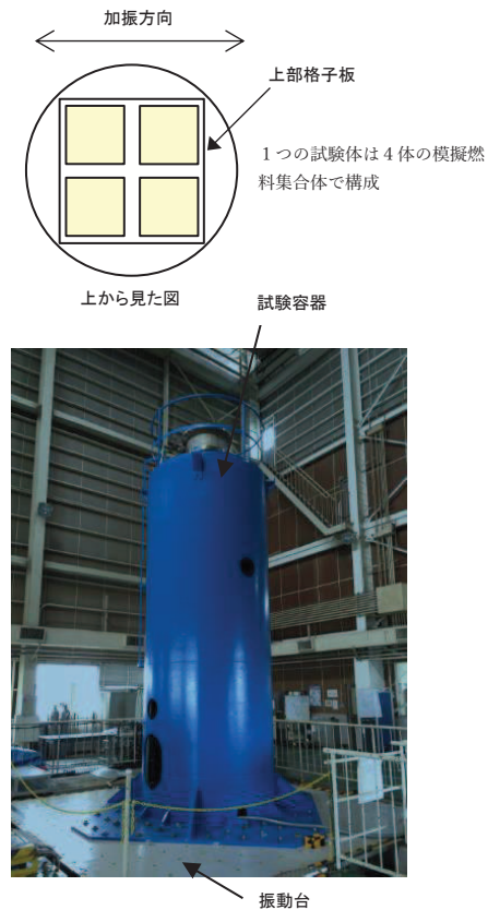
図 12-2 試験装置外観
