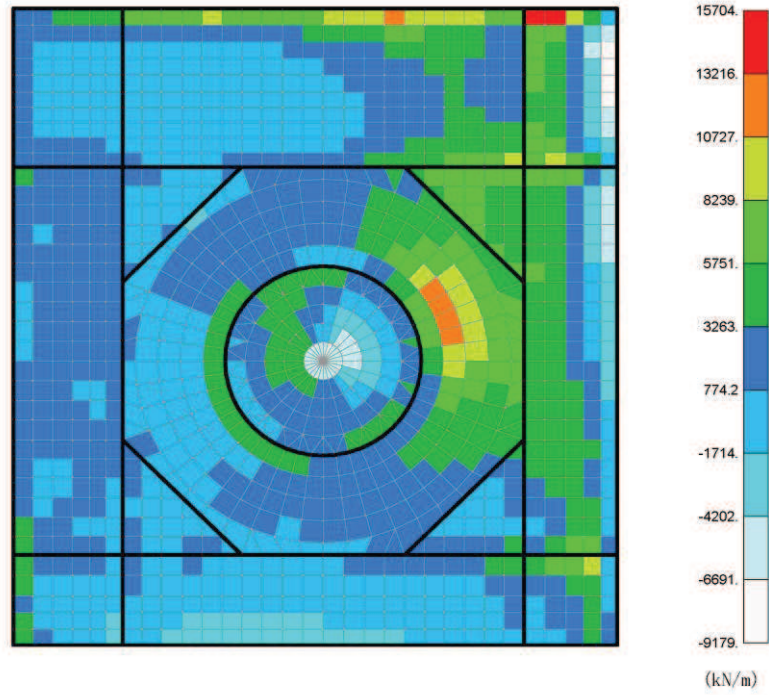
組合せケース 3-9 (放射方向, NS 方向)
