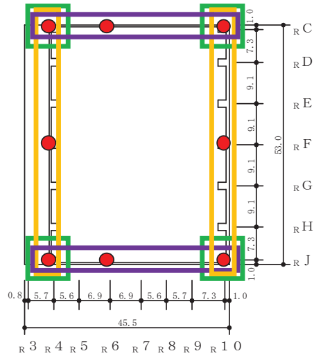
図 3-14(3) 代表節点の位置と応答平均化範囲 (O. P. 41. 2m)
