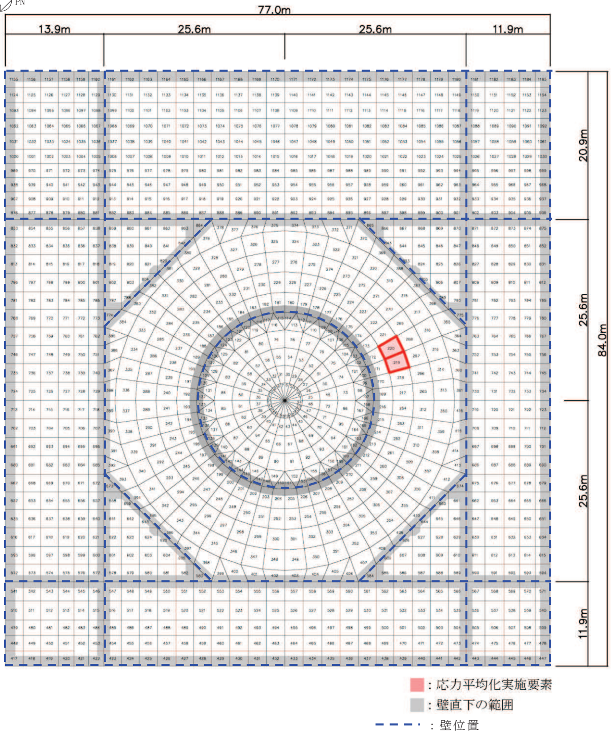
図 2-1 要素位置図
