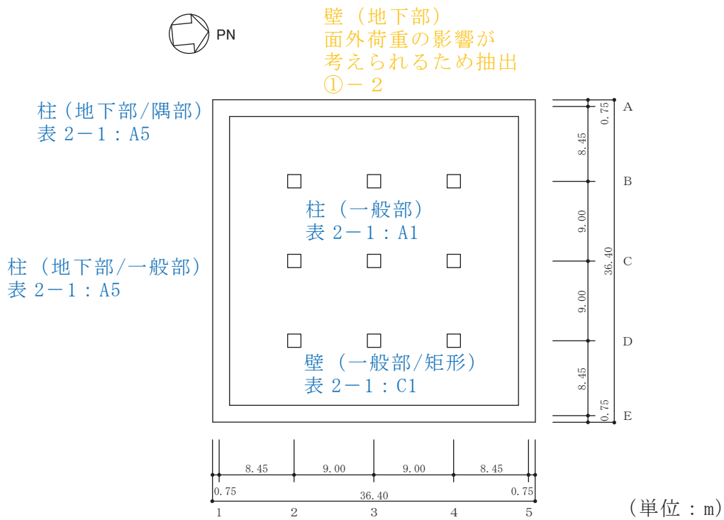
図 2-6-1(2) 緊急時対策建屋の概略平面図 (O. P. 57. 3m)
