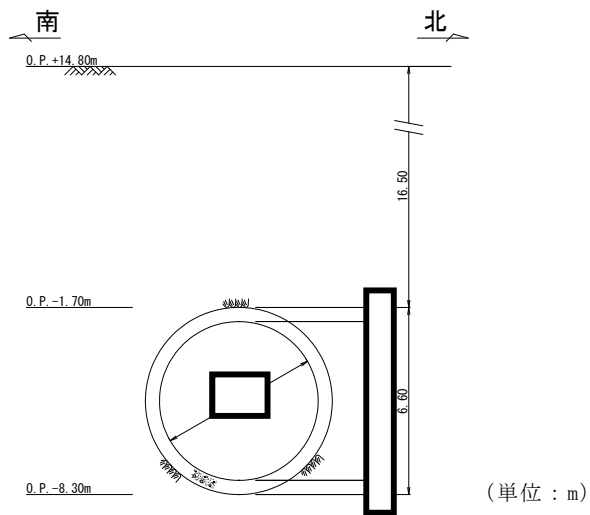
図 3-3-13 排気筒連絡ダクト断面図 (B-B 断面, 岩盤部)
