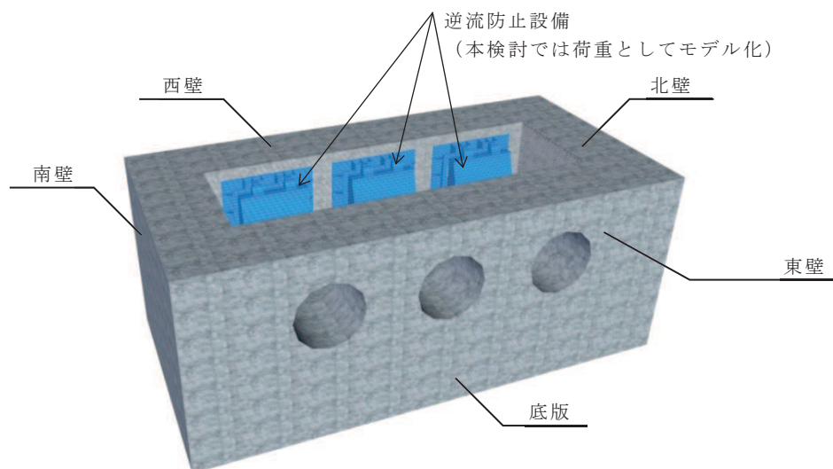
図 3-4-11 屋外排水路逆流防止設備（防潮堤南側）出口側集水ピット 構造概要図
