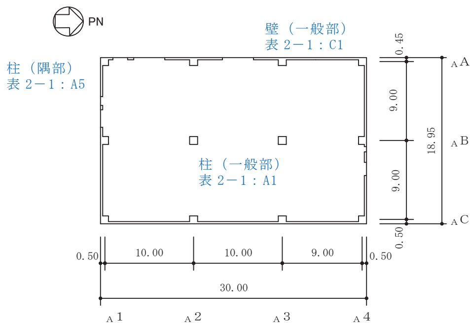
図 2-8-1(2) 補助ボイラー建屋の概略平面図 (0. P. 15. 0m)
