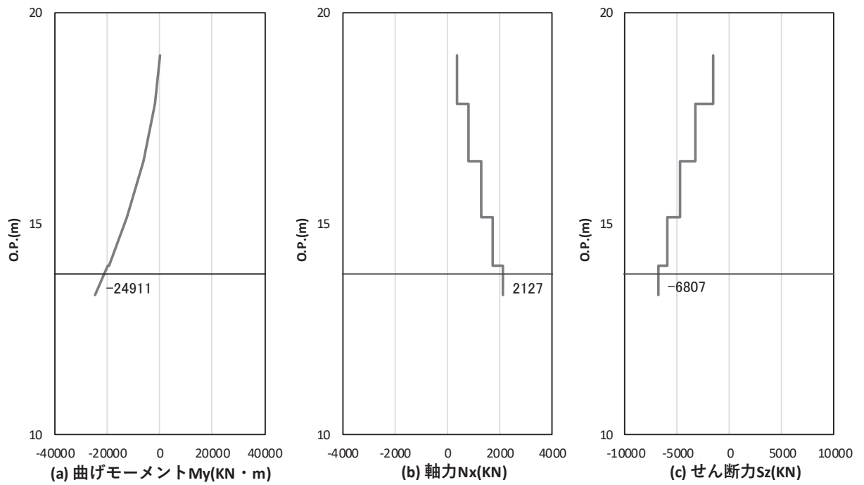
図 3-4-43 (1) 水平 2 方向及び鉛直方向地震力の組合せにおける RC 支柱の曲げ・軸力系の破壊に対する照査における照査時刻での断面力 (鋼桁 1 : 基礎 2, 主方向 (桁軸方向), t = 6.89\text{s} )
