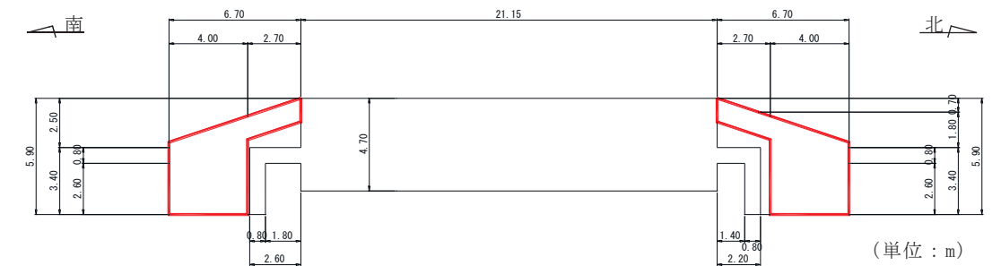
図 3-3-34 原子炉機器冷却海水配管ダクト (鉛直部) 水平断面図 (断面⑤)
