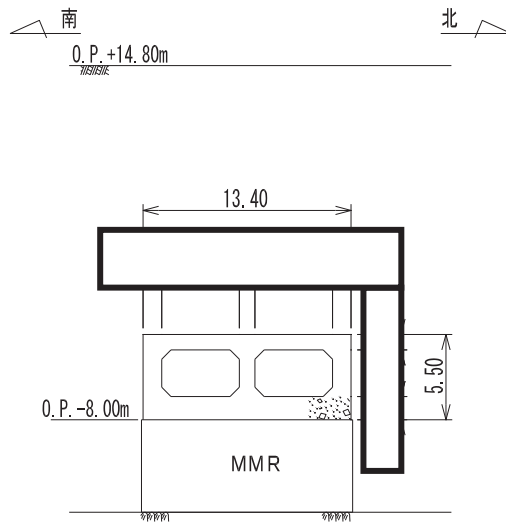
図 3-3-37 取水路（標準部）断面図（A-A 断面）
