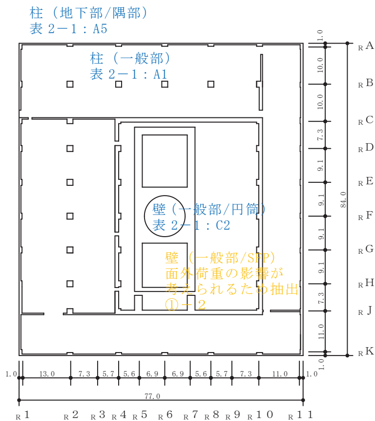
図 2-1-1(5) 原子炉建屋の概略平面図 (O.P. 22.5m)
