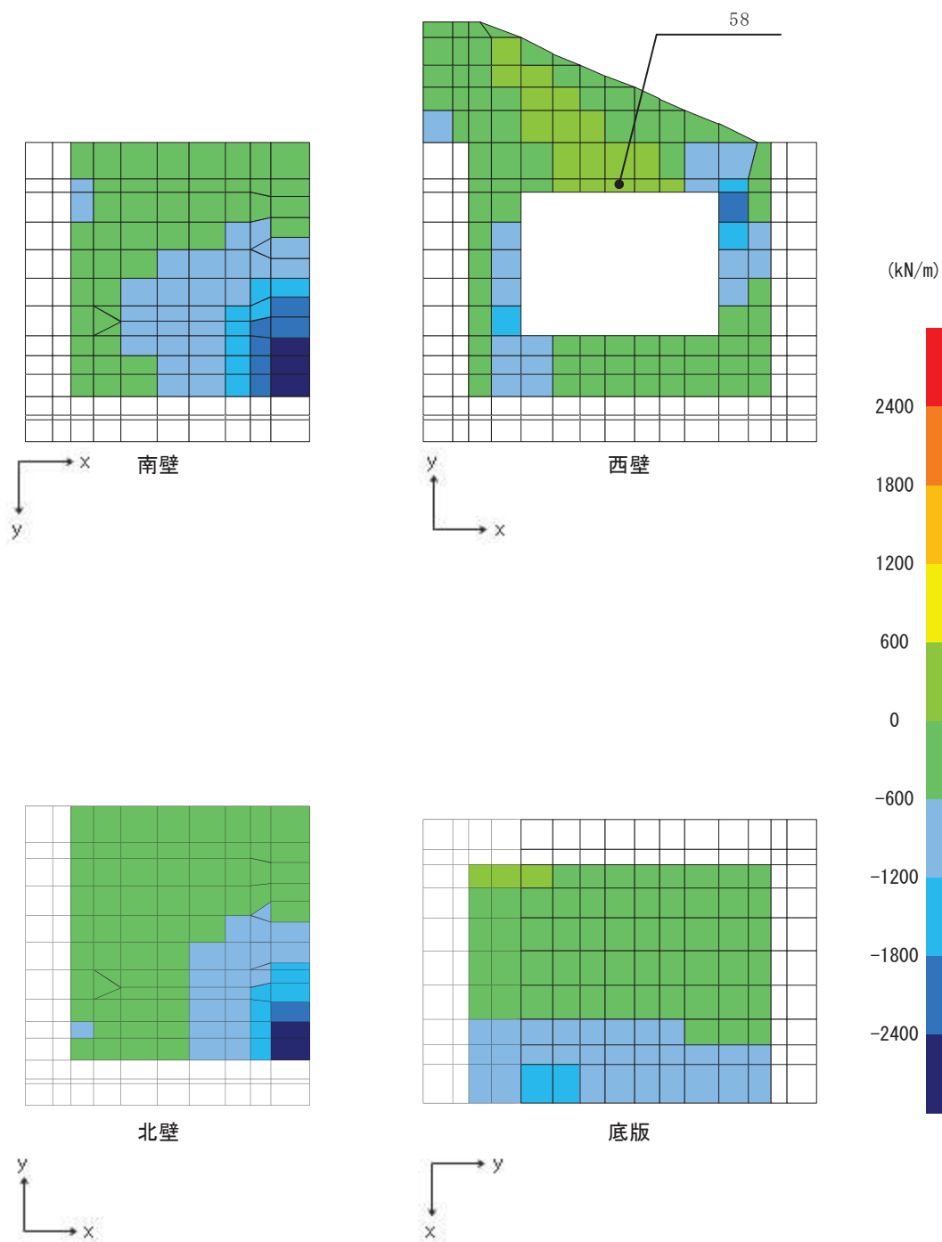
図3-4-34 水平2方向及び鉛直方向地震力の組合せによる 曲げ・軸力系の破壊に対する照査時の断面力分布図 (軸力 (kN/m) : N_y ) (解析ケース③, S_s - D2 (-+))
