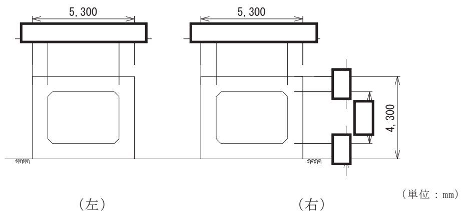
図 3-3-21 第 1 号機取水路の構造図 (B-B 断面)
