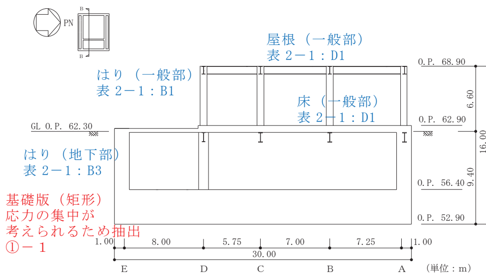
図 2-5-1 (2) 緊急用電気品建屋の概略断面図 (B-B 断面, EW 方向)
