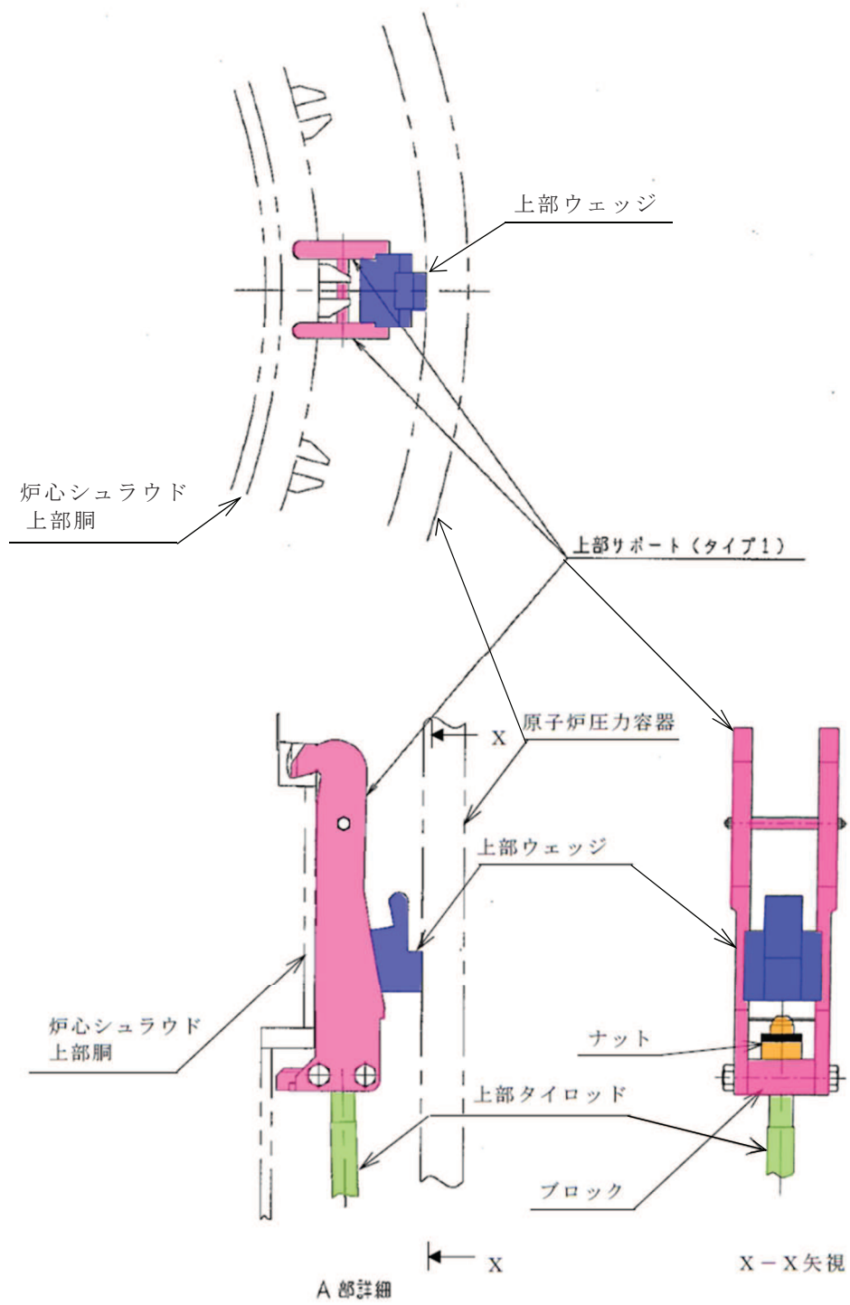
図 1(2) 炉心シュラウド支持ロッドの構造
