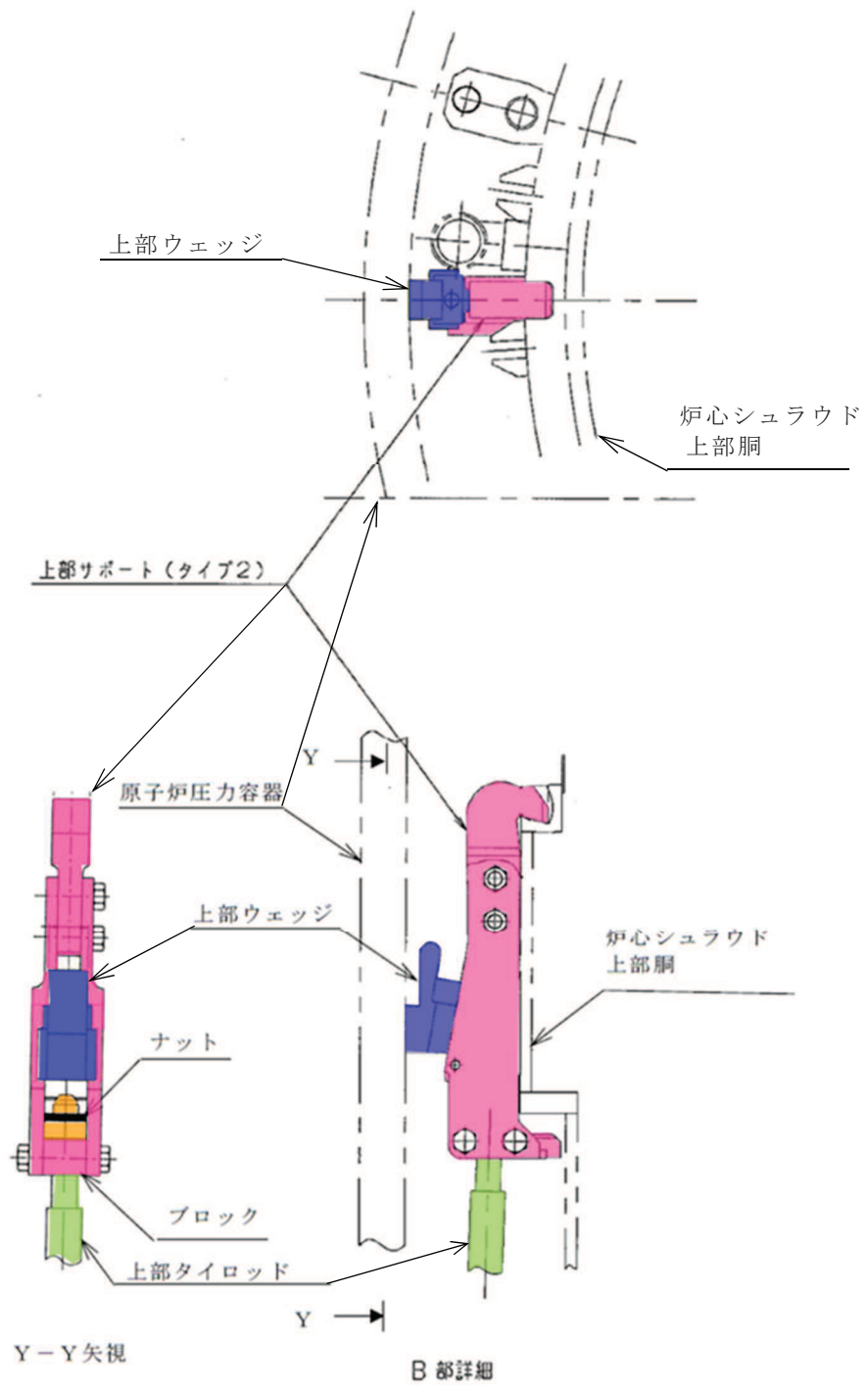
図 1(3) 炉心シュラウド支持ロッドの構造
