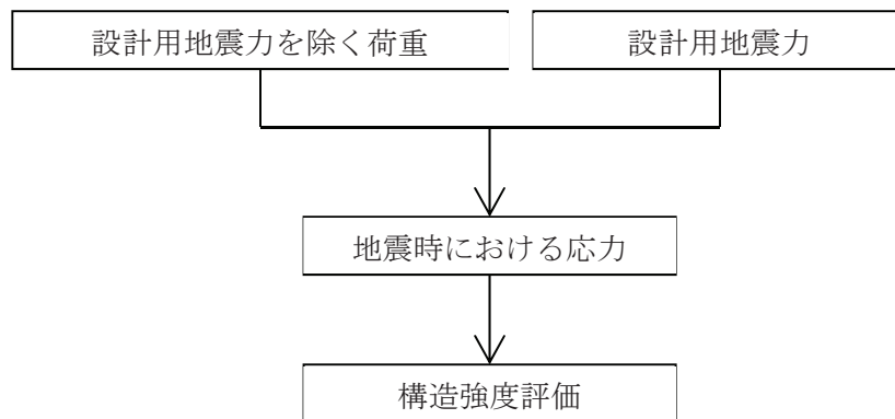
図2-1 原子炉压力容器の耐震評価フロー
