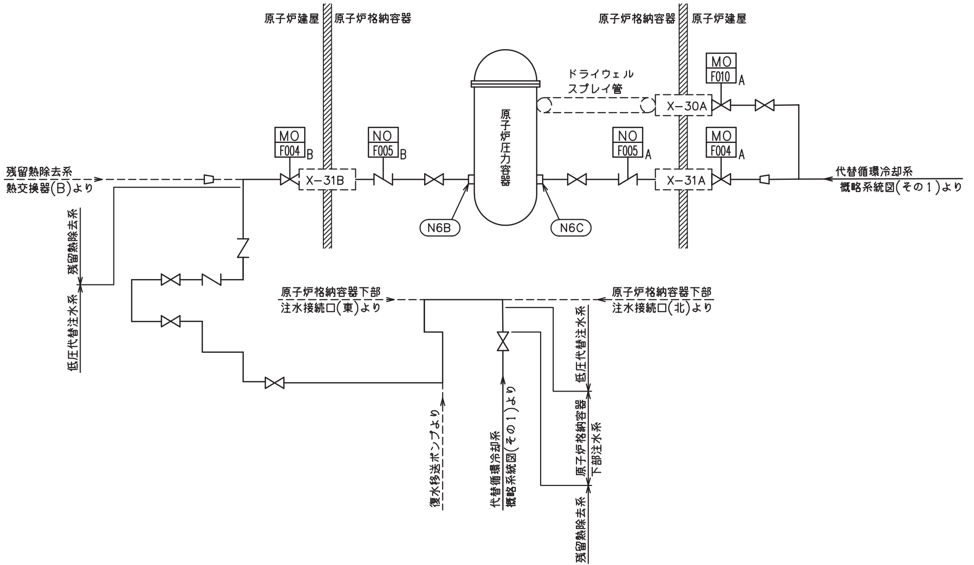
代替循環冷却系概略系統図(その2)
