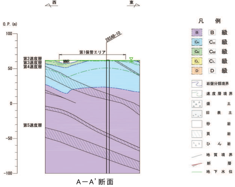
図 2.3.3-2 第1保管エリアの地質断面図
