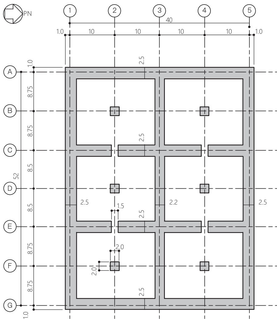
図 1-7 耐震壁の剛性評価範囲 (UD 方向)
