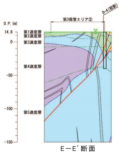
図 2.3.3-4 第3保管エリアの地質断面図
