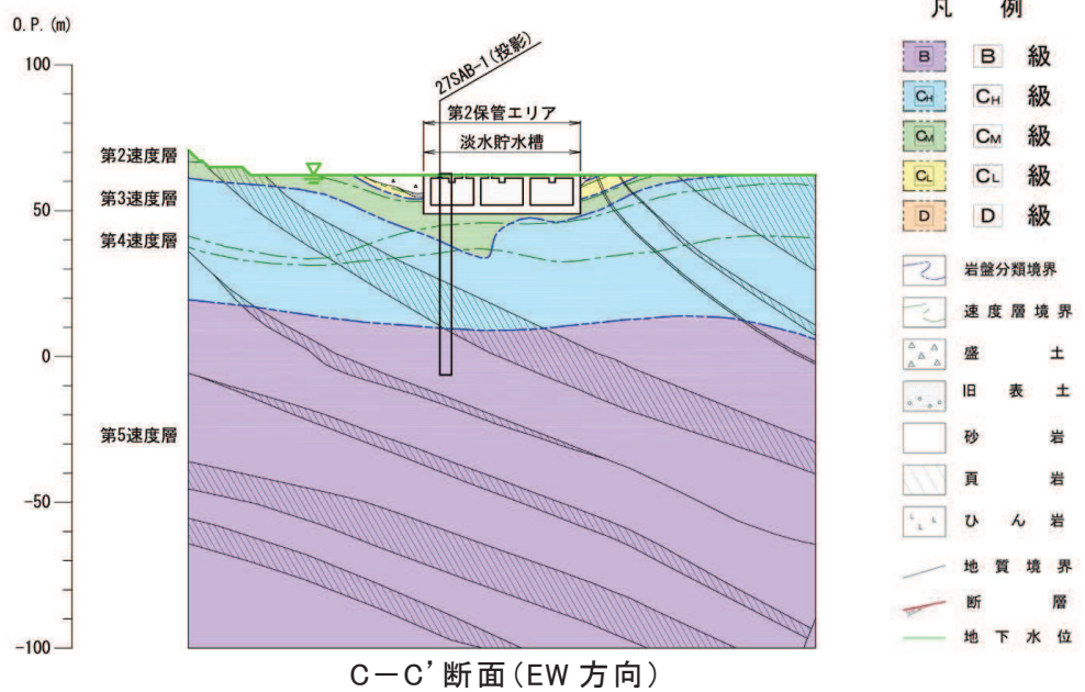
図 2.3.3-3 第 2 保管エリアの地質断面図
