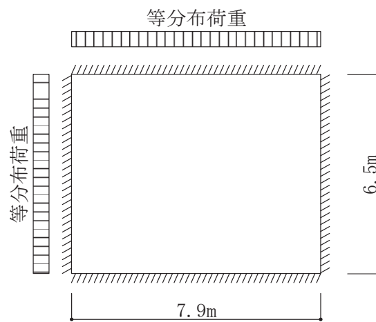
図 1-13 頂版の解析モデル
