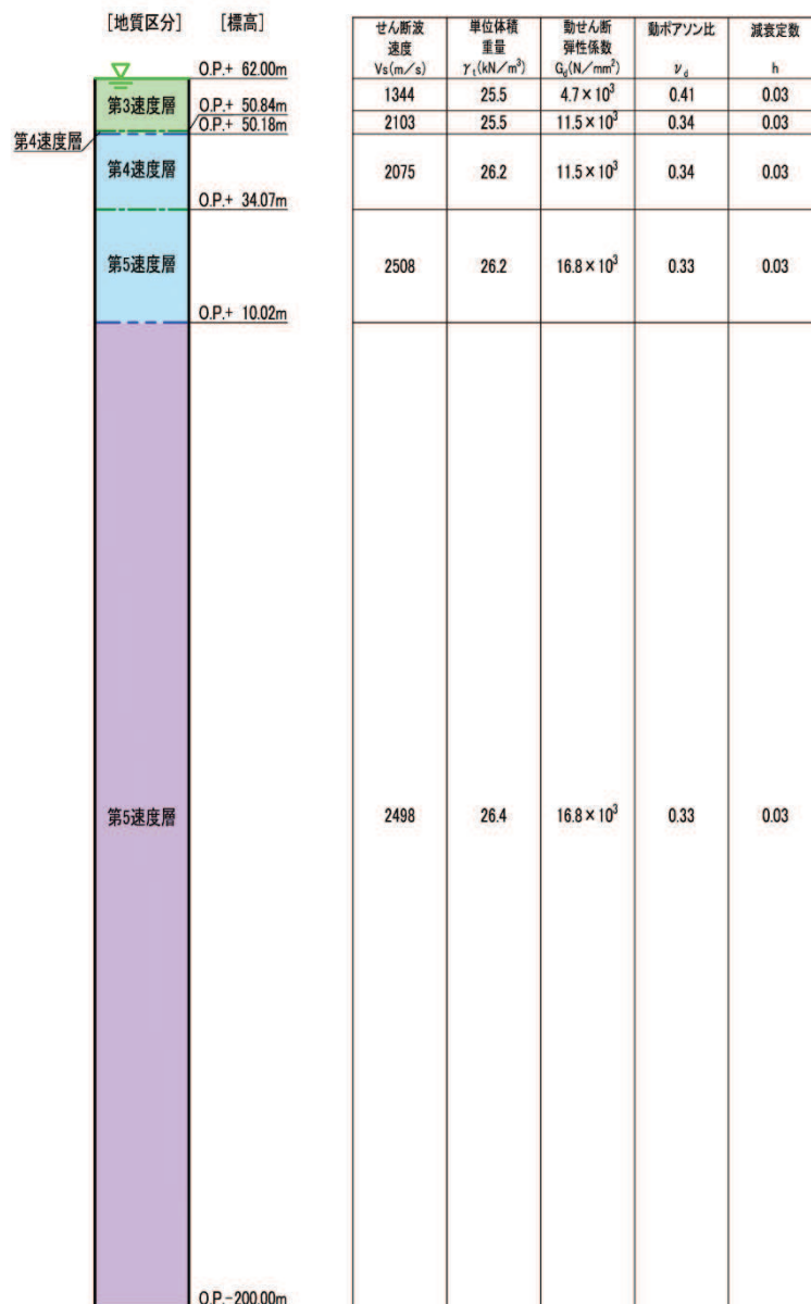
図 2.3.3-11(2) 第4保管エリア②の地震応答解析モデル(一次元)
