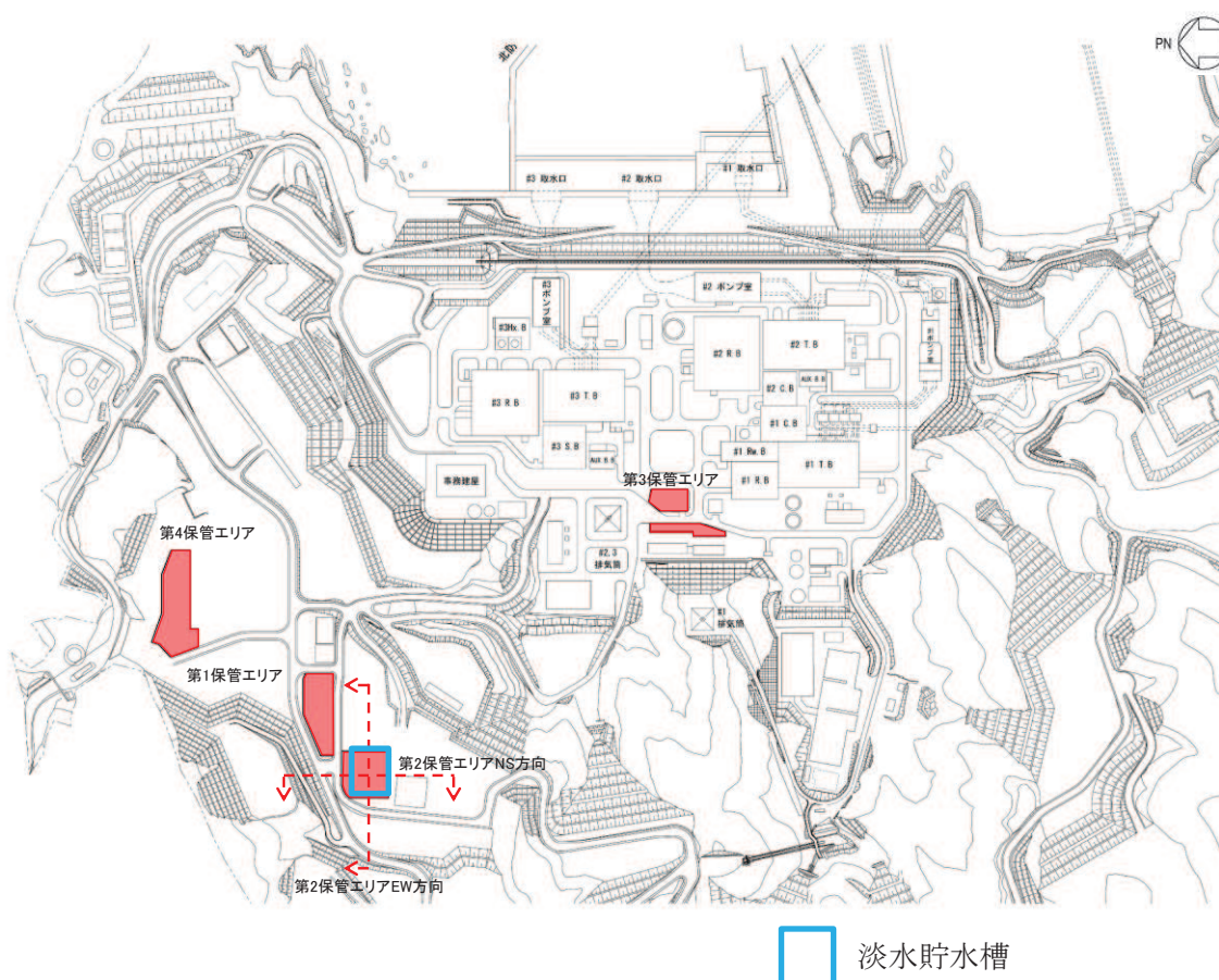
図 1-1 淡水貯水槽の設置位置
