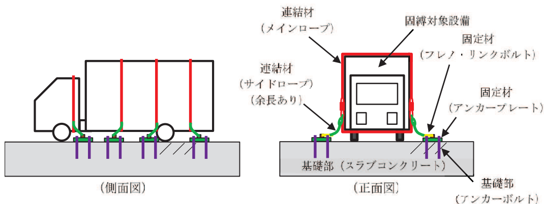
図3-1 固縛装置の構造概要
