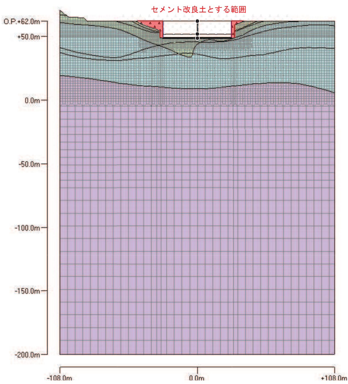
図 2-1(2) 第 2 保管エリアの地震応答解析モデル (二次元)
