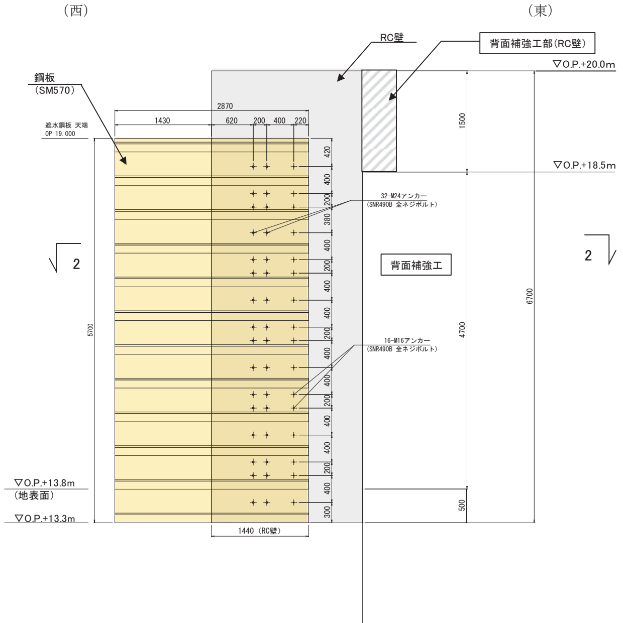
(正面図 : 1-1 断面)
