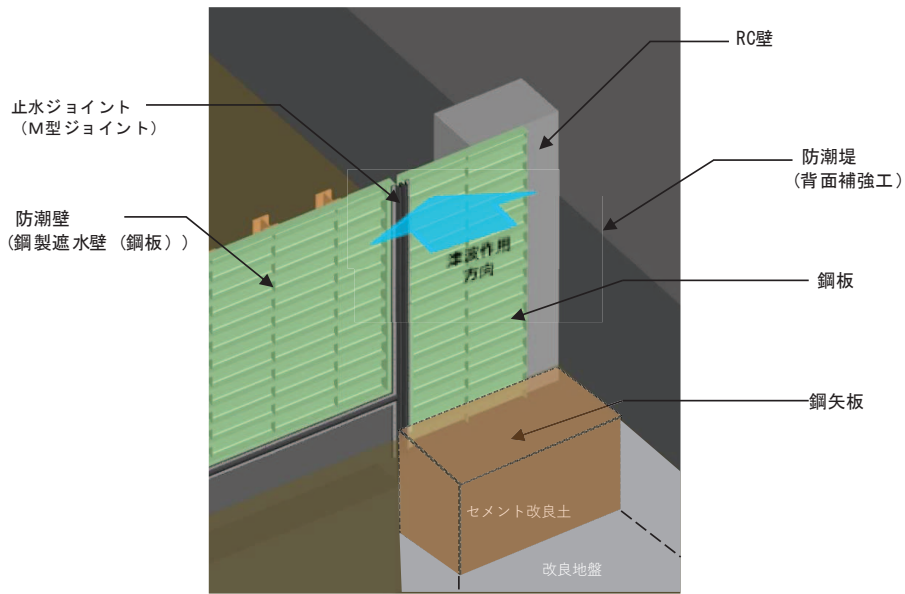
図 1-2(1) 防潮堤取り合い部の構造概要 (取合い部①)
