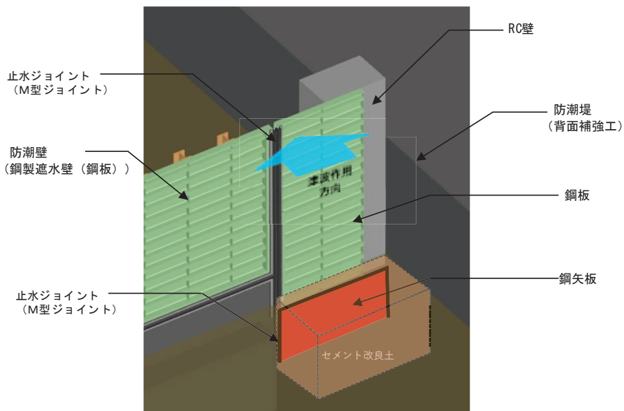
図 1-2(2) 防潮堤取り合い部の構造概要 (取合い部②・③・④)
