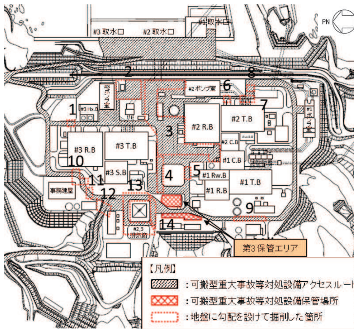
図 8.1-9 地山に勾配を設けて掘削した箇所の抽出結果
