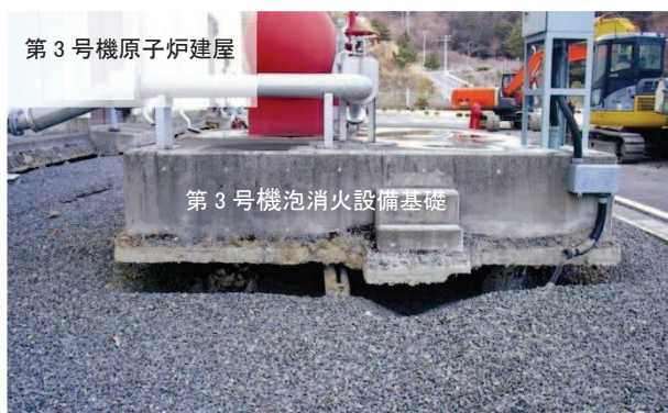
写真⑥ 沈下発生状況
