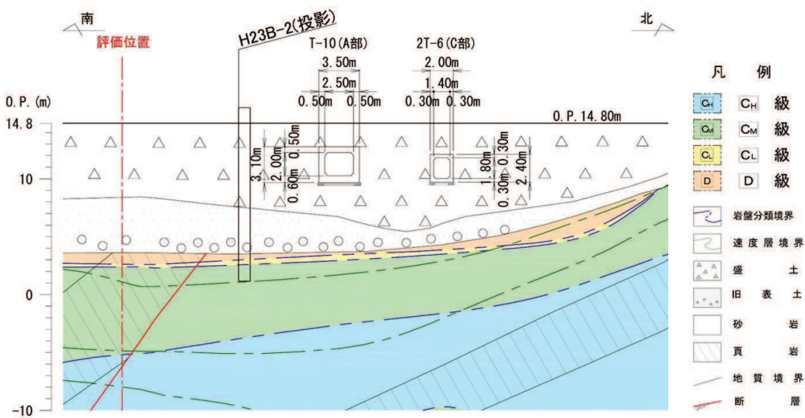
図 8.3-10 地質断面図 (C-C' 断面)
