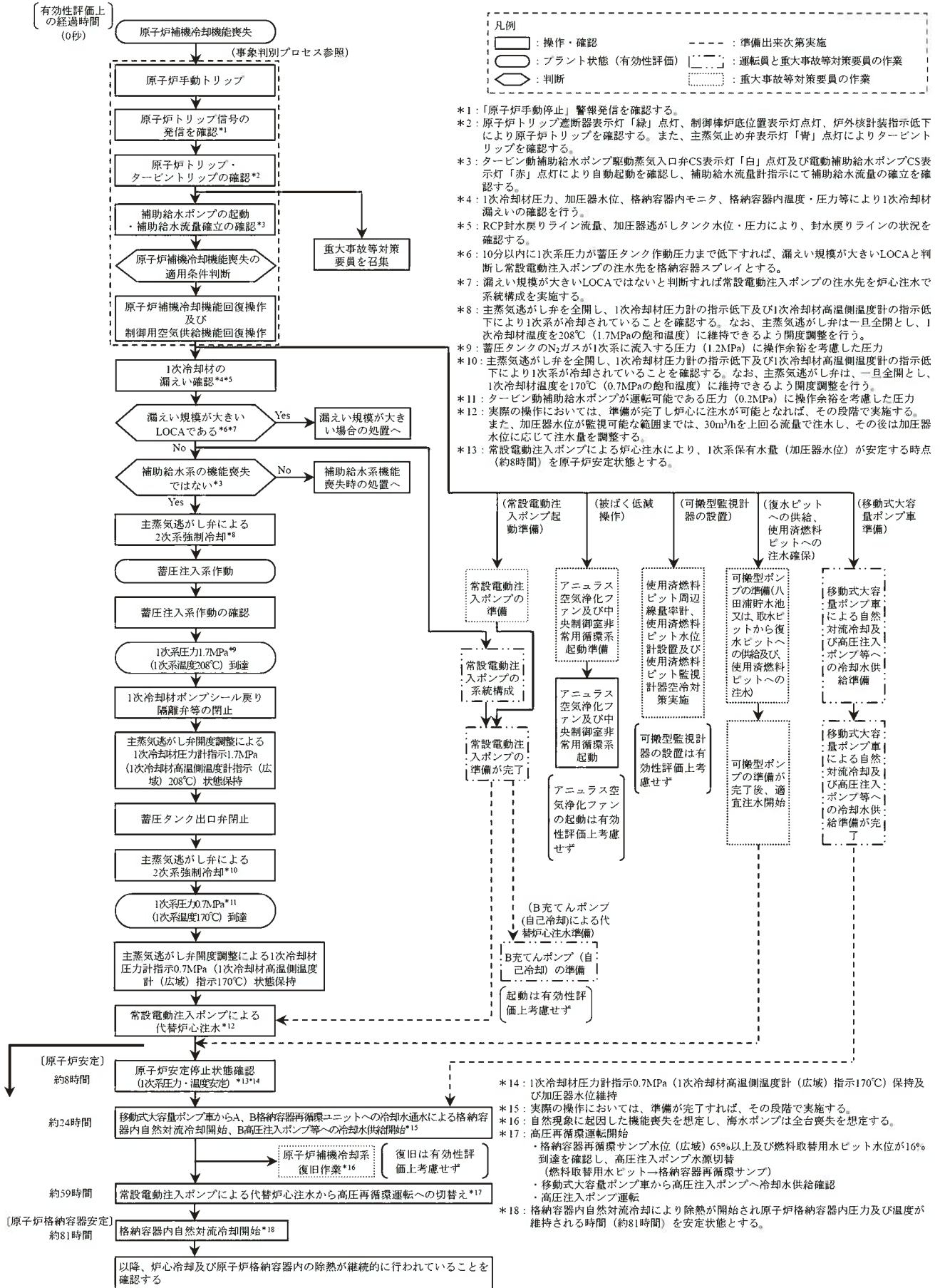
第1.15-19図 「原子炉補機冷却機能喪失」の対応手順の概要
