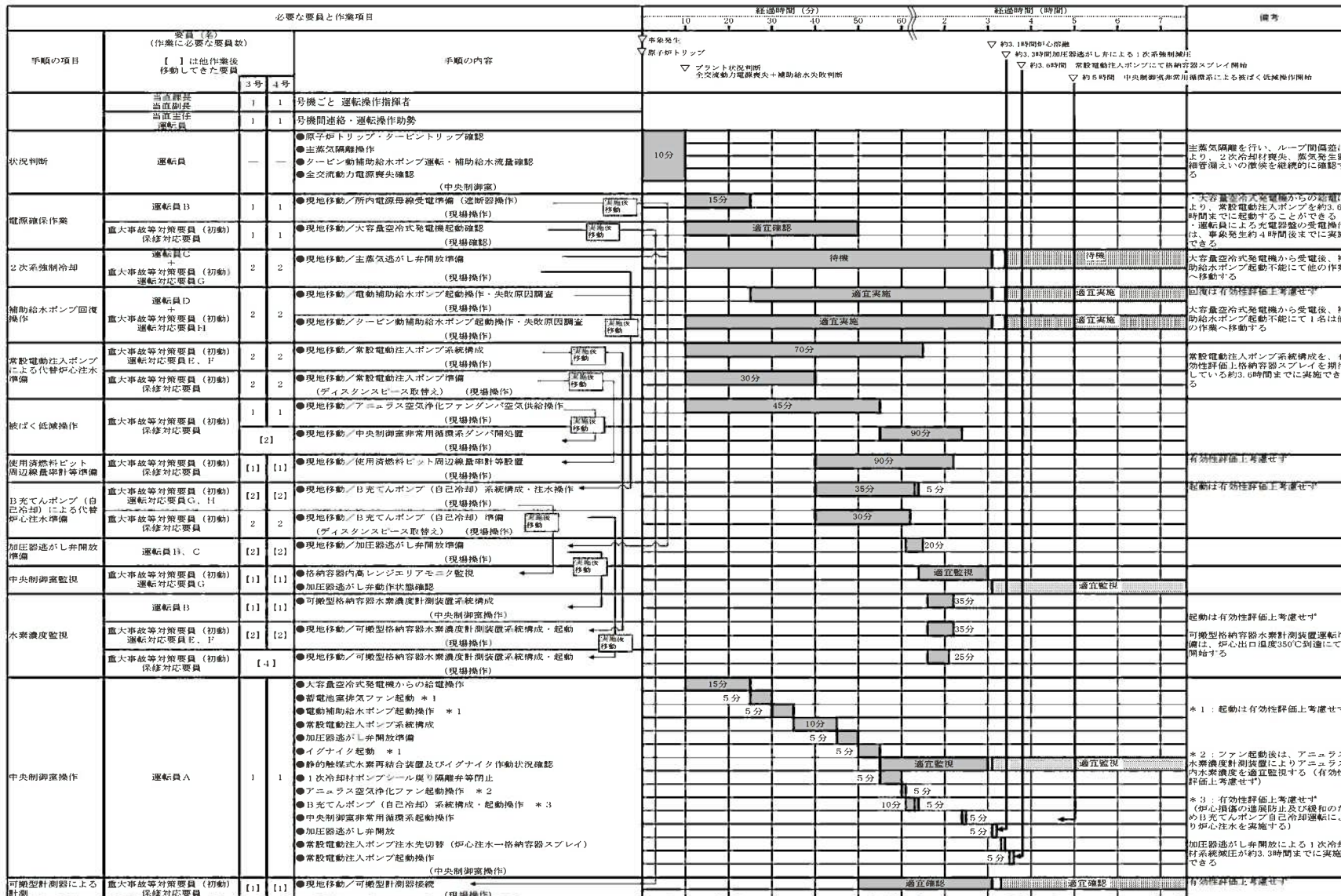
第1.15-53図 「雰囲気圧力・温度による静的負荷(格納容器過温破損)」の作業と所要時間(1/2) (外部電源喪失時に非常用所内交流動力電源が喪失し、補助給水機能が喪失する事故)
