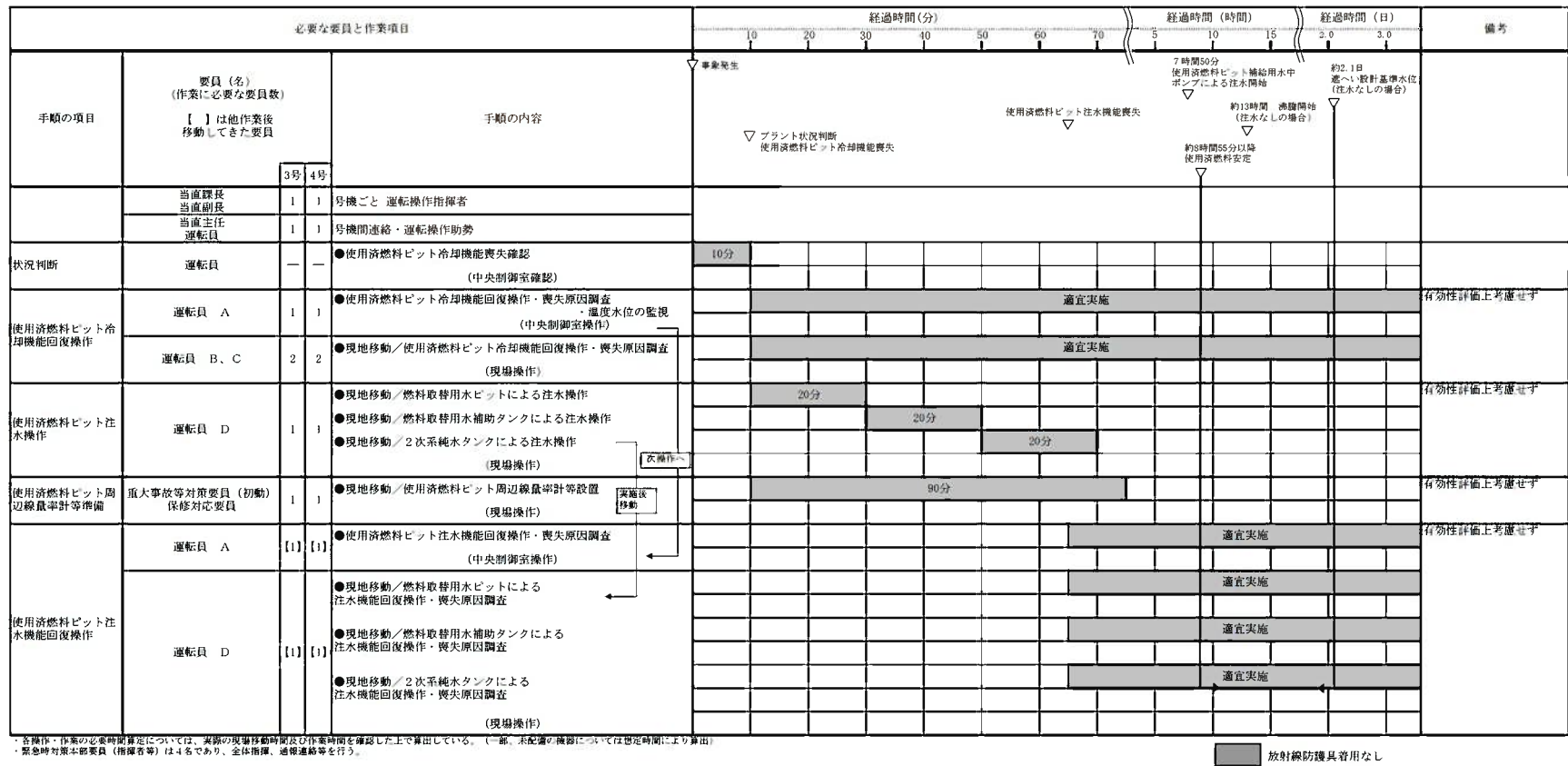
第1.15-59図 「想定事故1」の作業と所要時間(1/2)
