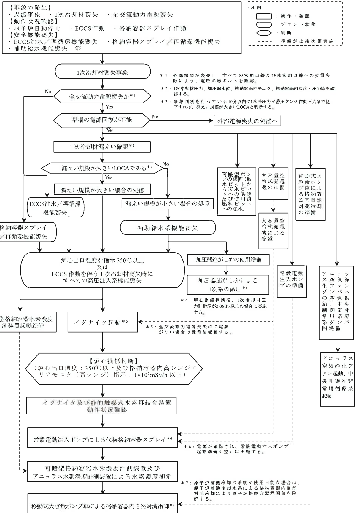
第1.15-49図 「雰囲気圧力・温度による静的負荷(格納容器過圧破損)」の対応手順の概要(格納容器破損モード)
