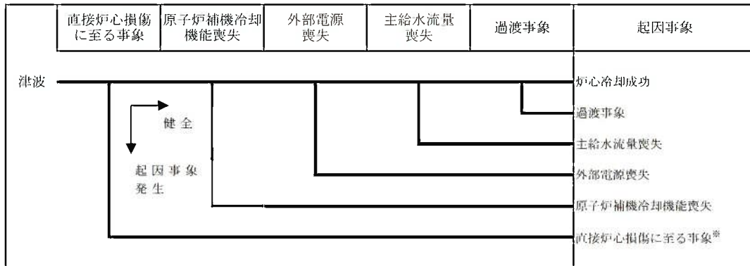
第1.15-2図 地震PRA階層イベントツリー
