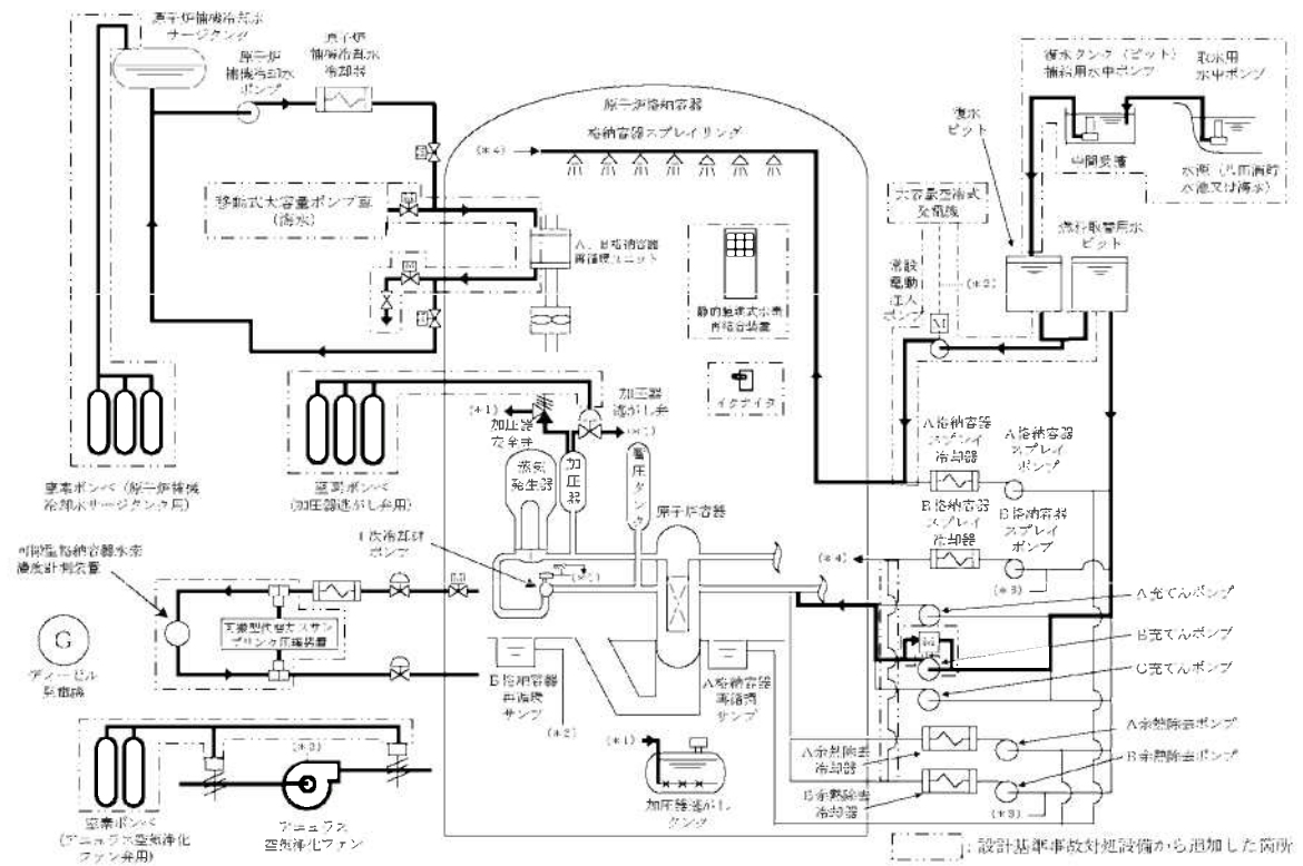
第1.15-54図 「水素燃焼」の重大事故等対策の概略系統図
