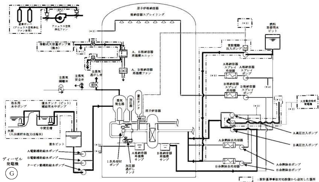
第1.15-10図 「全交流動力電源喪失」の重大事故等対策の概略系統図
