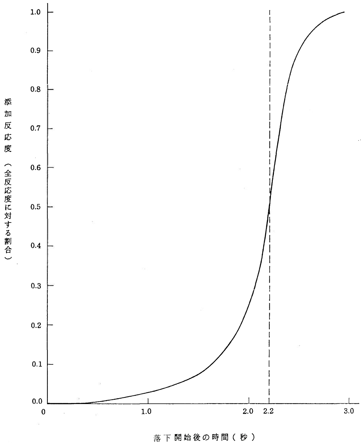
第1.15-79図 トリップ時の制御棒クラスタ落下による反応度添加曲線
