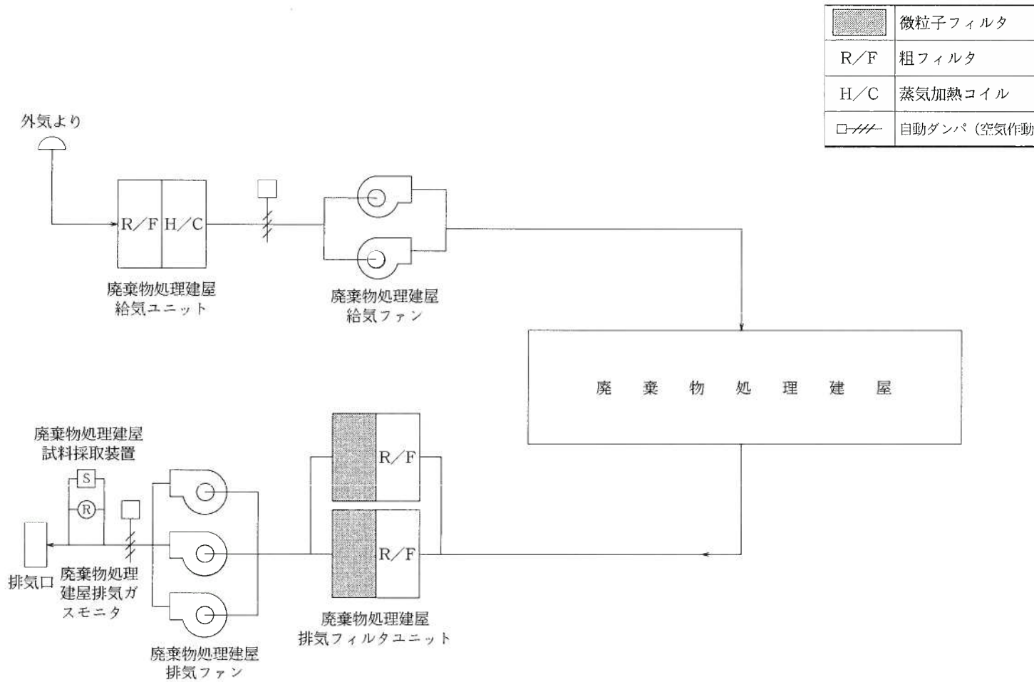
第1.12-26図 廃棄物処理建屋空調装置説明図(3、4号機共用)
