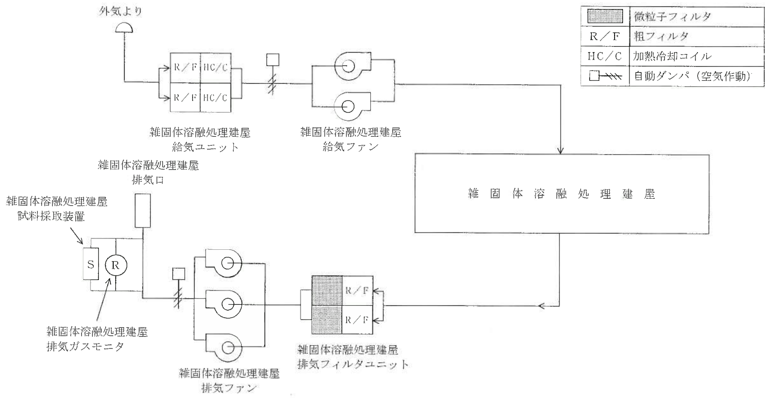
第1.12-27図 雑固体溶融処理建屋空調装置説明図
