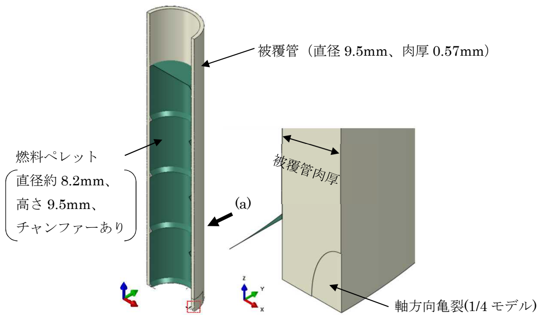
図1 既存のPCMI解析用モデル
