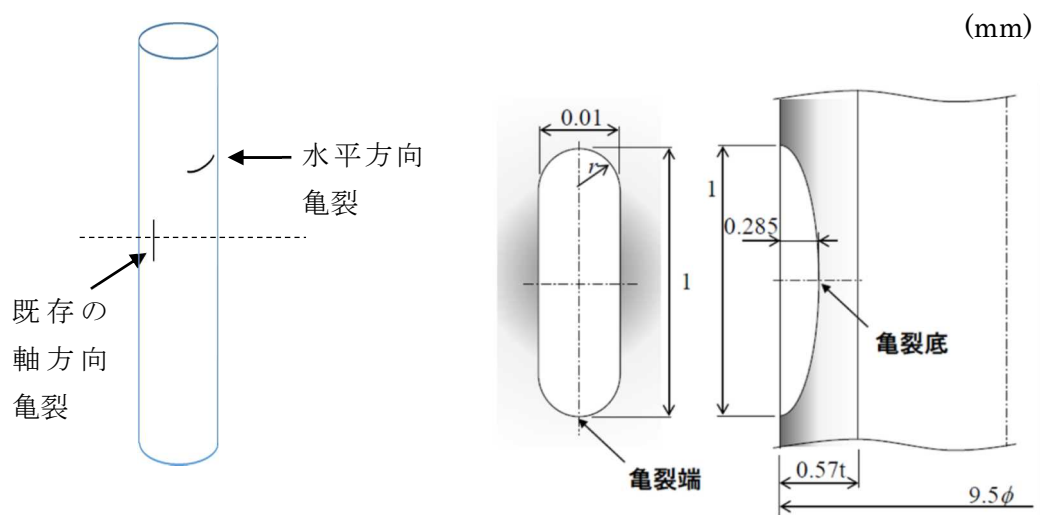
図2 亀裂の概略位置及び軸方向亀裂の寸法
