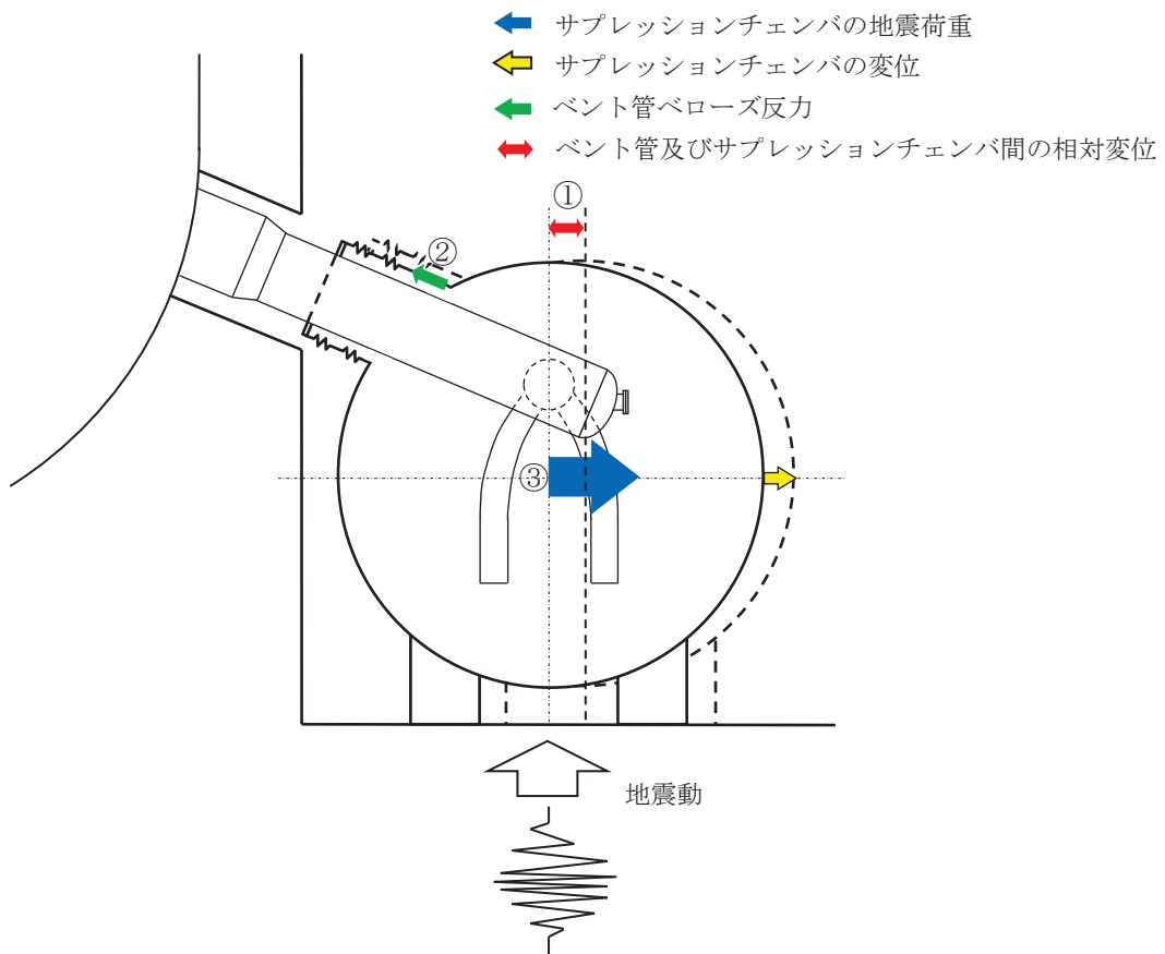
図2 抑制室の荷重伝達イメージ
