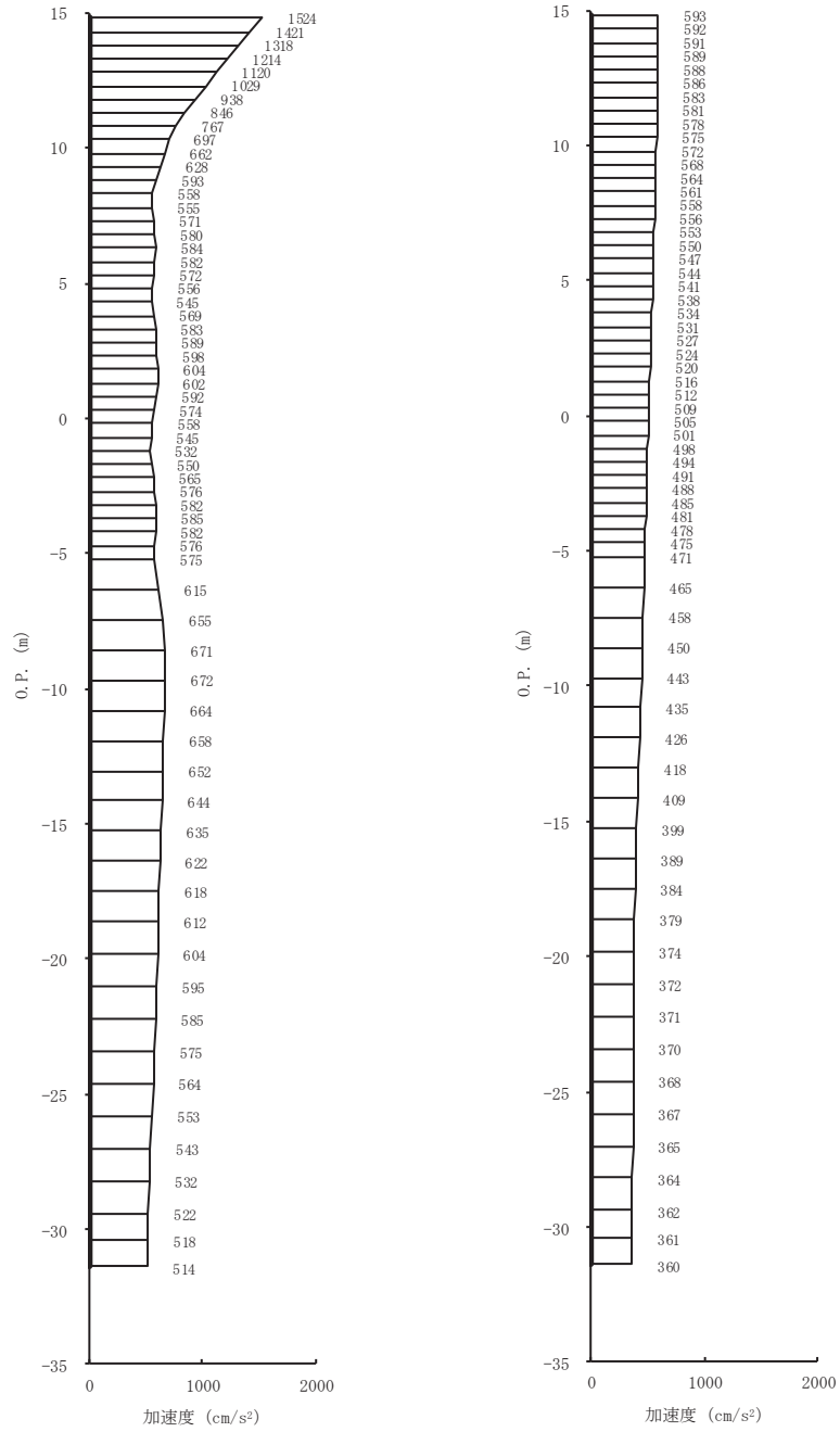
(a) S s - D 2 (-+) 水平 (b) S s - D 2 (-+) 鉛直 図 4-2(23) 最大加速度分布図 (23/28) (No. 1 揚水井戸, 解析ケース④)
