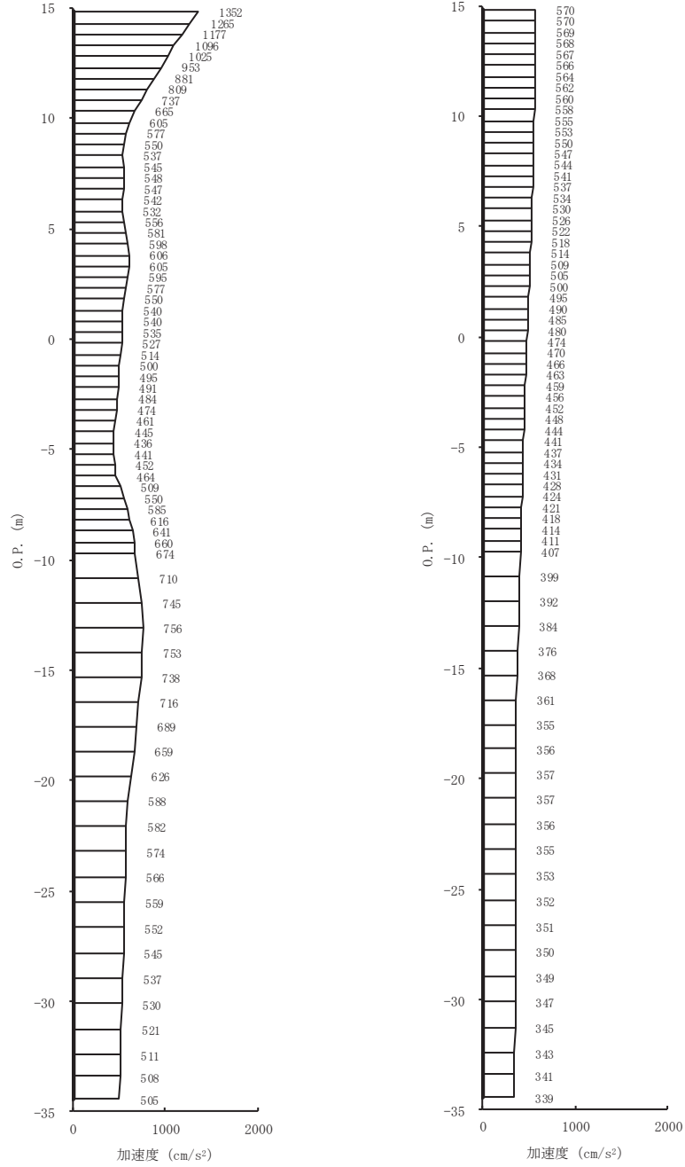
(a) S s - D 2 (-+) 水平 (b) S s - D 2 (-+) 鉛直 図 4-5(16) 最大加速度分布図 (16/28) (No. 2 揚水井戸, 解析ケース③)
