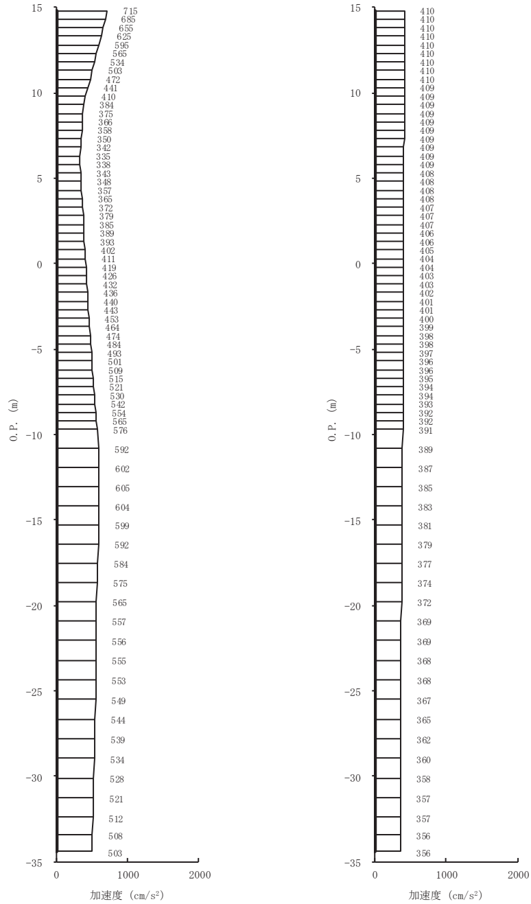
(a) S s - F 2 (-+) 水平 (b) S s - F 2 (-+) 鉛直 図 4-6(12) 最大加速度分布図 (12/14) (No. 2 揚水井戸, 解析ケース⑤)
