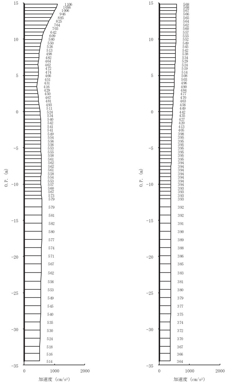
(a) S s - D 1 (++) 水平 (b) S s - D 1 (++) 鉛直 図 4-10(8) 最大加速度分布図 (8/28) (No. 4 揚水井戸, 解析ケース②)
