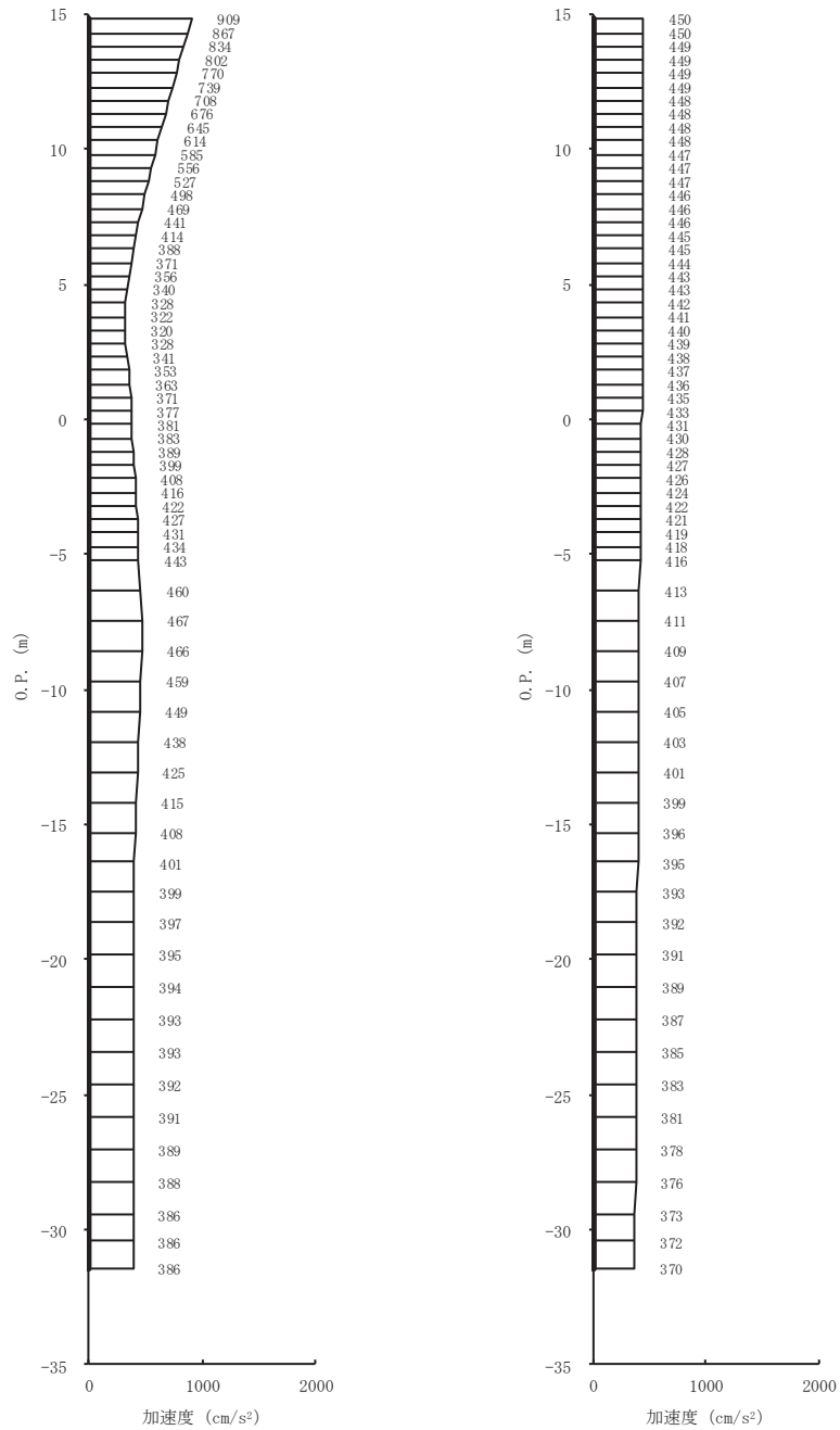
(a) S_s - D 1 (+ +) 水平 (b) S_s - D 1 (+ +) 鉛直 図 4-3(1) 最大加速度分布図 (1/14) (No. 1 揚水井戸, 解析ケース⑤)
