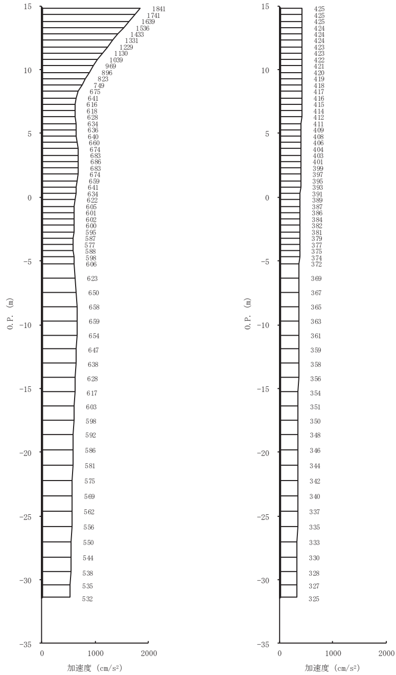
(a) S s - F 2 (++) 水平 (b) S s - F 2 (++) 鉛直 図 4-1(5) 最大加速度分布図 (5/28) (No.1 揚水井戸, 解析ケース①)
