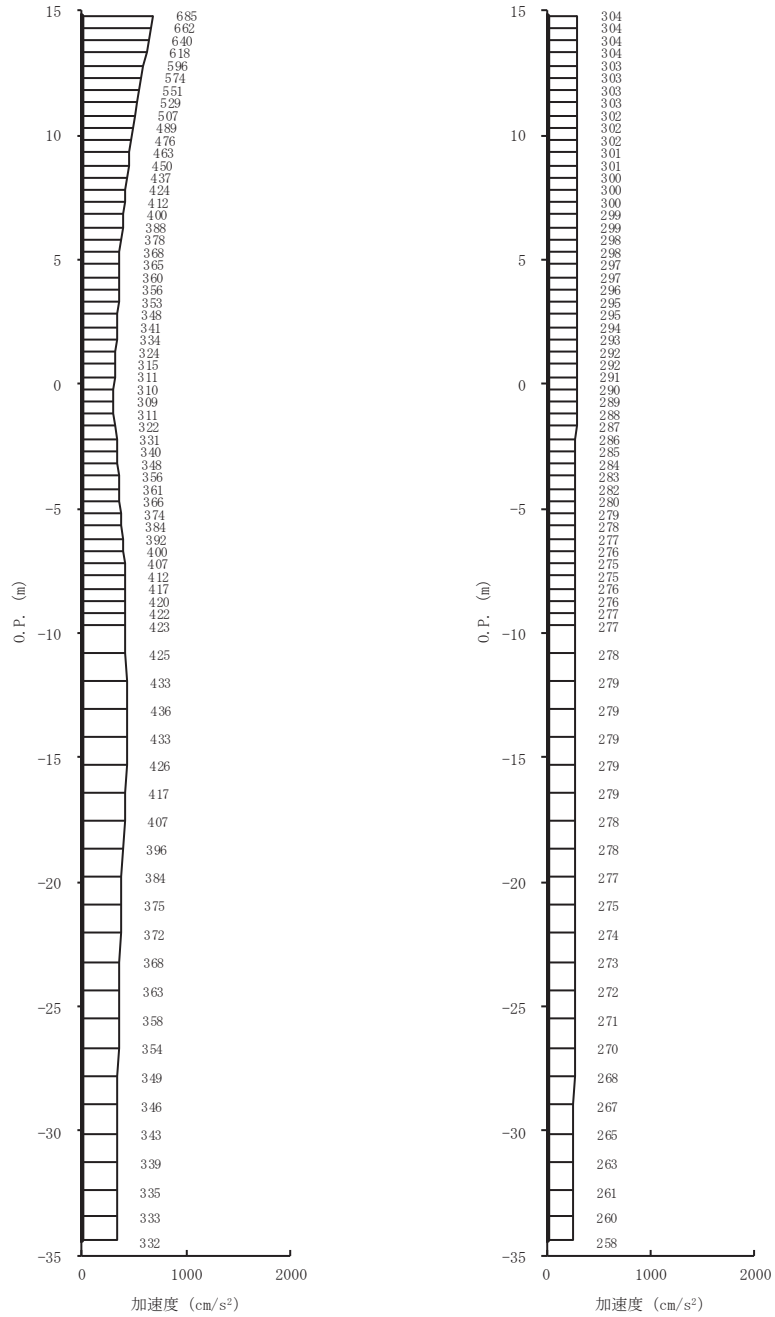
(a) S s - F 1 (-+) 水平 (b) S s - F 1 (-+) 鉛直 図 4-6(11) 最大加速度分布図 (11/14) (No. 2 揚水井戸, 解析ケース⑤)
