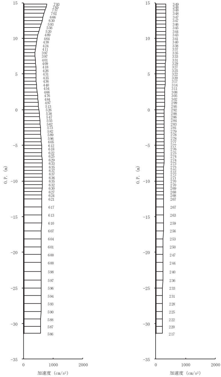
(a) S s - N 1 (-+) 水平 (b) S s - N 1 (-+) 鉛直 図 4-8(7) 最大加速度分布図 (7/28) (No. 3 揚水井戸, 解析ケース①)
