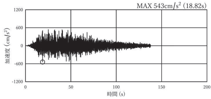
図 4-1(5) 加速度時刻歴波形（接続柵③）（水平方向：S s - D 1 : 解析ケース②）
