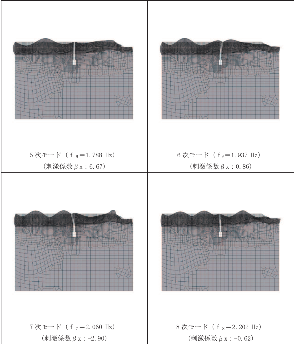
図 3-7(11) 固有値解析結果 (2/3) (No. 4 揚水井戸)
