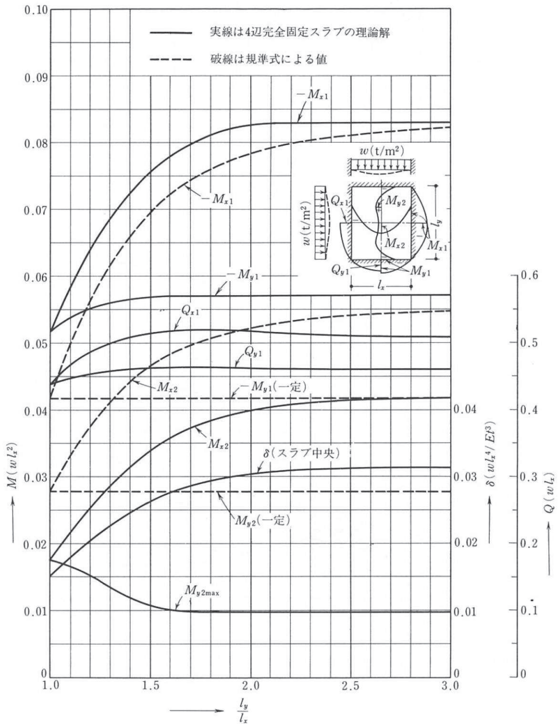
図 3-10(1) 等分布荷重時 4 辺固定スラブの応力図と中央点のたわみ \delta ( \nu = 0 ) (鉄筋コンクリート構造計算基準・同解説 ( (社) 日本建築学会, 1991 年) )
