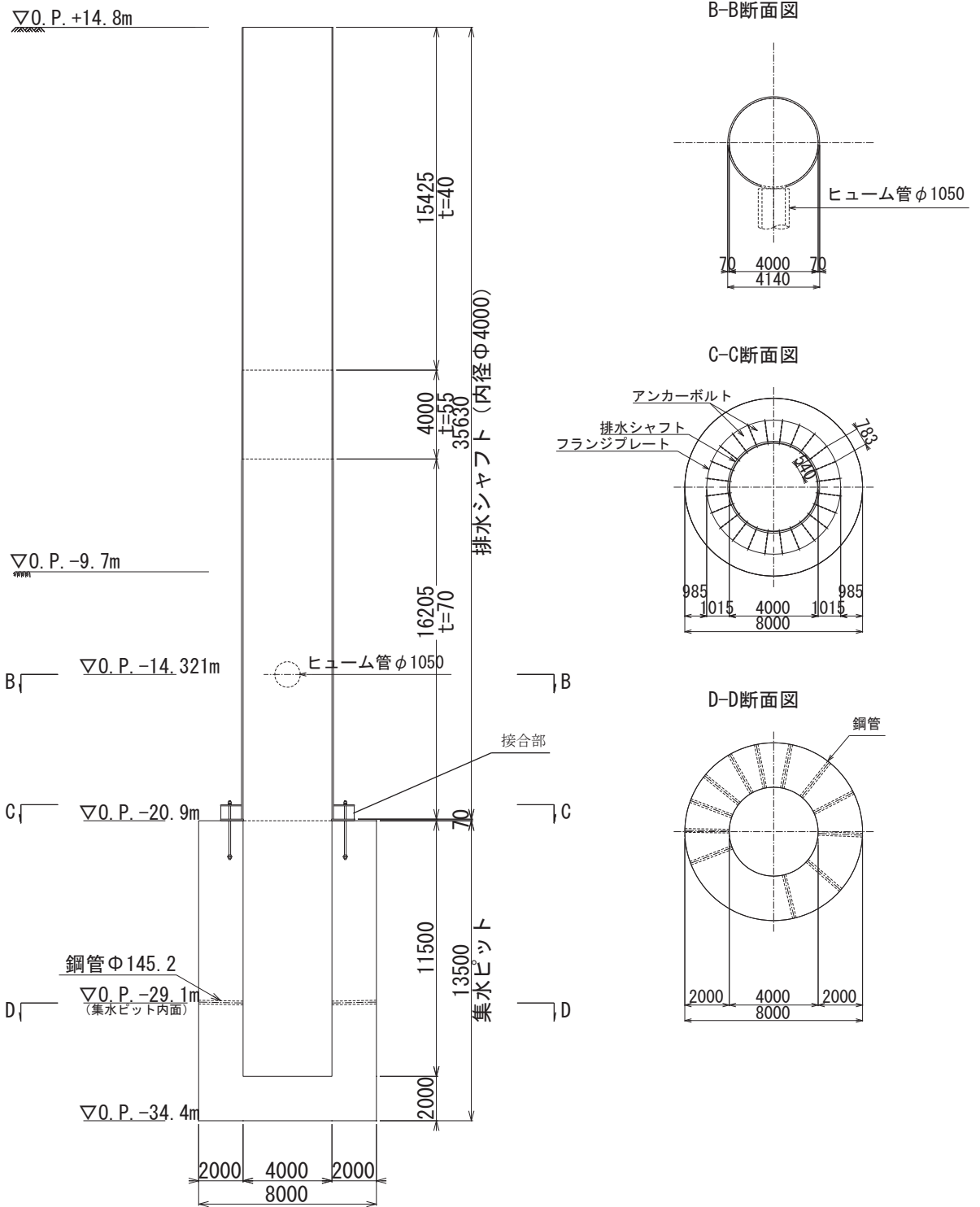
図 2-3(2) No.2 揚水井戸 構造図 (単位: mm)
