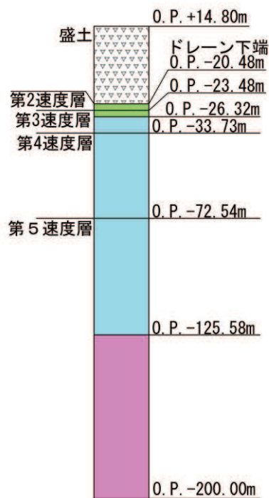
断面⑤
