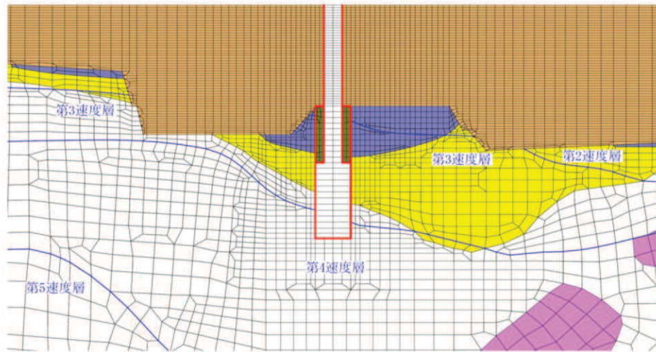
図 3-18(1) ジョイント要素の配置図 (No.1 揚水井戸)
