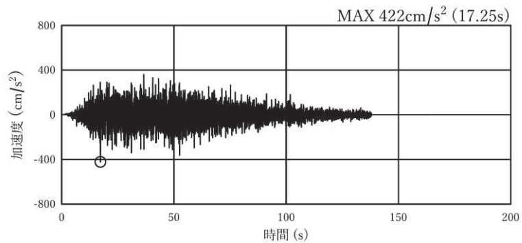
図 4-1(8) 加速度時刻歴波形（接続柵④）（鉛直方向：S s - D 1 : 解析ケース②）
