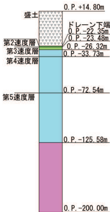
断面④
