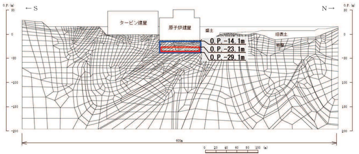
(1) NS 断面
