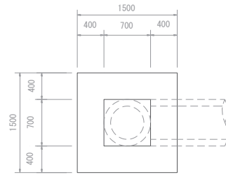
B-B 断面图
