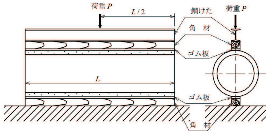
図2 外圧試験概要図
