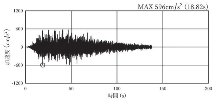
図 4-1(7) 加速度時刻歴波形（接続柵④）（水平方向：S s - D 1 : 解析ケース②）
