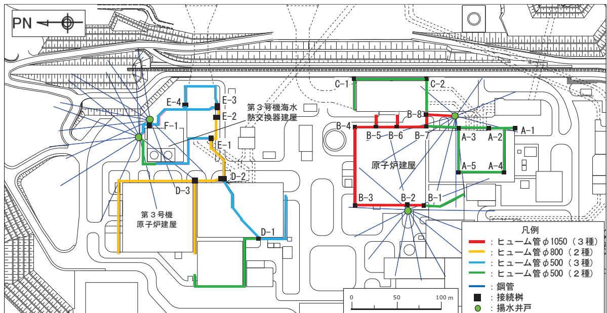
図 2-1 接続桝の設置位置
