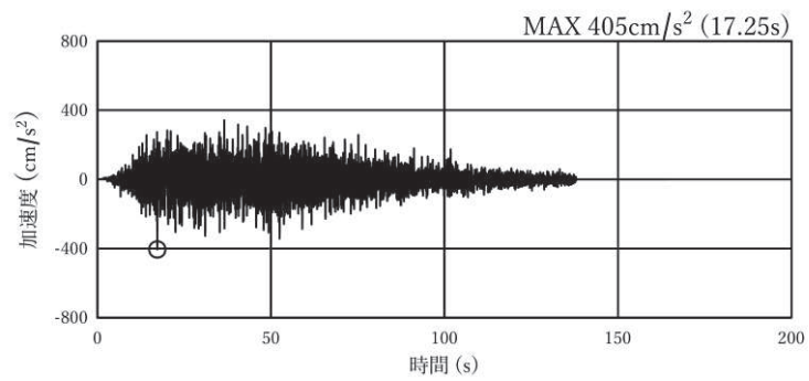
図 4-1(6) 加速度時刻歴波形（接続柵③）（鉛直方向：S s - D 1 : 解析ケース②）
