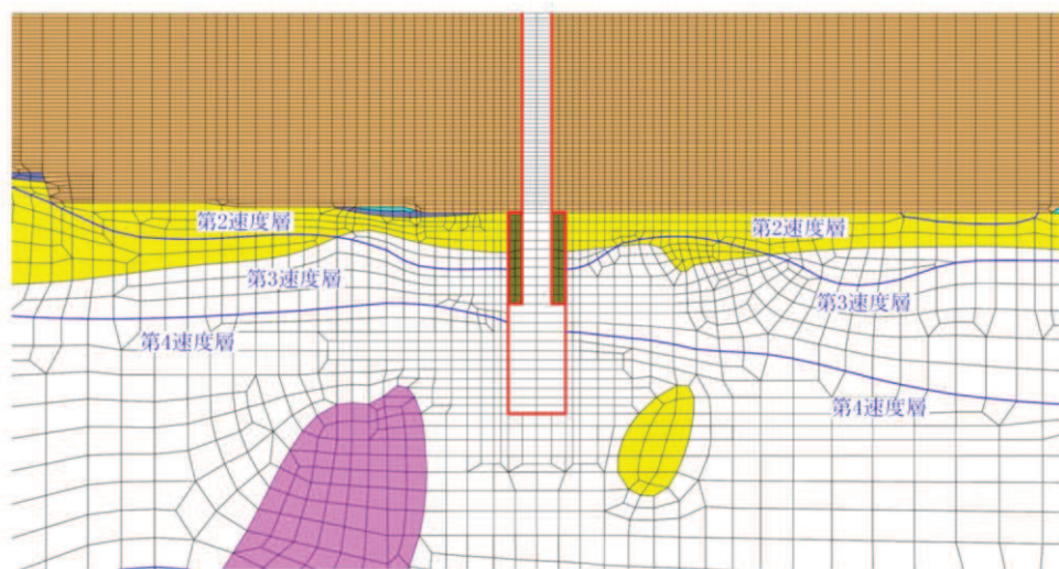
図 3-18(2) ジョイント要素の配置図 (No.2 揚水井戸)
