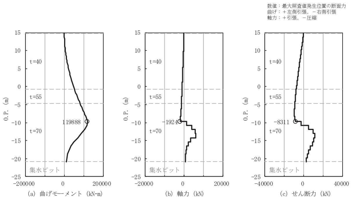
(No.2 揚水井戸 (板厚 t=70\text{mm} ) , S_s-N1 (++) , 7.78s)
