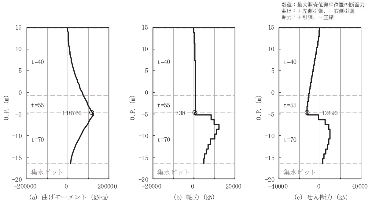
(No.1 揚水井戸 (板厚 t=55\text{mm} ) , S_s-N1 (++) , 7.77s)
