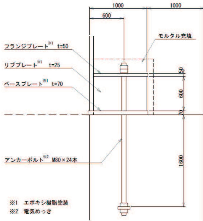
図 2-3(5) 接合部詳細図 (No. 1~4 揚水井戸共通)
