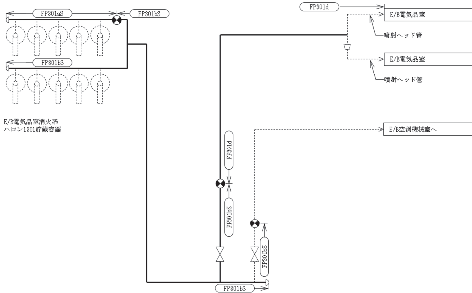
ハロンガス消火設備概略系統図 (その 56)
