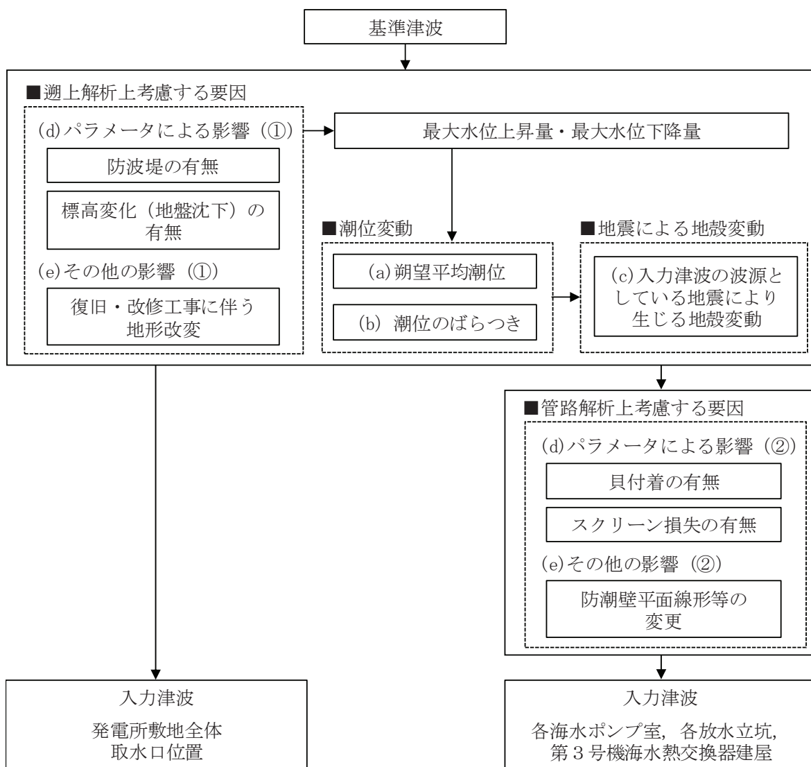
図 1.5-1 入力津波高さの算定フロー
