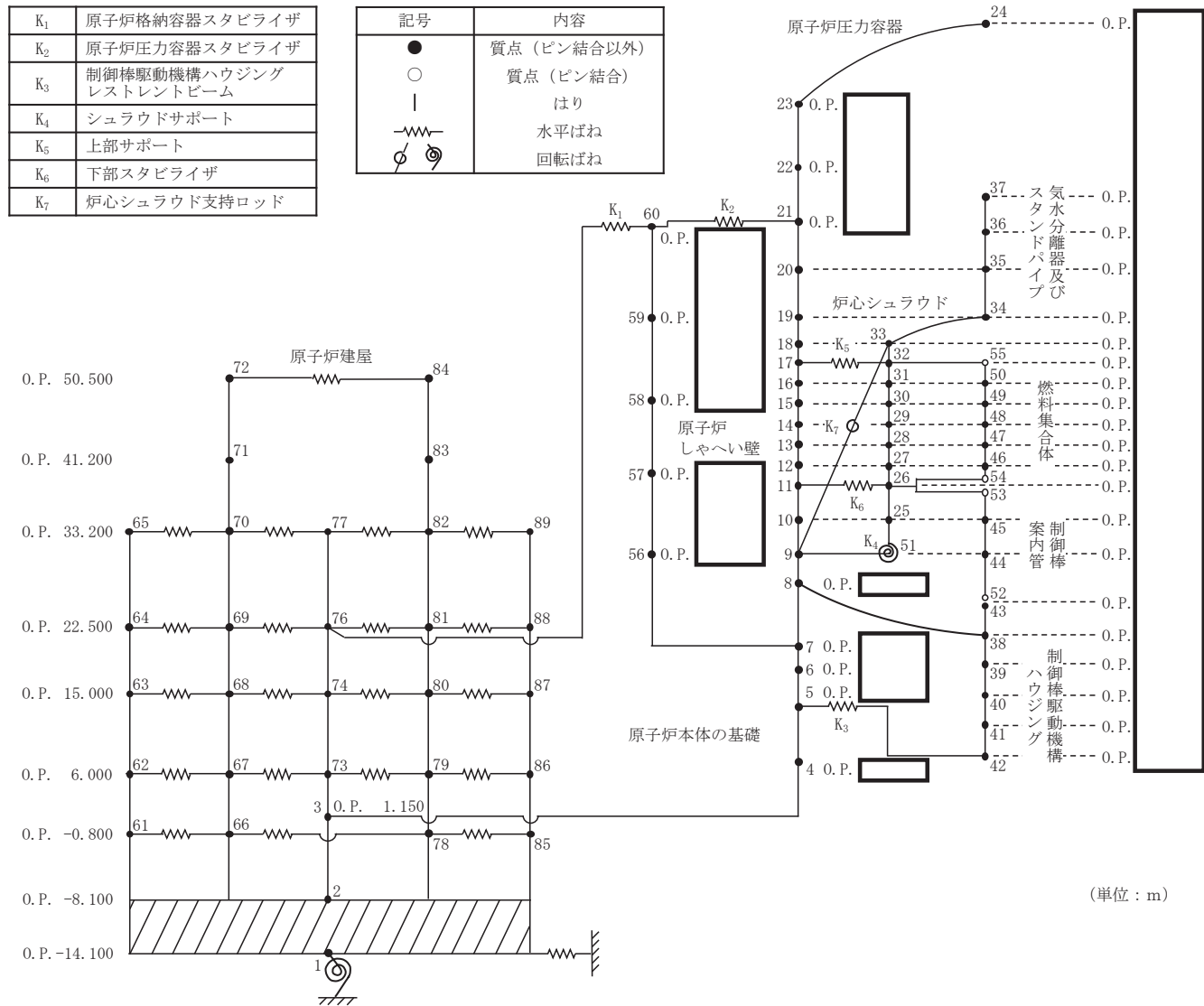
図1 炉内構造物系地震応答解析モデル図 (NS方向)
