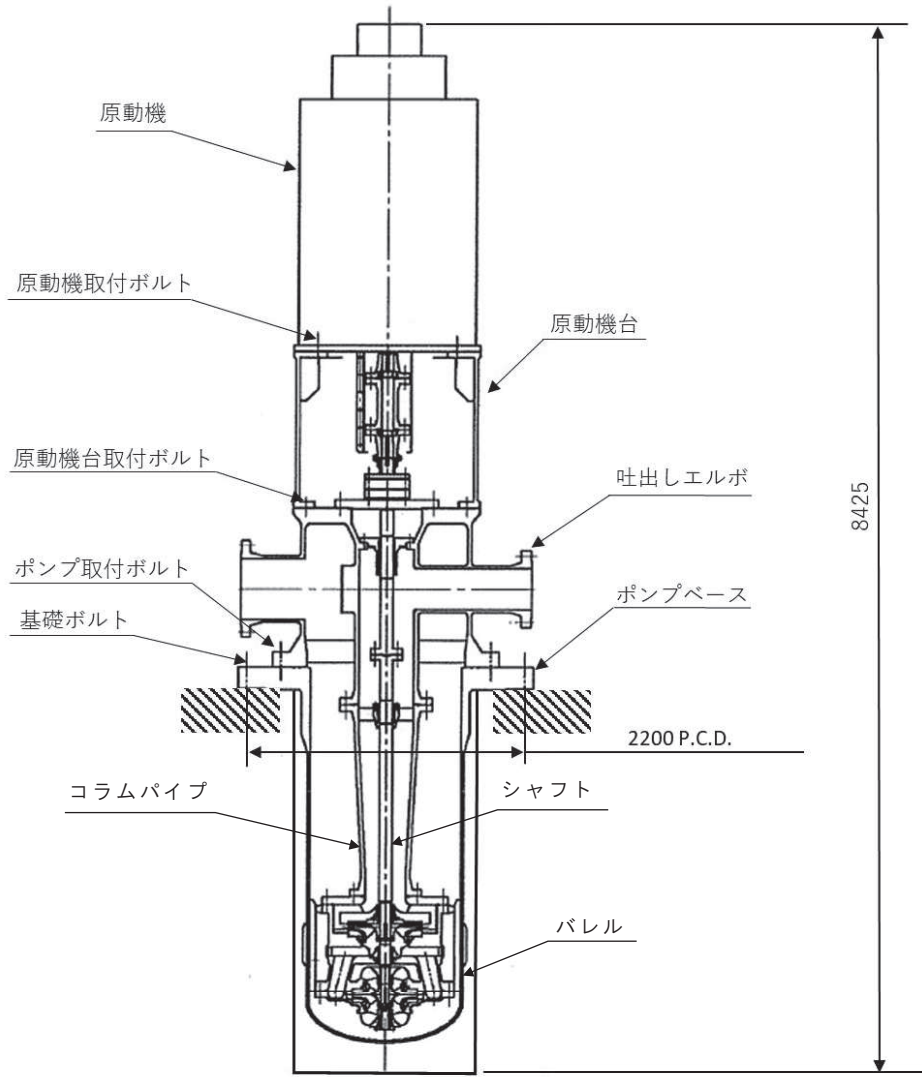
構造概要図
