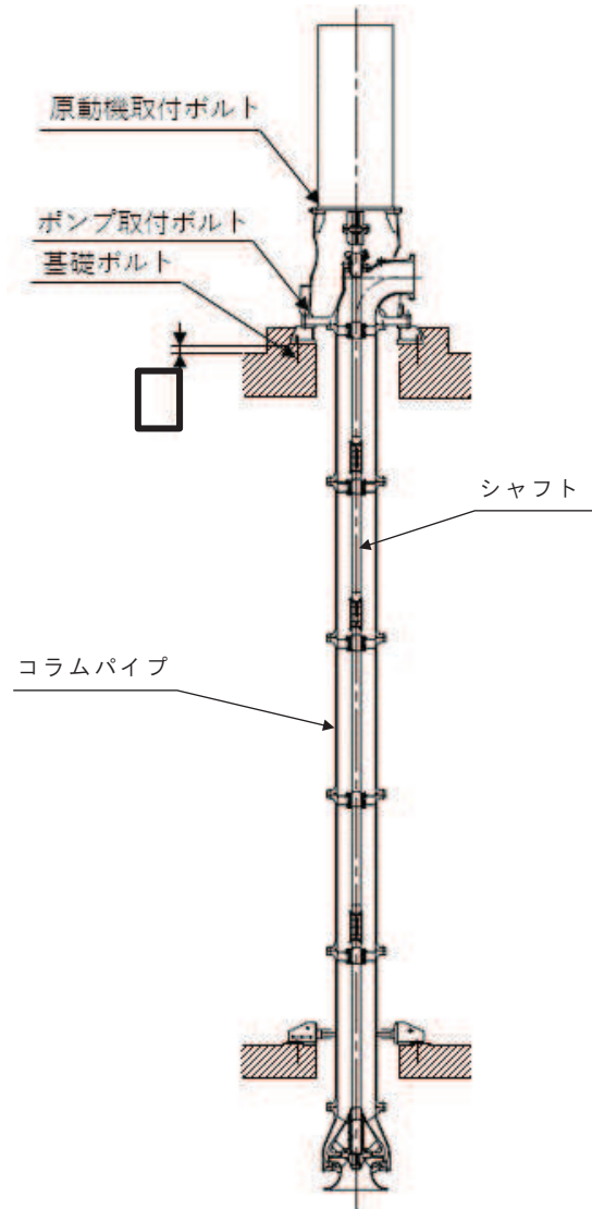
構造概要図
