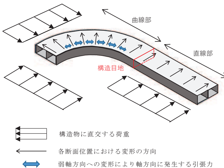
図 3-3-30 取水路（標準部）における変形
