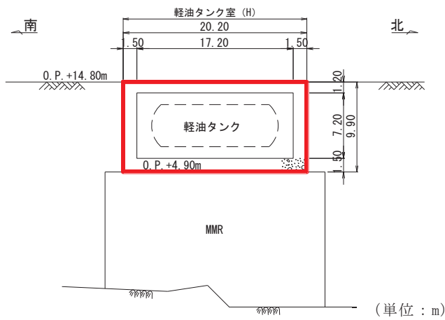
図 3-3-36 軽油タンク室 (H) 断面図 (A-A 断面, 南北)
