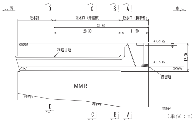
図 3-3-49 取水口縦断面図 (E-E 断面, 東西)
