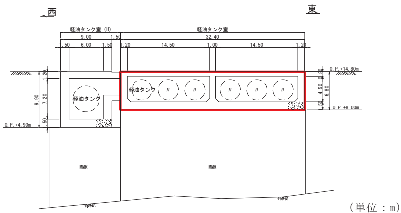
図 3-3-33 軽油タンク室断面図 (B-B 断面, 東西 (タンク室))
