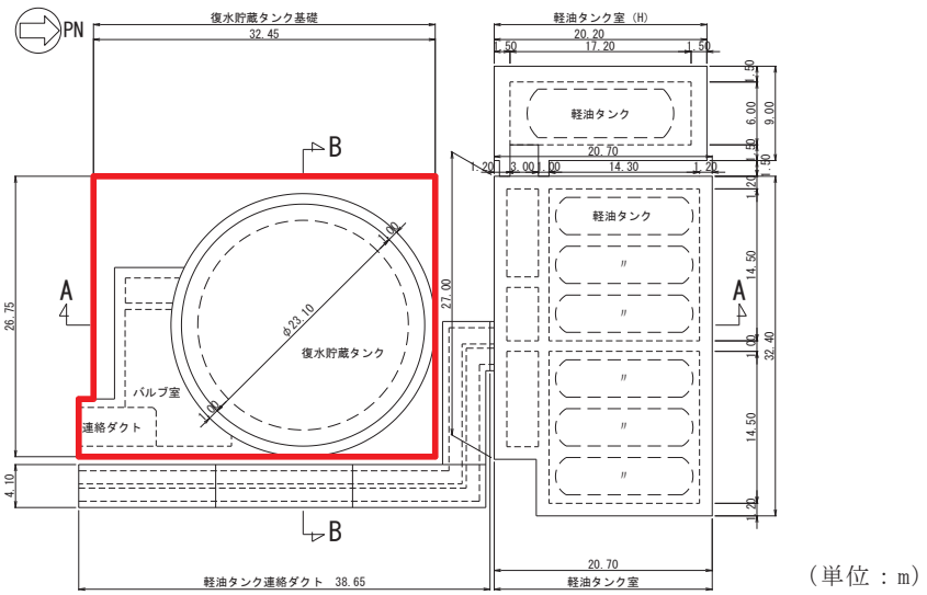
図 3-3-50 復水貯蔵タンク基礎平面図
