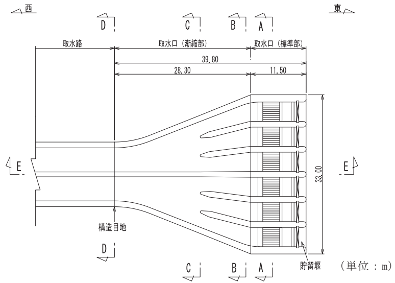
図 3-3-44 取水口，貯留堰平面図
