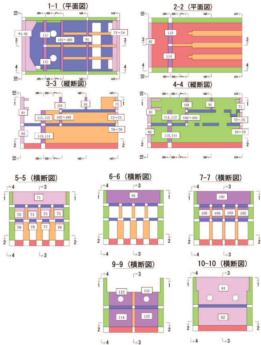
図 3-3-71(3) 第 3 号機海水ポンプ室 評価位置図
