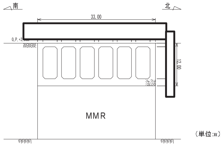
図 3-3-45 取水口断面図 (A-A 断面，南北 (標準部))
