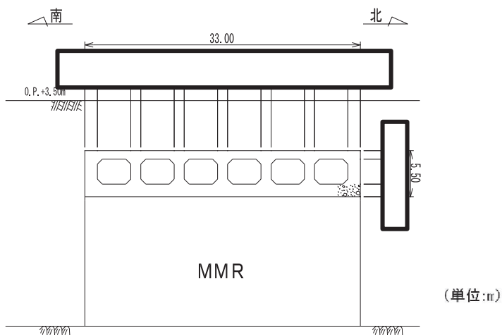
図 3-3-46 取水口断面図 (B-B 断面，南北 (漸縮部))
