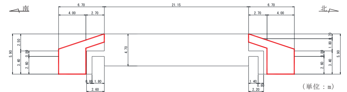
図 3-3-26 原子炉機器冷却海水配管ダクト (鉛直部) 水平断面図 (断面⑤)
