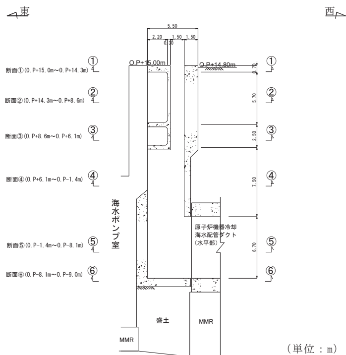
図 3-3-21 原子炉機器冷却海水配管ダクト（鉛直部）縦断図（B-B 断面）
