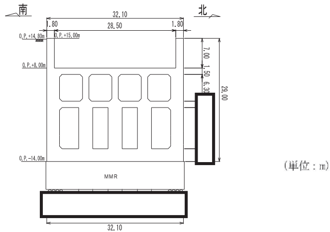
図 3-3-57 第 3 号機海水ポンプ室縦断面図 (A-A 断面, 南北 (スクリーンエリア))
