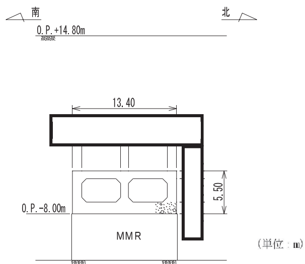
図 3-3-29 取水路（標準部）断面図（A-A 断面）
