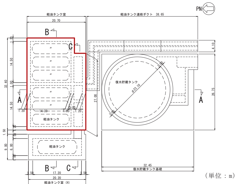
図 3-3-31 軽油タンク室平面図
