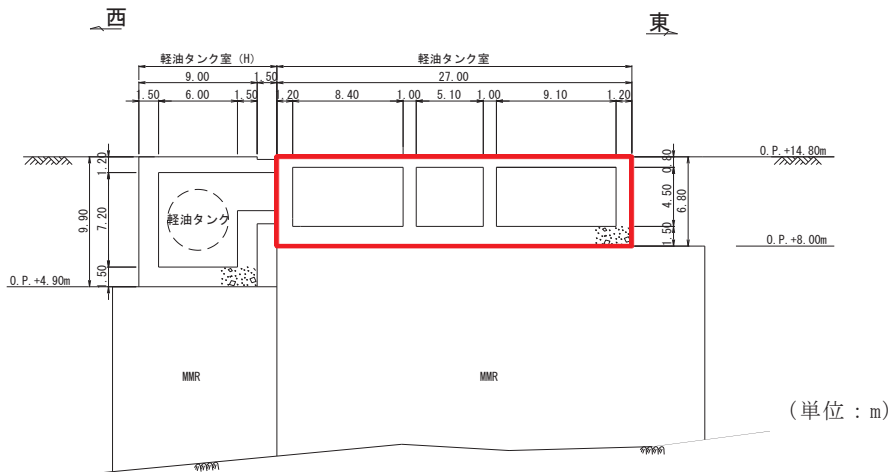
図 3-3-34 軽油タンク室断面図 (C-C 断面, 東西 (ポンプ室))
