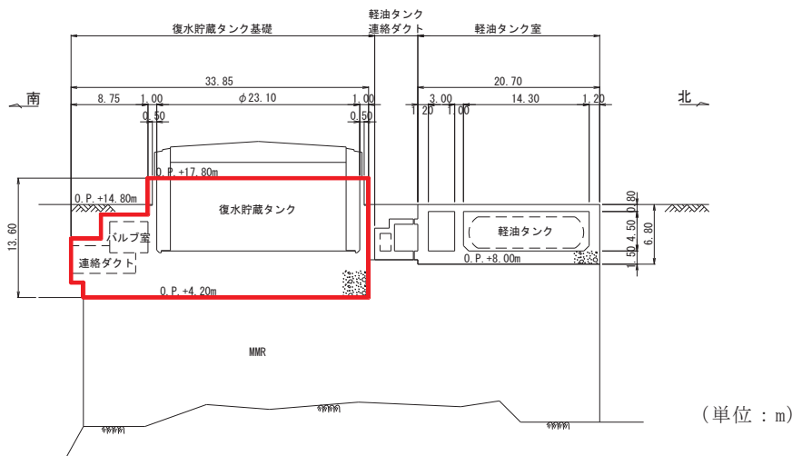
図 3-3-51 復水貯蔵タンク基礎断面図 (A-A 断面, 南北)
