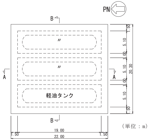
図 3-3-53 ガスタービン発電設備軽油タンク室平面図
