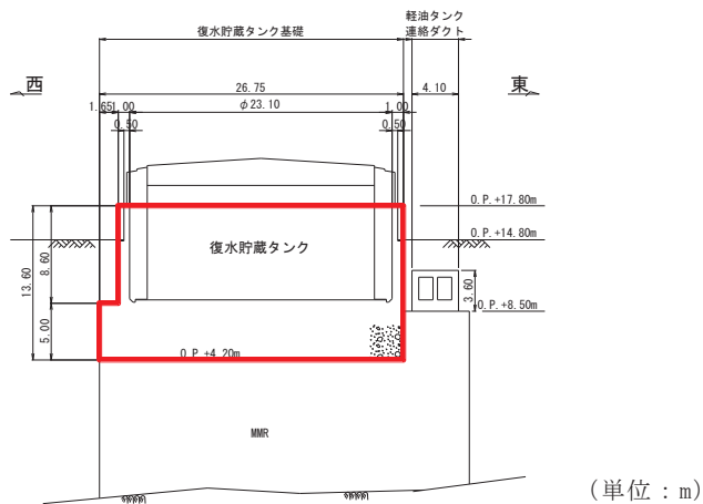
図 3-3-52 復水貯蔵タンク基礎断面図 (B-B 断面, 東西)
