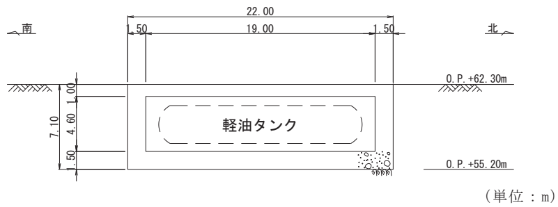
図 3-3-54 ガスタービン発電設備軽油タンク室断面図 (A-A 断面, 南北)
