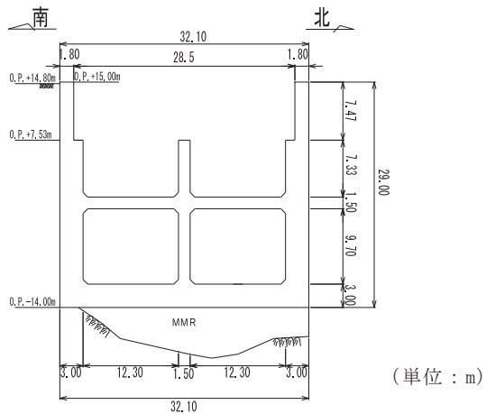
図 3-3-58 第 3 号機海水ポンプ室断面図 (B-B 断面, 南北 (循環水ポンプエリア))
