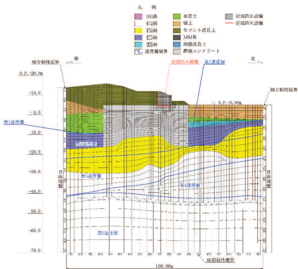
図 3-4-32 解析モデル
