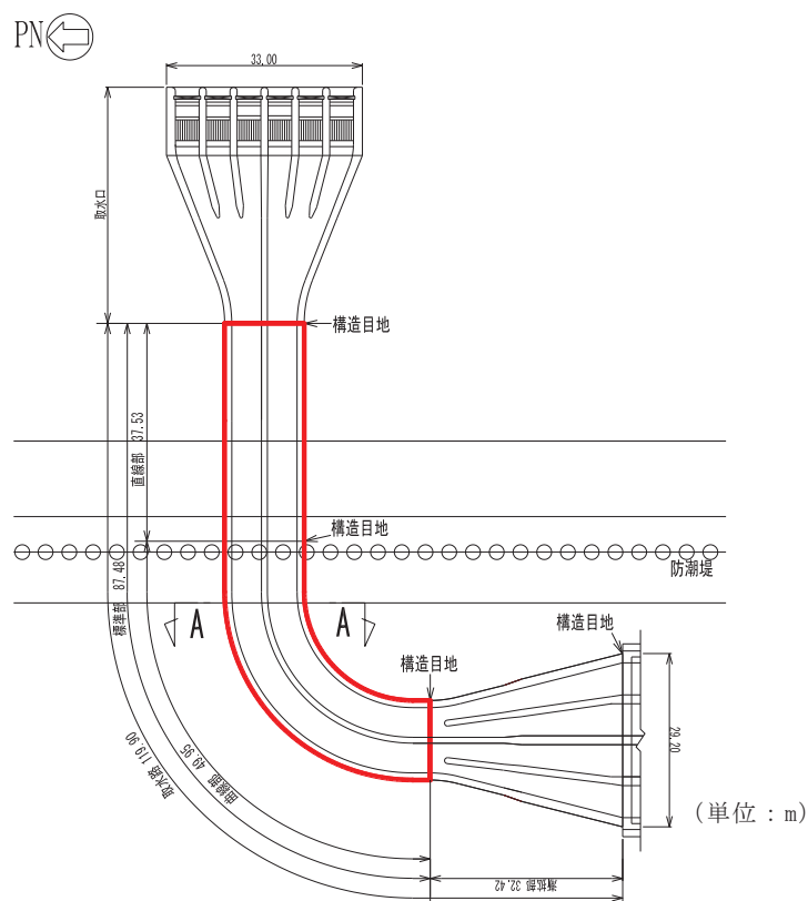
図 3-3-28 取水路（標準部）平面図
