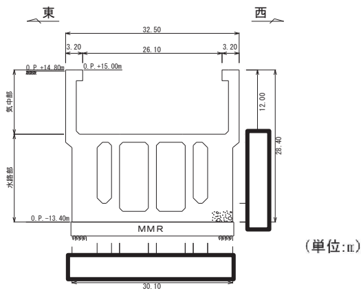
図 3-3-39 海水ポンプ室断面図 (A-A 断面, 東西 (スクリーンエリア))
