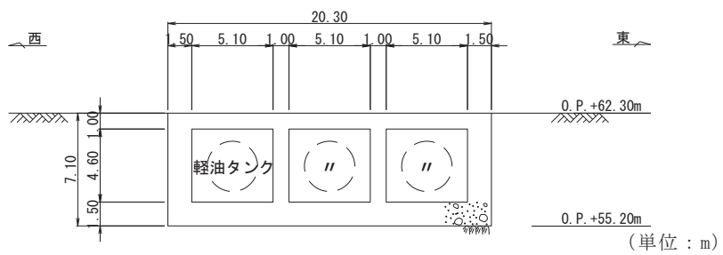
図 3-3-55 ガスタービン発電設備軽油タンク室断面図 (B-B 断面, 東西)
