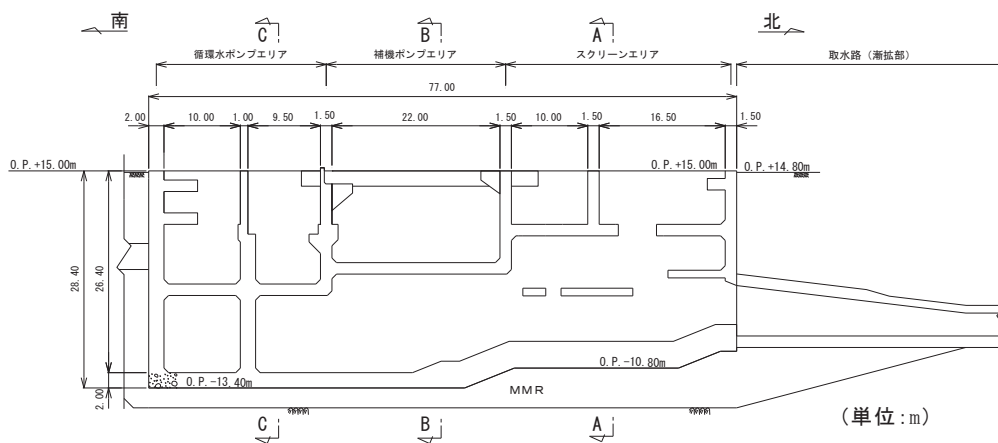
図 3-3-42 海水ポンプ室断面図 (D-D 断面, 南北)
