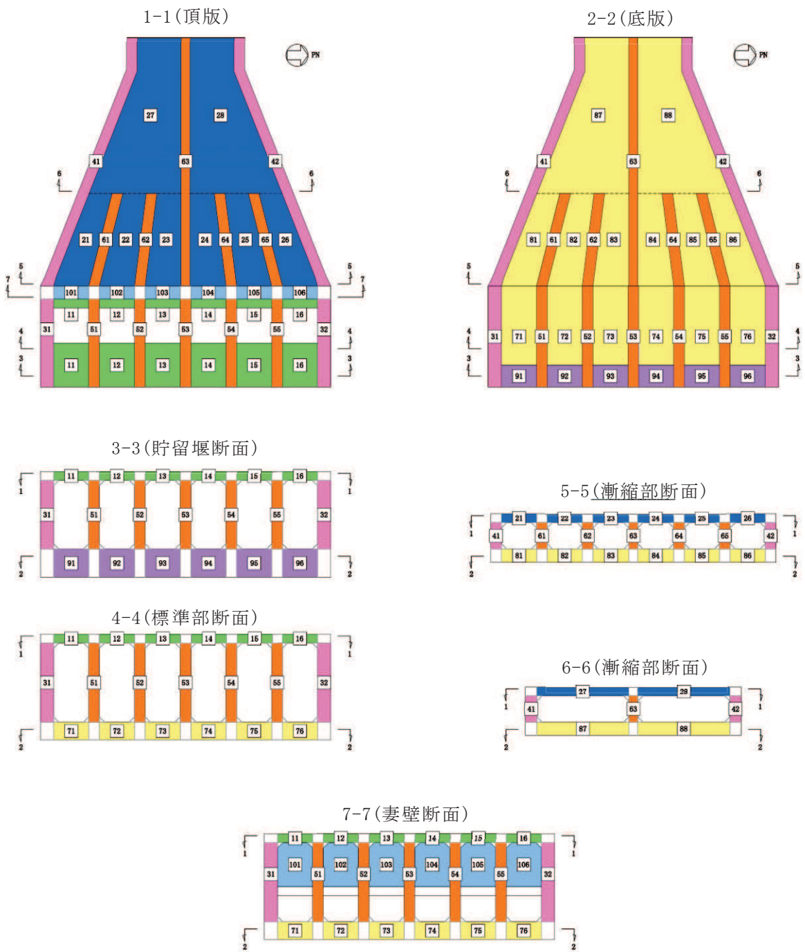
図 3-3-65 取水口，貯留堰 評価位置図 (曲げ・軸力系の破壊及びせん断破壊)
