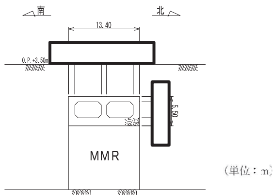
図 3-3-48 取水口断面図 (D-D 断面, 南北 (漸縮部))
