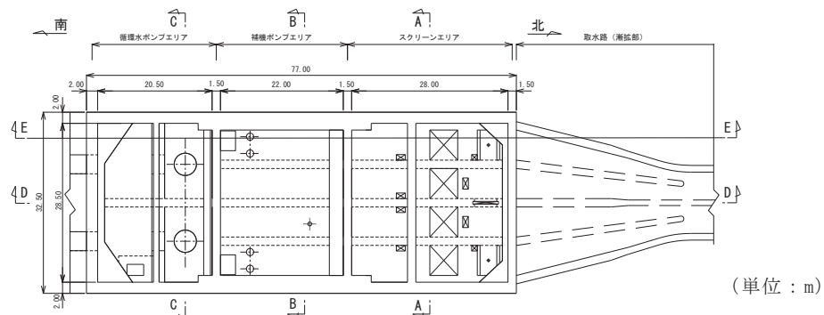
図 4.10-2 海水ポンプ室平面図
