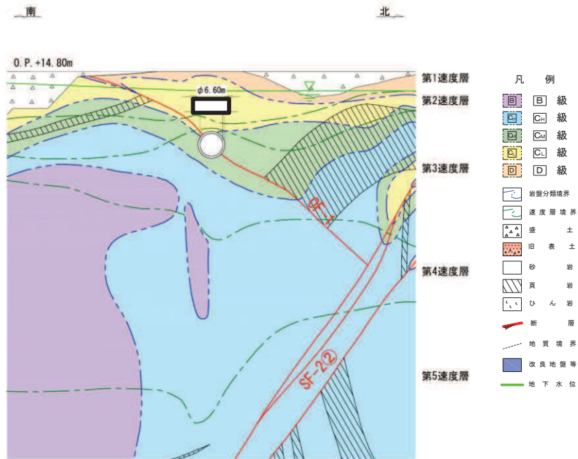
図 4.5-12 排気筒連絡ダクト（岩盤部） 評価対象断面図（断面⑦）
