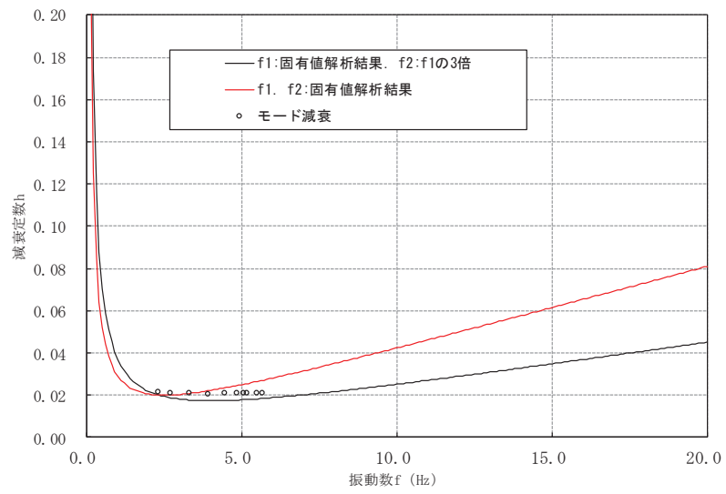
Rayleigh 減衰
