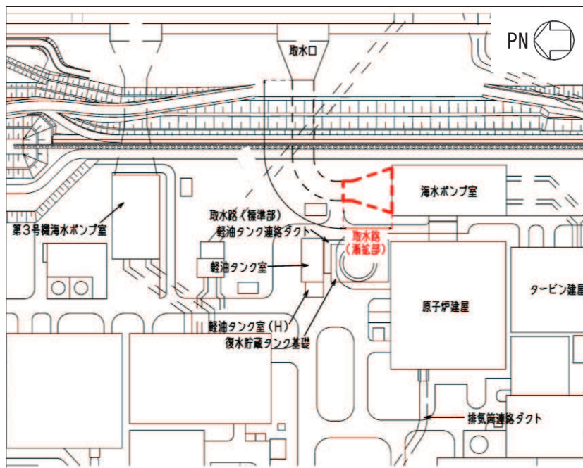
図 4.7-1 取水路（漸拡部）配置図
