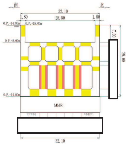
A-A 断面
