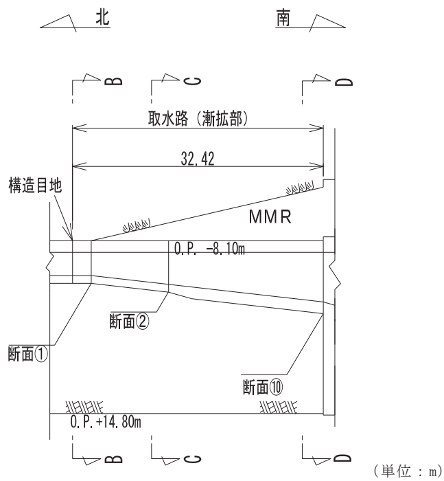
図 4.7-5 取水路（漸拡部）縦断図（A-A 断面）及び候補断面位置
