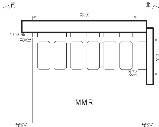
図11.2-7 取水口断面図 (A-A断面図, 標準部)
