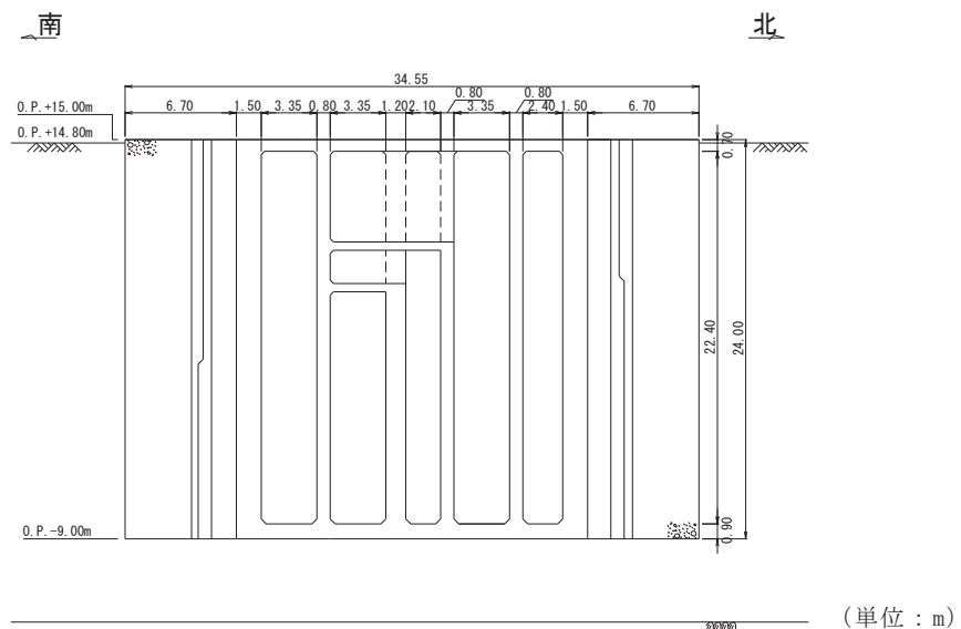
図 4.6-4 原子炉機器冷却海水配管ダクト（鉛直部）断面図（B-B 断面）
