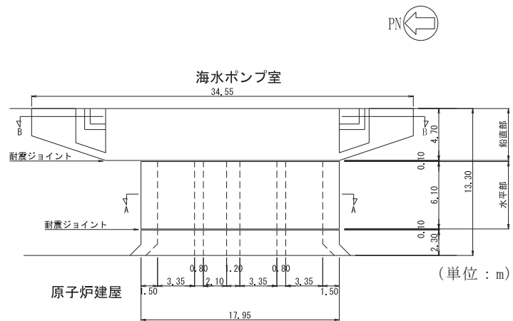
図 4.6-2 原子炉機器冷却海水配管ダクト平面図
