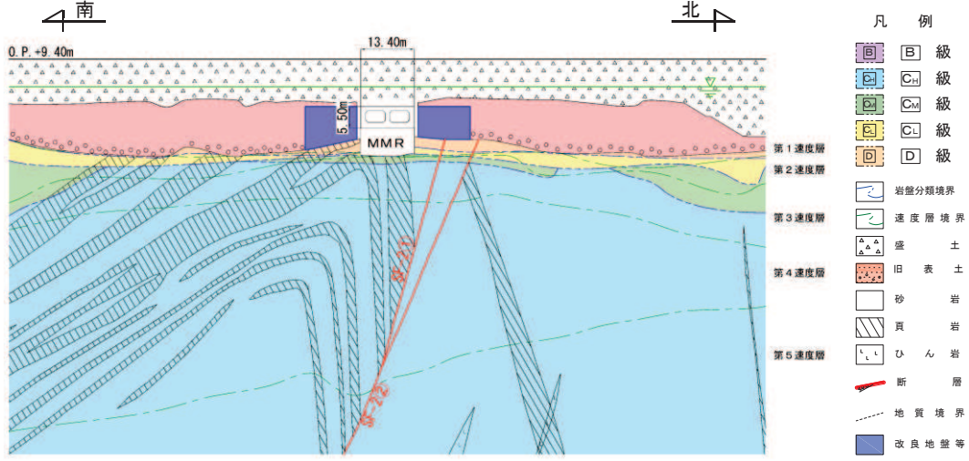
図 4.12-14(2) 取水路（標準部）地震時荷重算出断面図（断面③：直線部）
