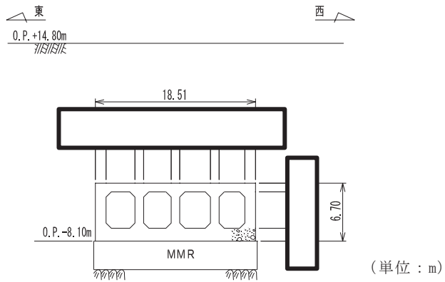
図 4.7-7 取水路（漸拡部）断面図（C-C 断面：断面②）
