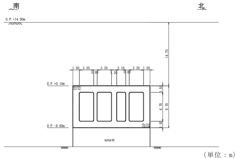
図 4.6-3 原子炉機器冷却海水配管ダクト（水平部）断面図（A-A 断面）
