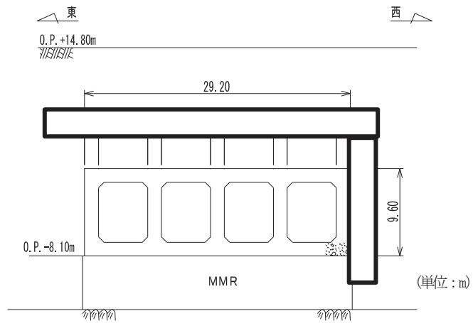
図 4.7-3 取水路（漸拡部）断面図（A-A 断面）
