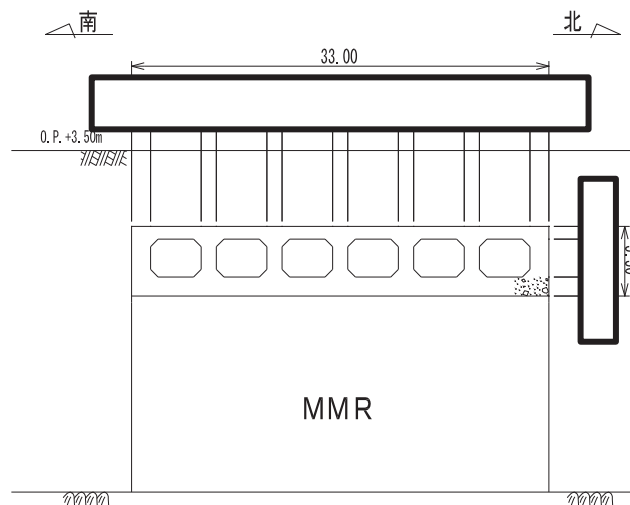
図 4.11-4 取水口断面図 (B-B 断面，南北 (漸縮部))
