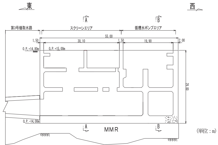
図 4.15-5 第3号機海水ポンプ室縦断面図 (C-C断面)
