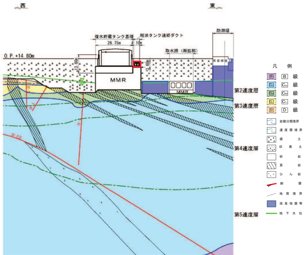
図 4.4-9 軽油タンク連絡ダクト地質断面図 (B-B 断面)
