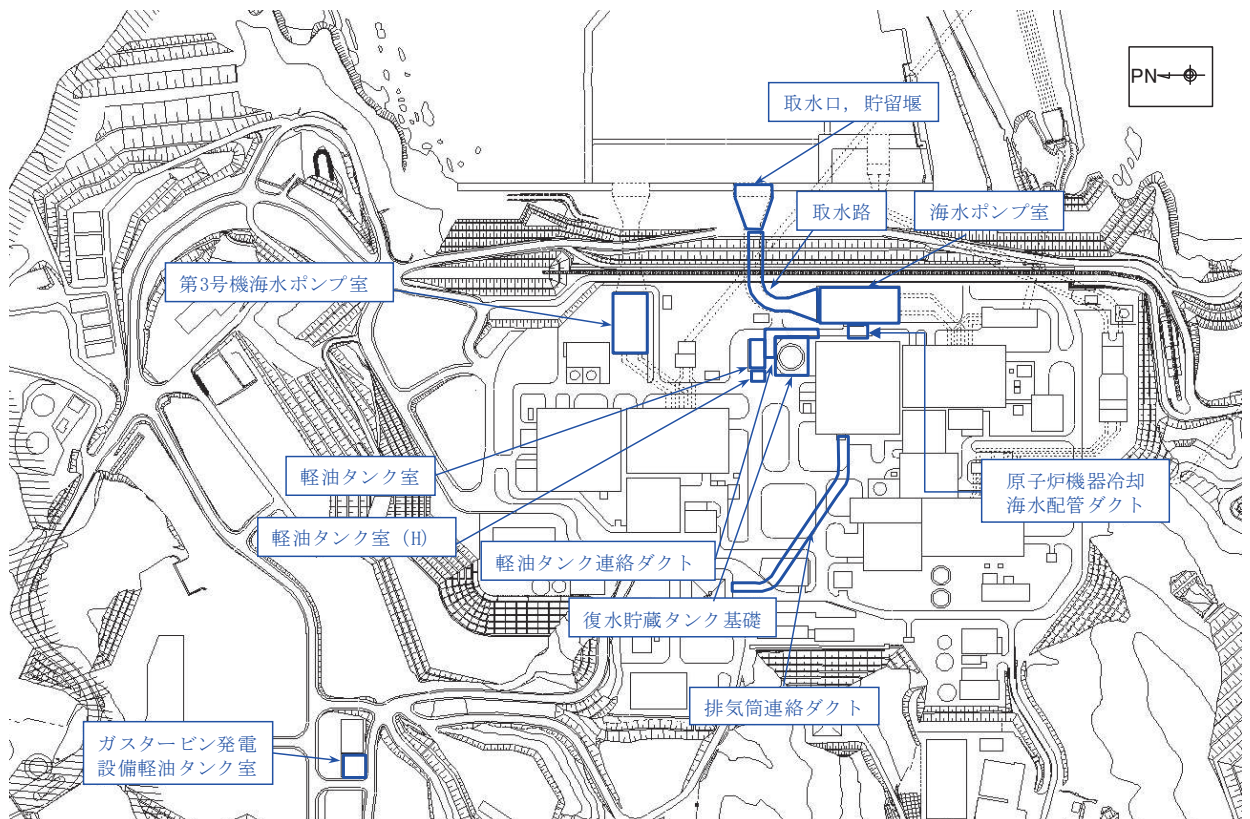
図1-1 屋外重要土木構造物等 位置図
