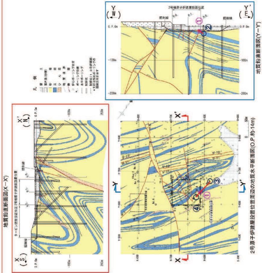
図1-2 OF-4断層の確認位置、性状及び連続性 (第778回審査委員会 資料1-2-1「女川原子力発電所2号炉 地盤(敷地の地形、地質・地質構造)」より抜粋)
