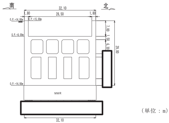
図 4.15-3 第 3 号機海水ポンプ室断面図 (A-A 断面)
