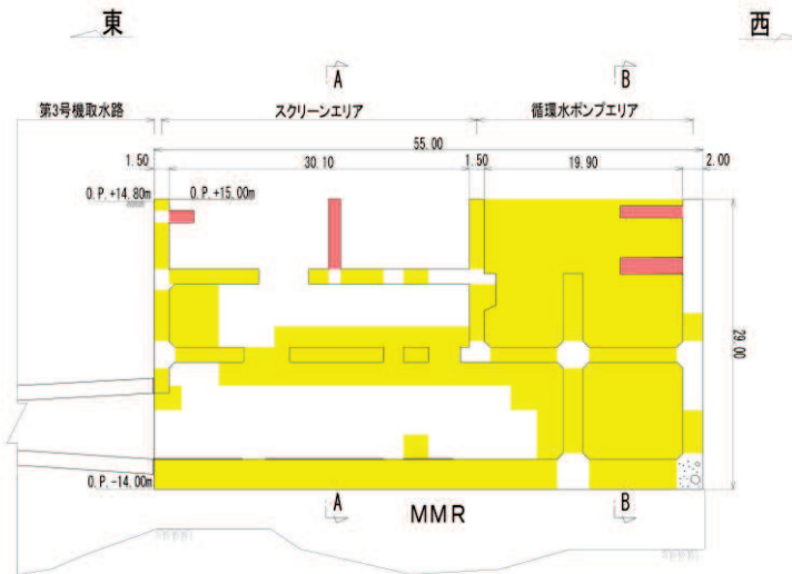
C-C 断面
