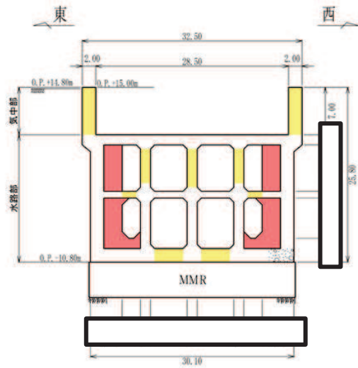
A-A 断面
