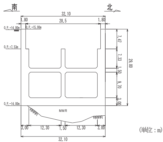
図 4.15-4 第 3 号機海水ポンプ室断面図 (B-B 断面)
