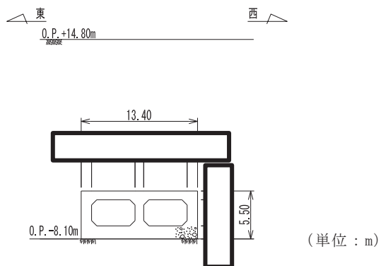
図 4.7-6 取水路（漸拡部）断面図（B-B 断面：断面①）
