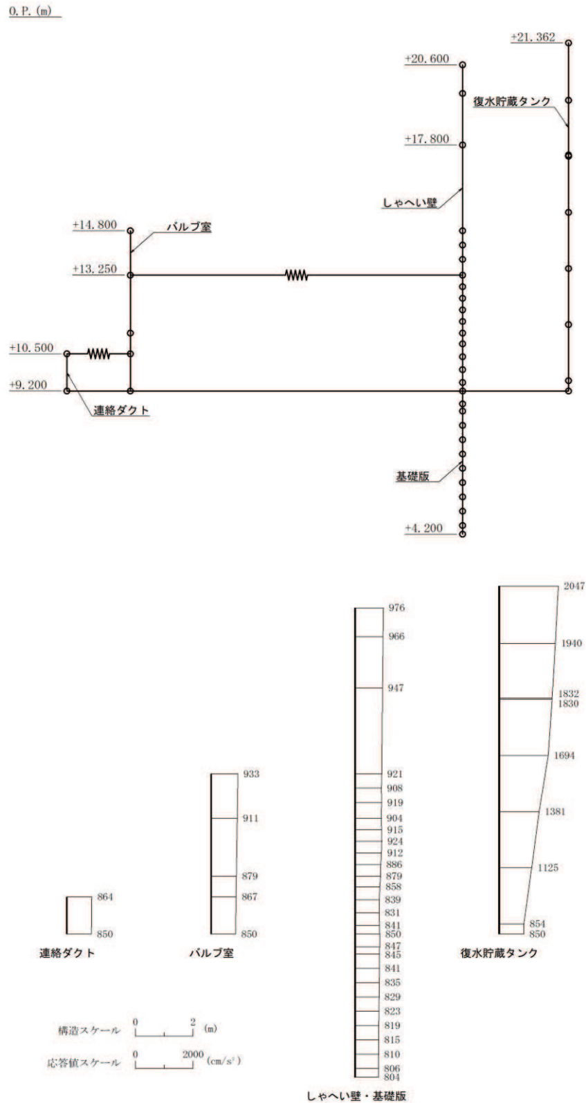
図 4-54(1) 最大加速度分布図 (解析ケース④) (37/42)
