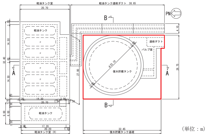
図 2-2 復水貯蔵タンク基礎平面図
