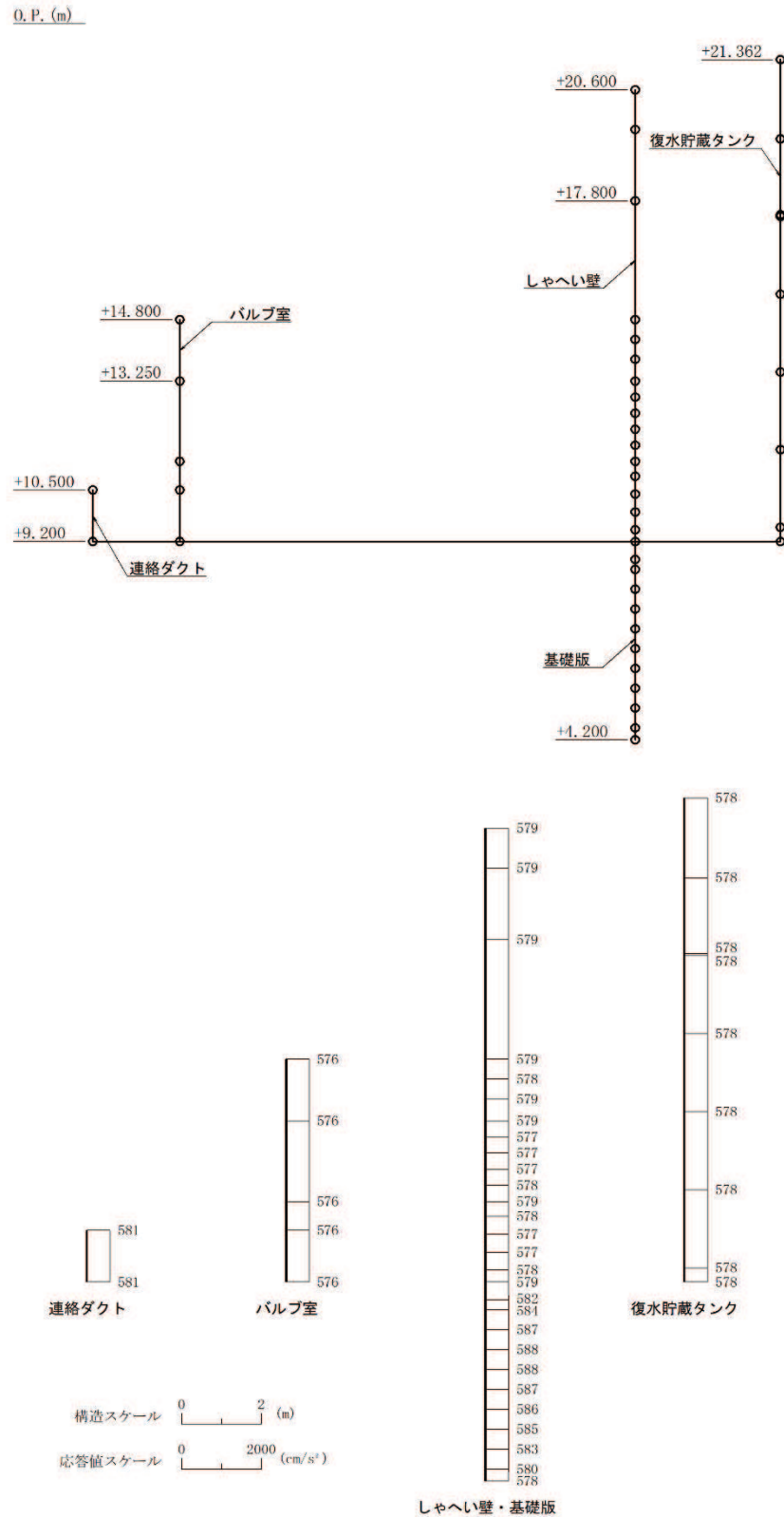
図 4-28 (2) 最大加速度分布図 (解析ケース②) (11/42)
