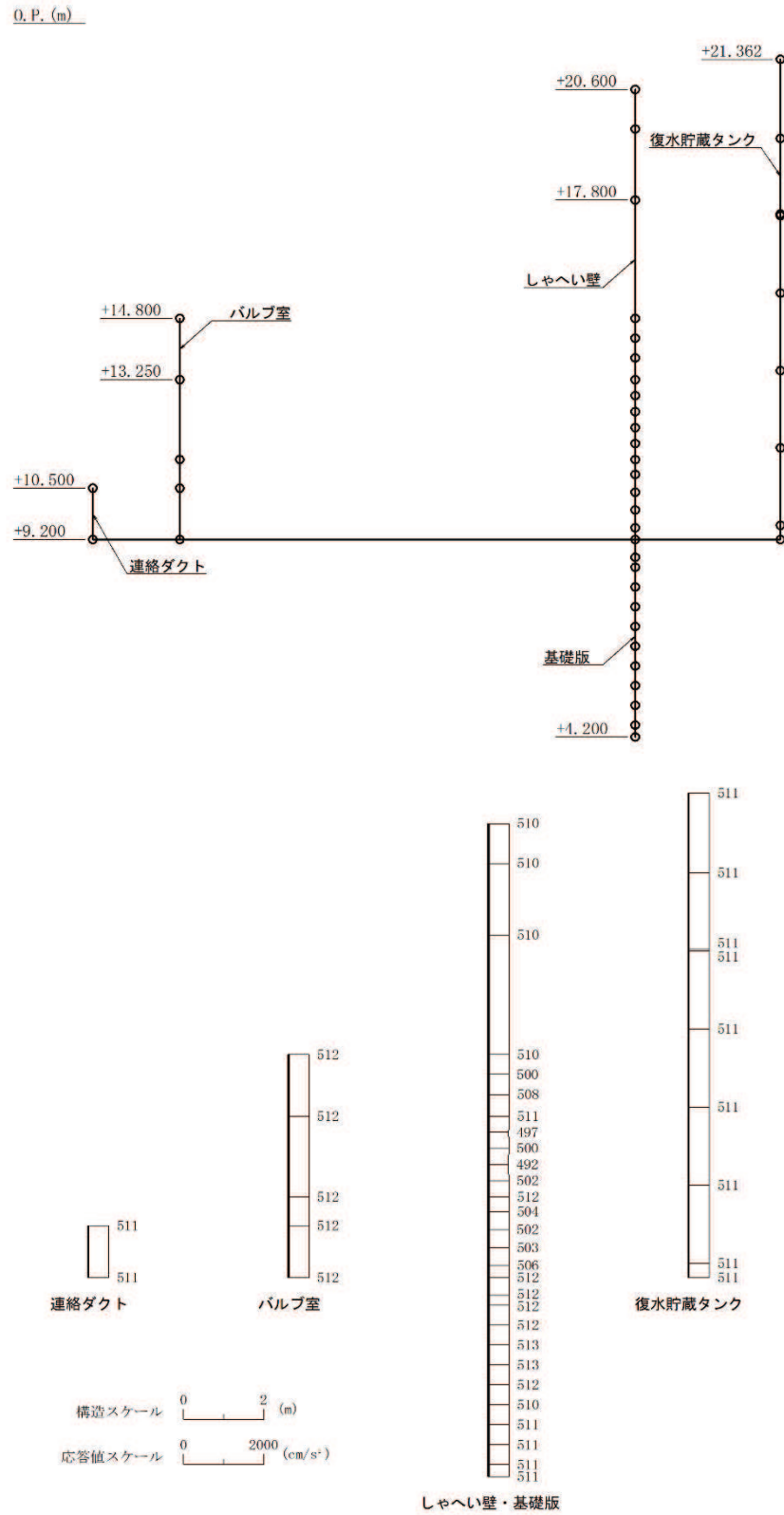
図 4-22(2) 最大加速度分布図 (解析ケース②) (5/42)
