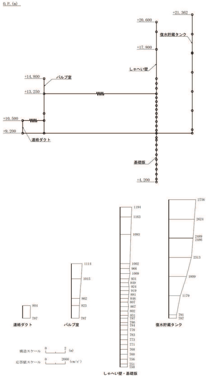
図 4-6(1) 最大加速度分布図 (解析ケース①) (6/17)
