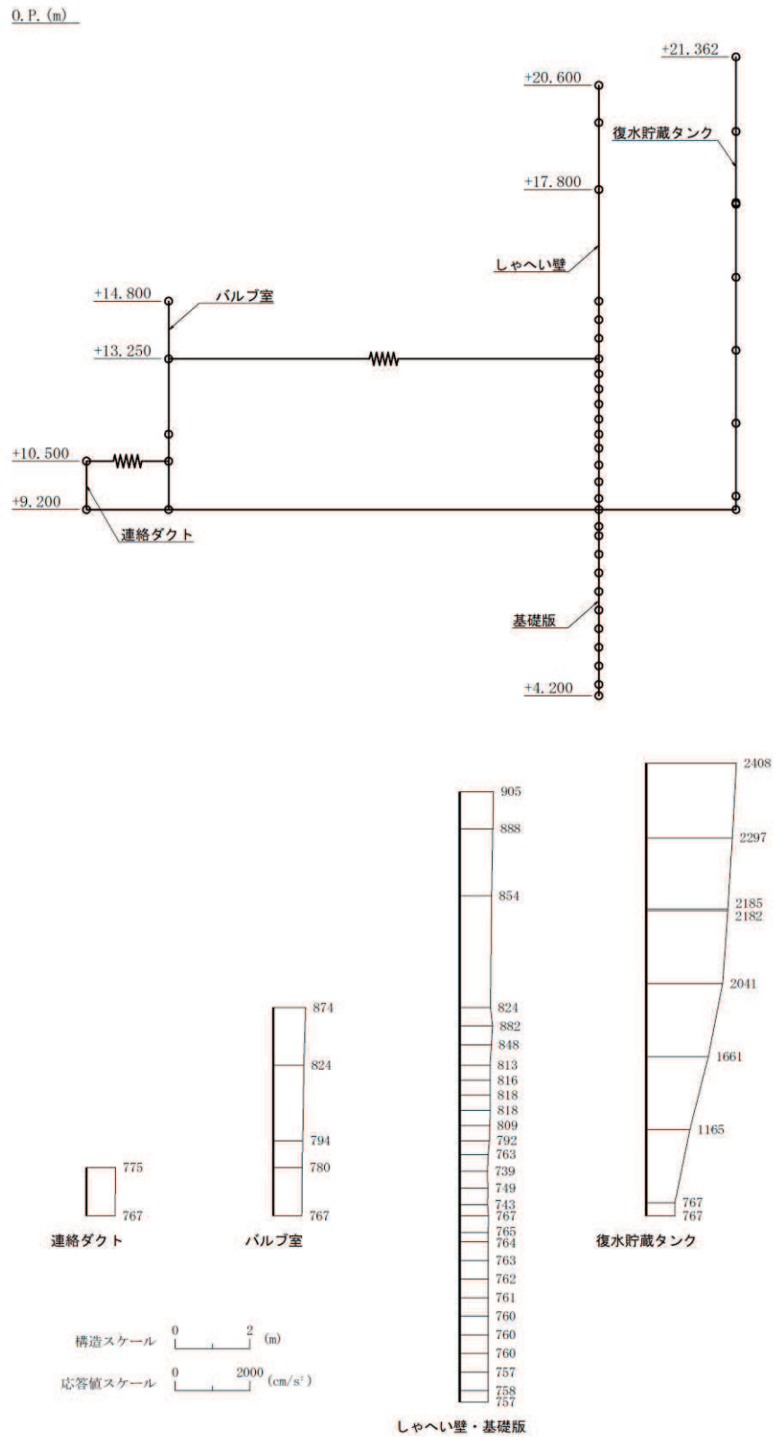
図 4-52(1) 最大加速度分布図 (解析ケース④) (35/42)
