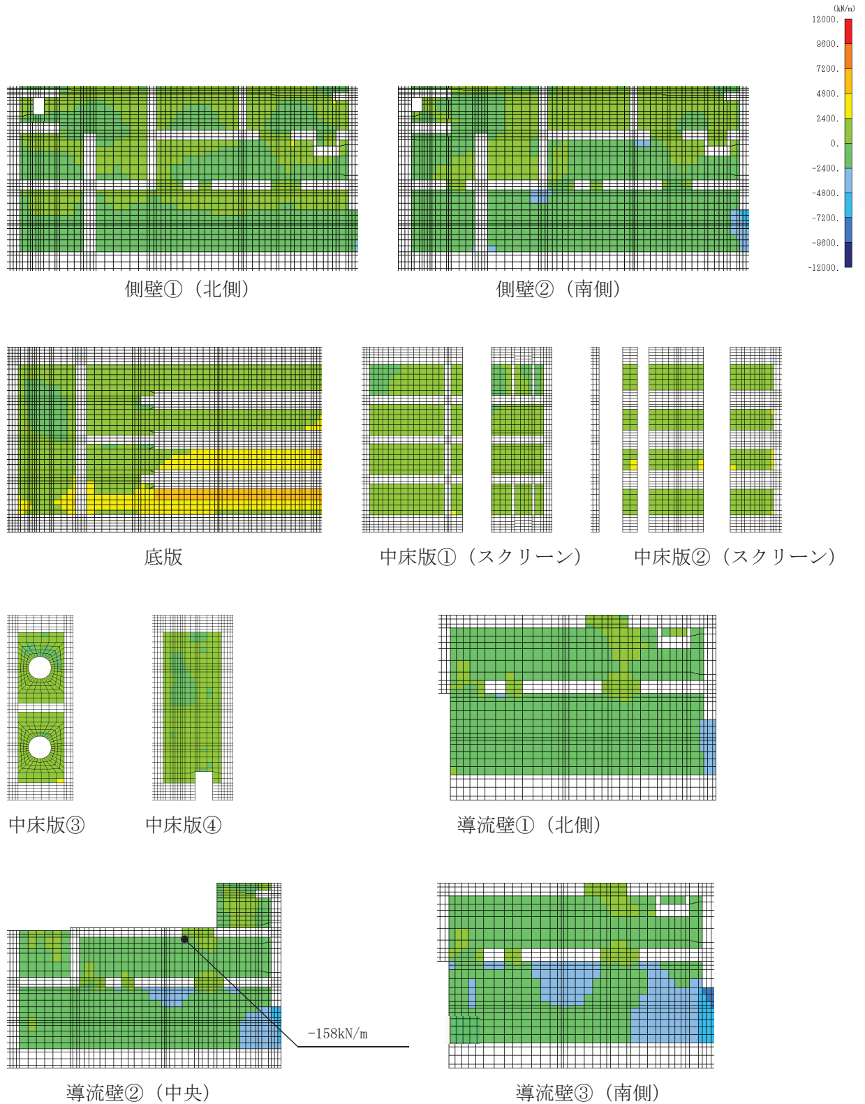
図 4-22(1) せん断破壊に対する照査値最大時の断面力分布図 (せん断力 (kN/m) : Q_y ) (導流壁②, 解析ケース⑧, S_s-D2 (++) )
