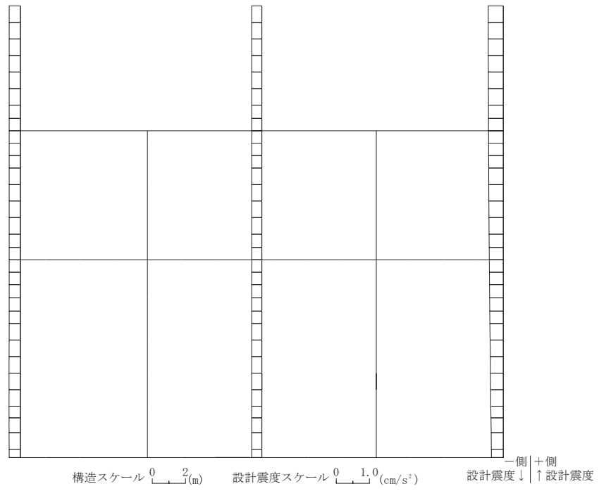
図 3-12(2) 作用荷重分布図 (設計震度分布)
