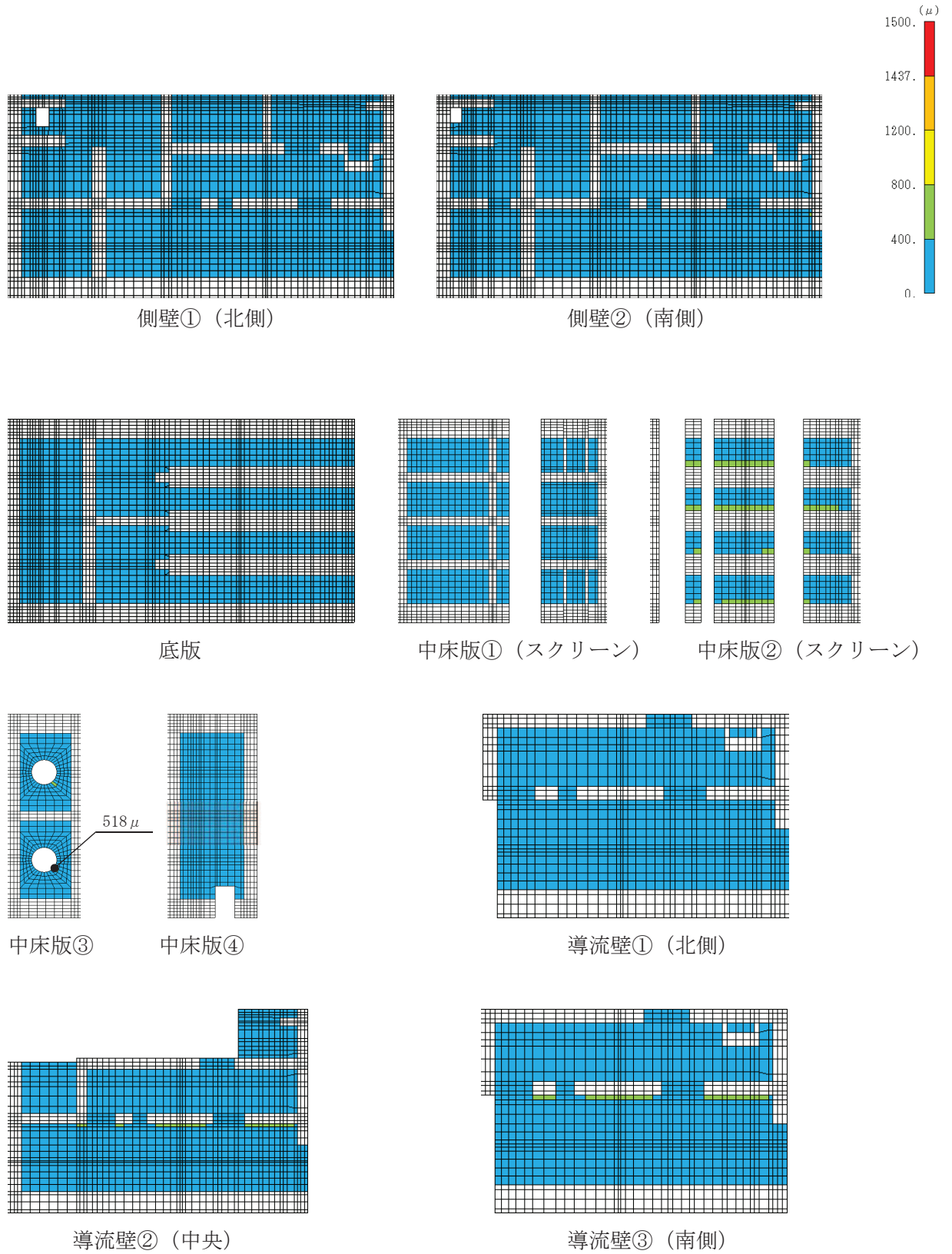
図 4-7(1) 曲げ・軸力系の破壊に対する照査値最大時のひずみ分布図 (鉄筋) (中床版③, 解析ケース①, S s - D 2 (++) )
