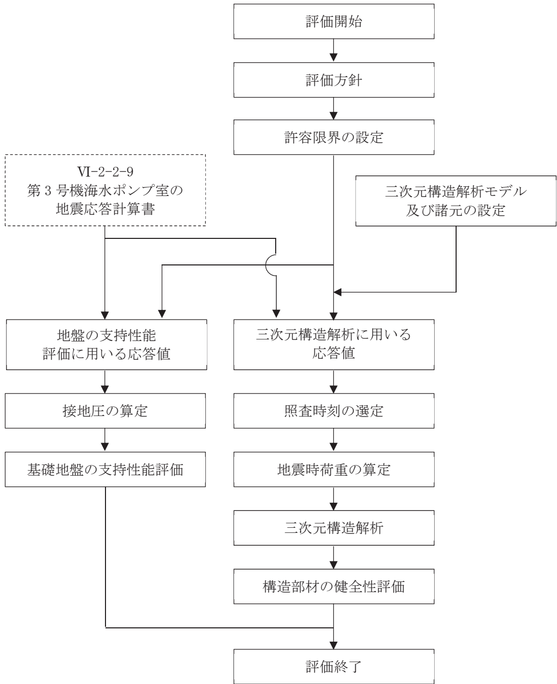
図 2-14 第 3 号機海水ポンプ室の耐震評価フロー
