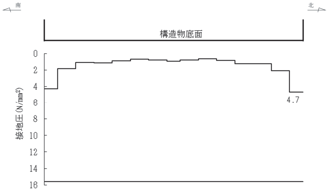
図 5-13 MMR (既設) の最大接地圧分布図
