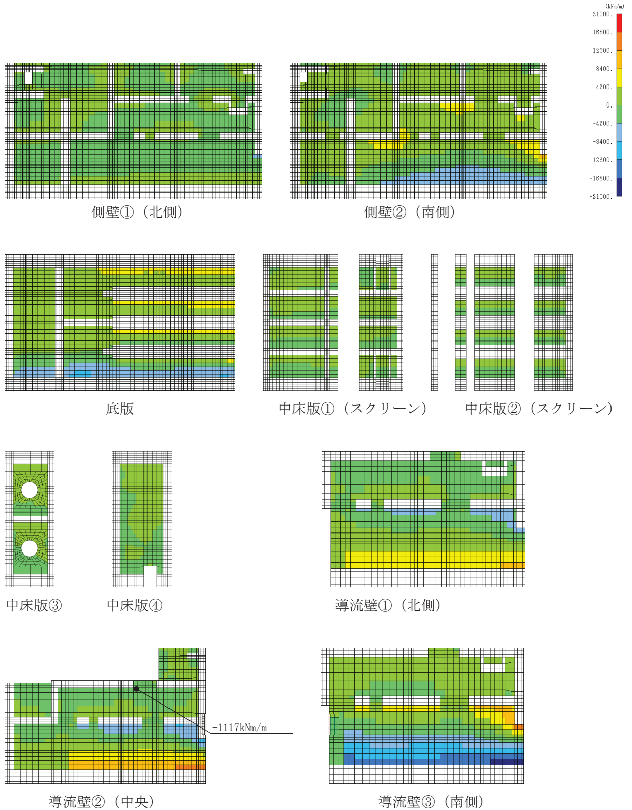
図 4-18(1) せん断破壊に対する照査値最大時の断面力分布図 (曲げモーメント (kN・m/m) : M_y ) (導流壁②, 解析ケース⑧, S s - D 2 (++) )
