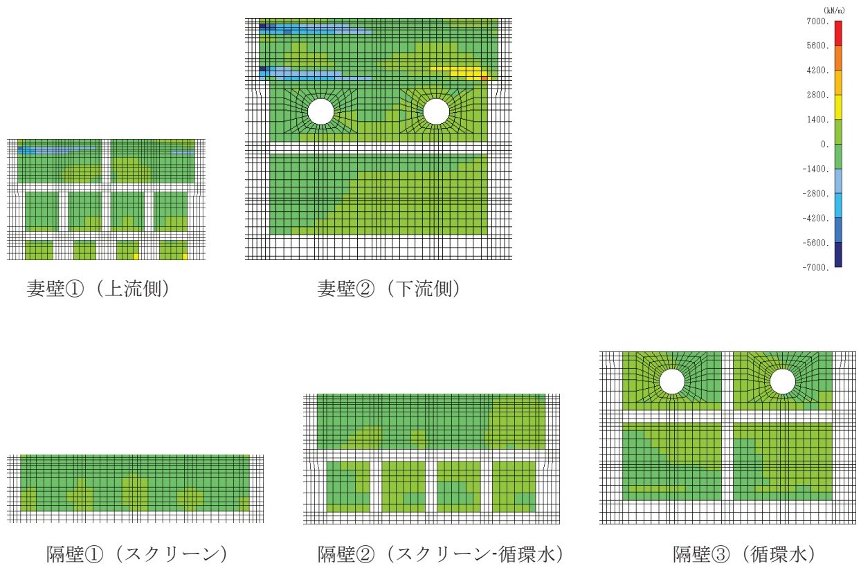
図 4-12(2) せん断破壊に対する照査値最大時の断面力分布図 (せん断力 (kN/m) : Q_x ) (導流壁①, 解析ケース④, S_s - N1 (++) )
