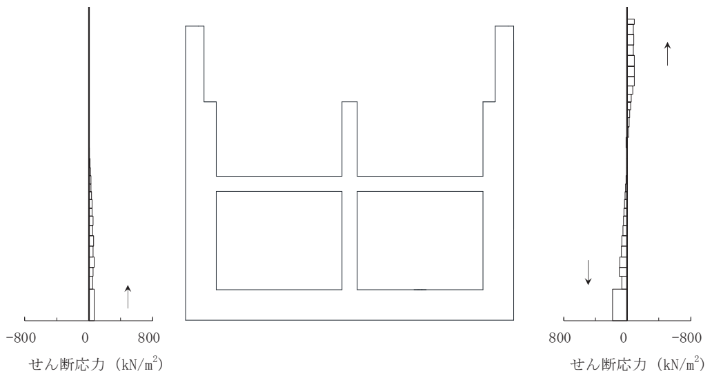
せん断応力
