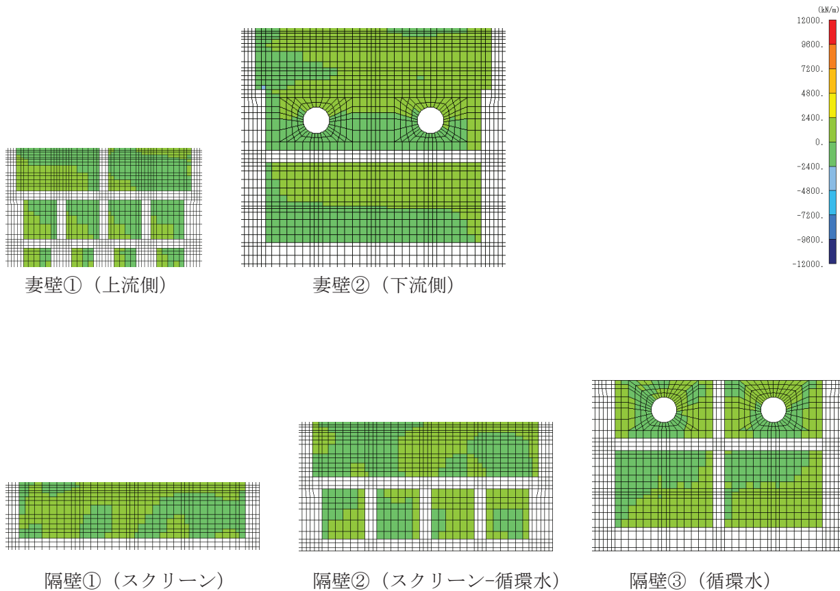
図 4-22(2) せん断破壊に対する照査値最大時の断面力分布図 (せん断力 (kN/m) : Q_y ) (導流壁②, 解析ケース⑧, S_s - D2 (++) )
