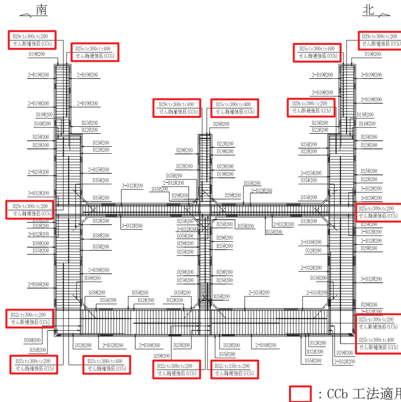
図 2-12 第 3 号機海水ポンプ室概略配筋図 (B-B 断面, 南北 (循環水ポンプエリア))
