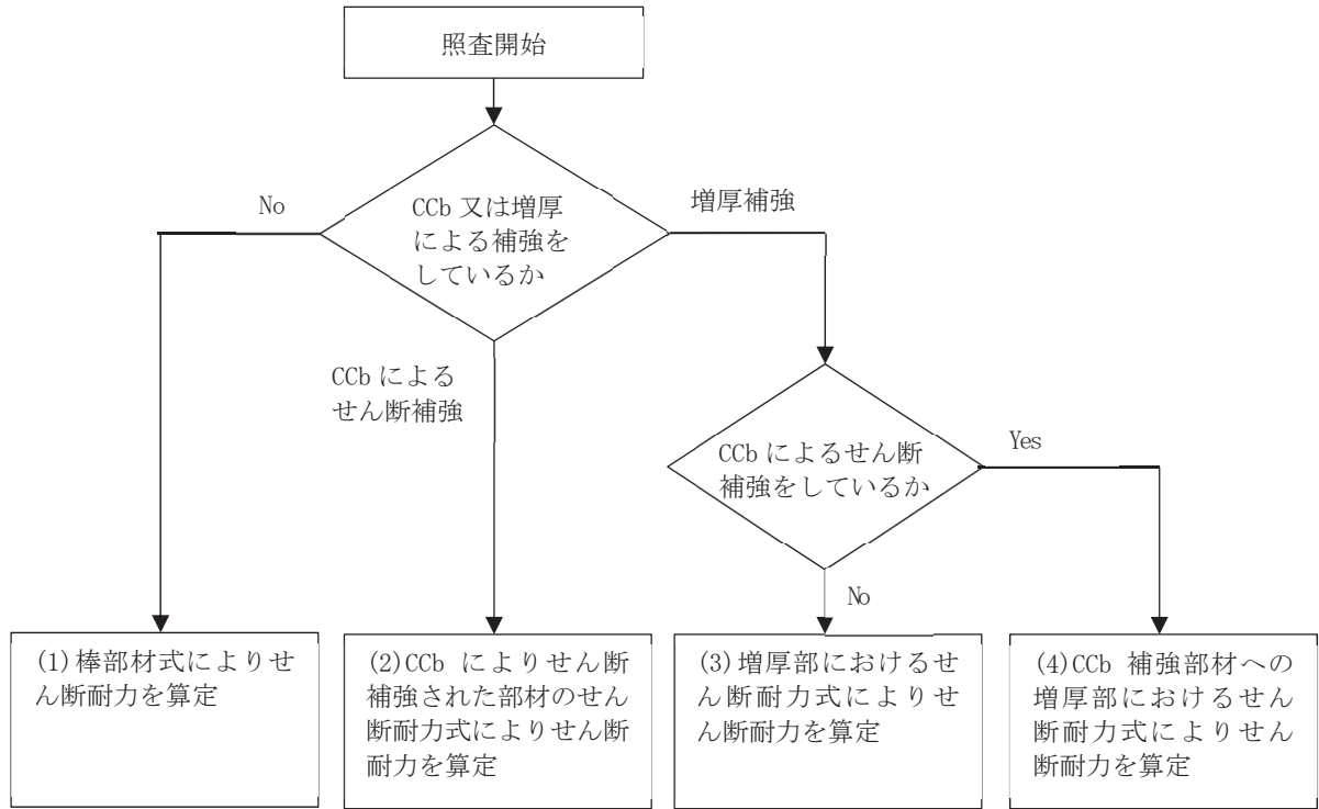
図 3-5 せん断破壊に対する耐力評価フロー
