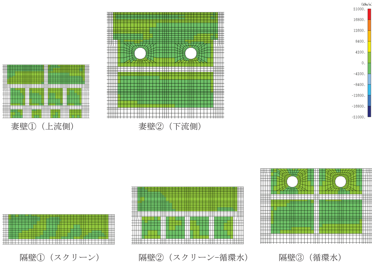
図 4-18(2) せん断破壊に対する照査値最大時の断面力分布図 (曲げモーメント (kN・m/m) : M_y ) (導流壁②, 解析ケース⑧, S s - D 2 (++) )
