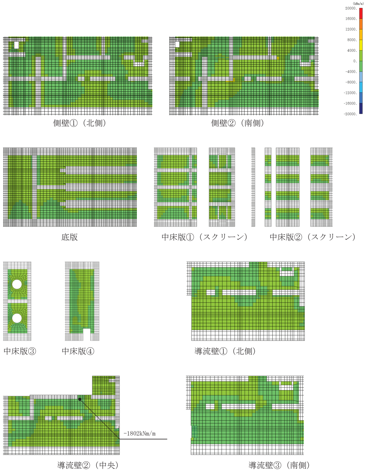
図 4-17(1) せん断破壊に対する照査値最大時の断面力分布図 (曲げモーメント (kN・m/m) : M_x ) (導流壁②, 解析ケース⑧, S s - D 2 (++) )
