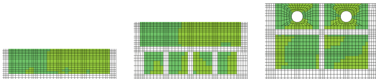
図 4-17(2) せん断破壊に対する照査値最大時の断面力分布図 (曲げモーメント (kN・m/m) : M_x ) (導流壁②, 解析ケース⑧, S_s - D2 (++) )
