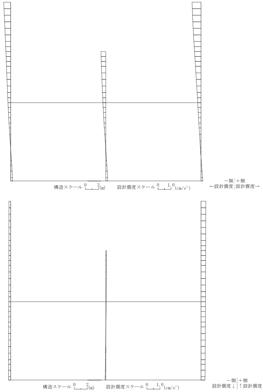
図 3-15(2) 作用荷重分布図 (設計震度分布) (解析ケース⑧, S s - D 2 (++) , B-B 断面, 南北 (循環水ポンプエリア))
