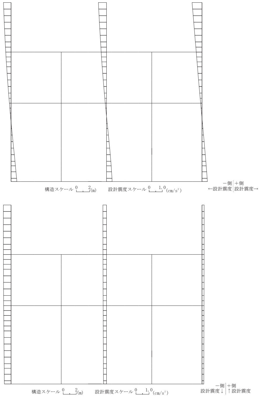
図 3-14(2) 作用荷重分布図 (設計震度分布) (解析ケース⑧, S s - D 2 (++) , A-A 断面, 南北 (スクリーンエリア))
