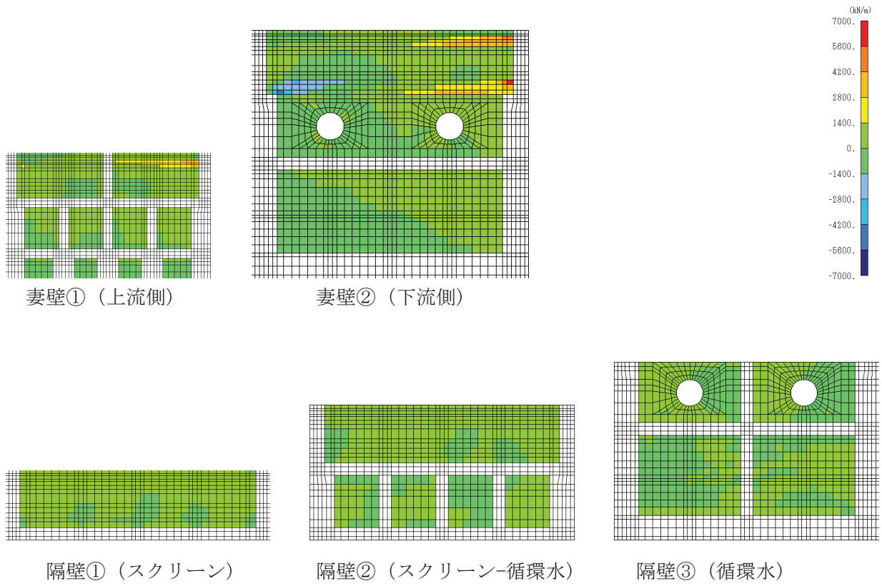
図 4-21 (2) せん断破壊に対する照査値最大時の断面力分布図 (せん断力 (kN/m) : Q_x ) (導流壁②, 解析ケース⑧, S_s - D2 (++) )
