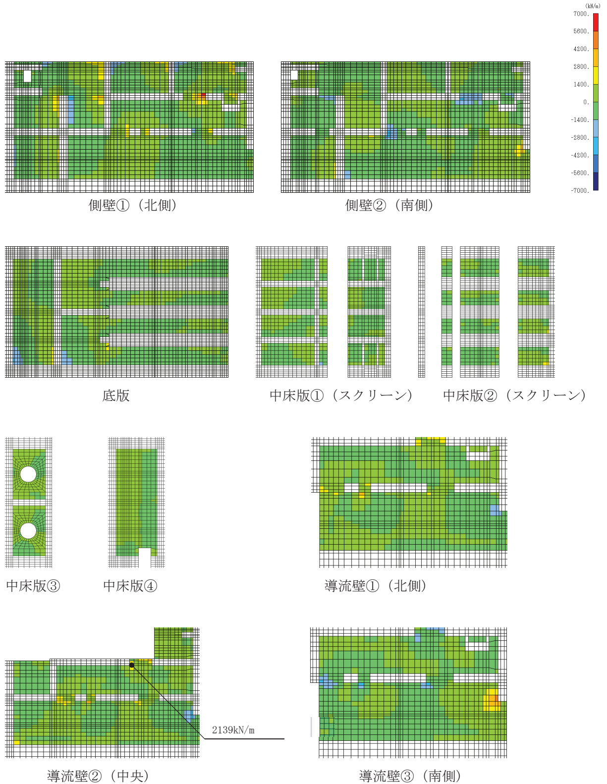
図 4-21(1) せん断破壊に対する照査値最大時の断面力分布図 (せん断力 (kN/m) : Q_x ) (導流壁②, 解析ケース⑧, S_s-D2 (++))
