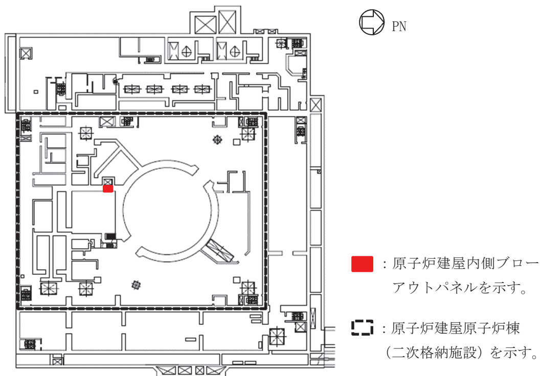
原子炉建屋原子炉棟地下1階 概略平面図 (O.P. 6.00m)
