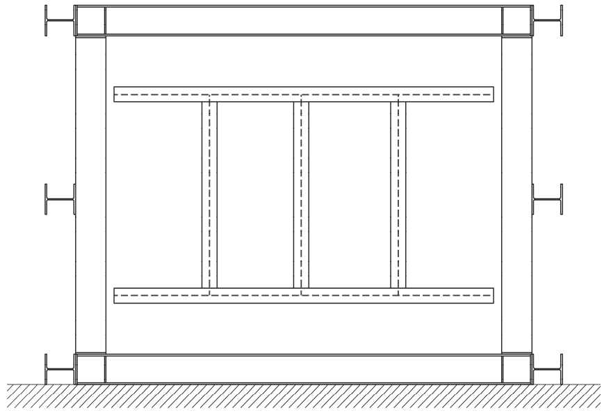
パネル及び押し出し梁図
