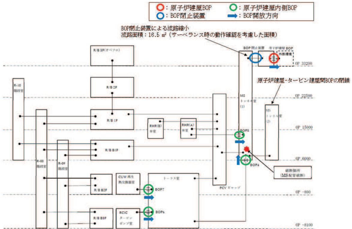
図 2-1 解析モデル
