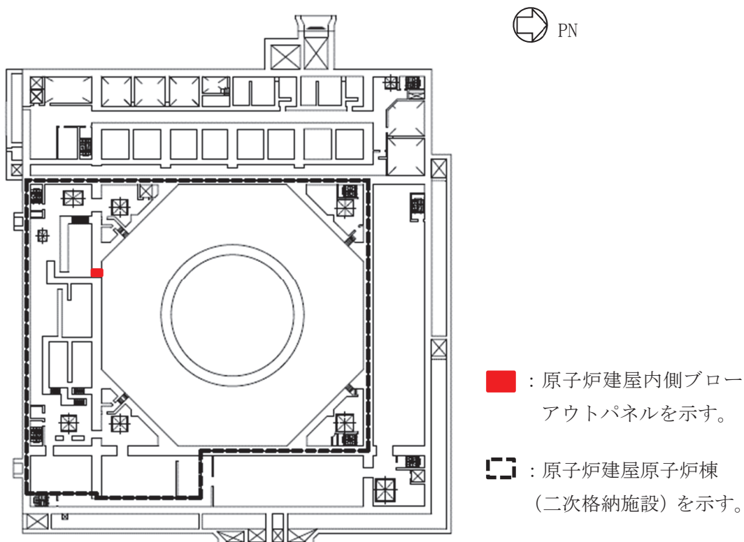
原子炉建屋原子炉棟地下2階 概略平面図 (O.P. -0.80m)
