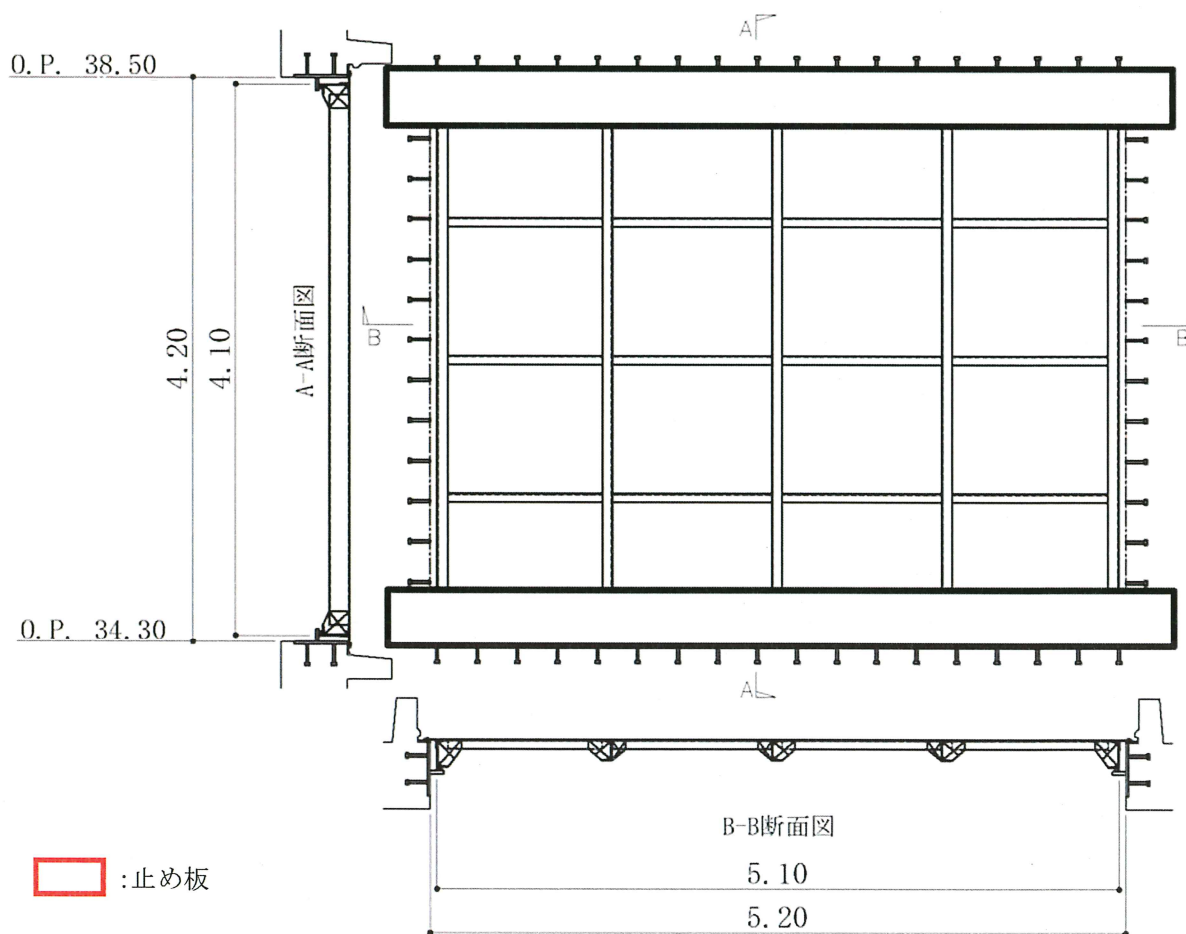
図 4-4 止め板配置図 (立面図)
