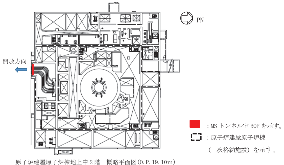
図 3-1 MS トンネル室 BOP 配置図 (閉鎖)
