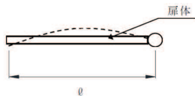
図 3-2 固有値計算モデル（扉開放時）
