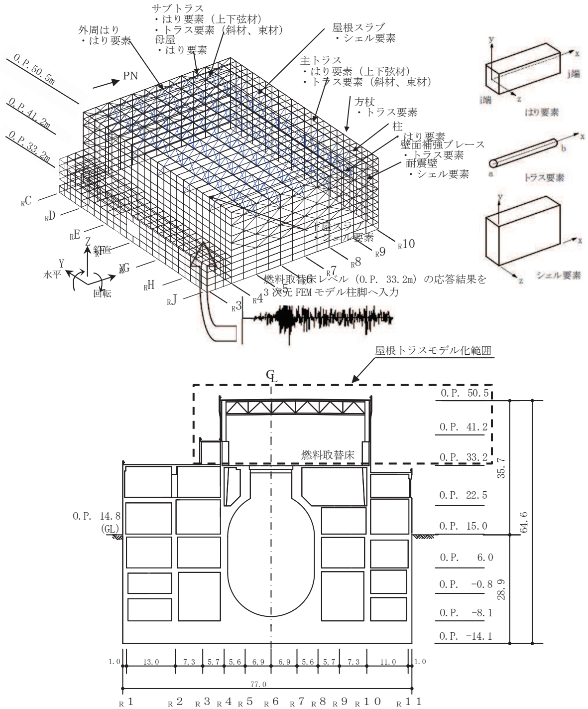
図 4-15 屋根トラス (燃料取替床上部フレーム) の解析モデル図と入力概要
