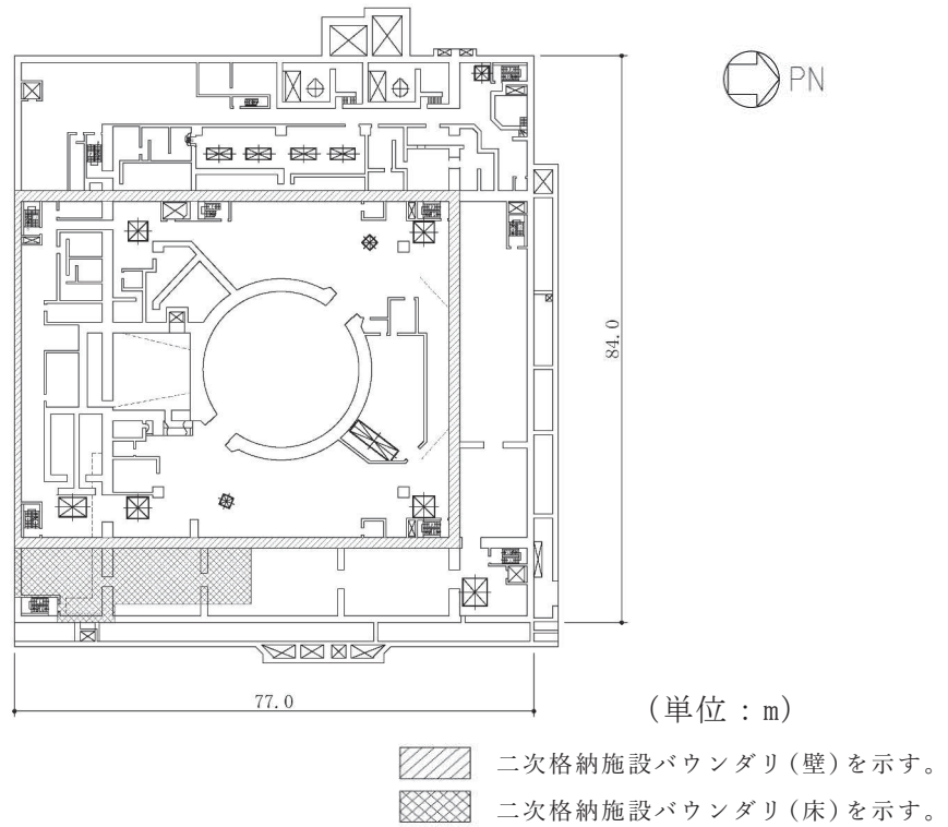
図 2-2(3) 原子炉建屋原子炉棟（二次格納施設）の範囲の平面図 (B1F, O.P. 6.0m)
