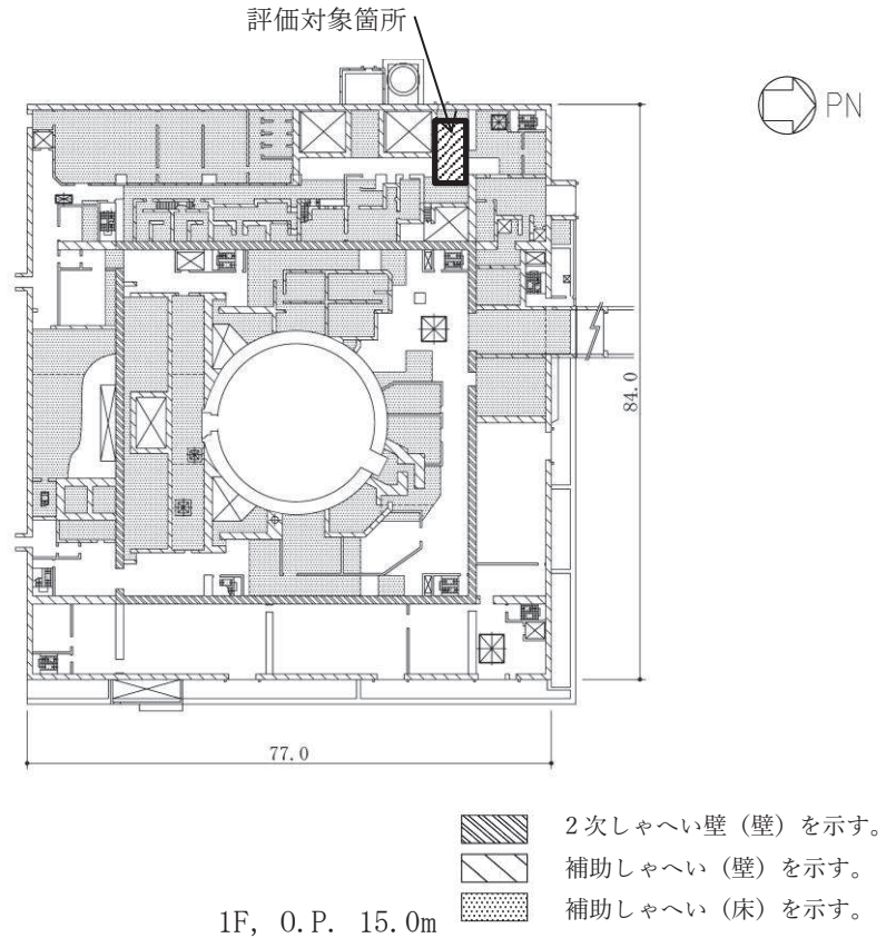
図 6-2 評価対象箇所（床スラブ）
