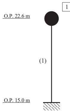
図 3-3 地震応答解析モデル (UD 方向)
