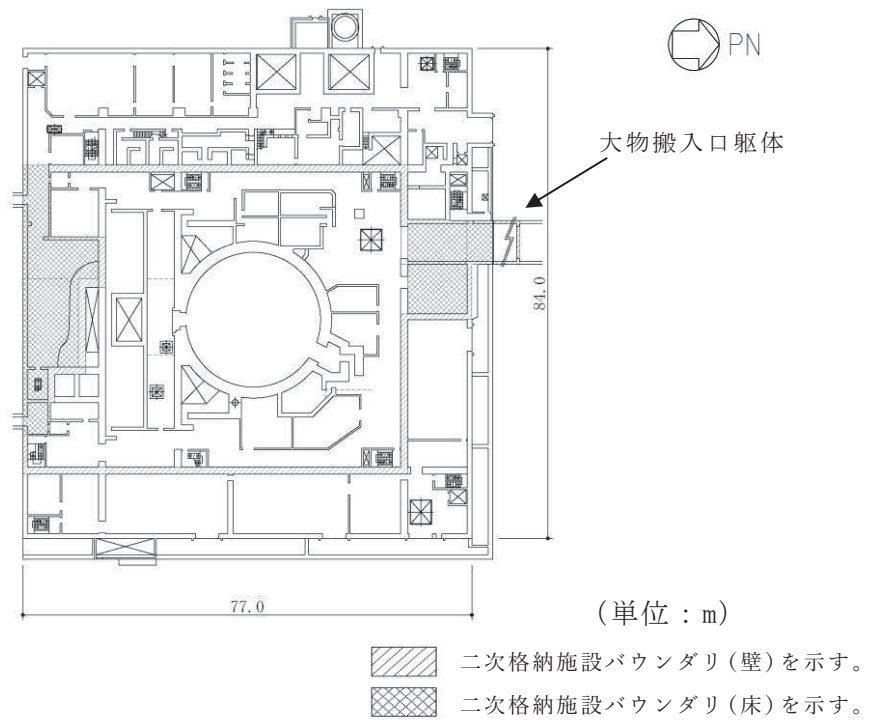
図 2-2(4) 原子炉建屋原子炉棟（二次格納施設）の範囲の平面図 (1F, O.P. 15.0m)
