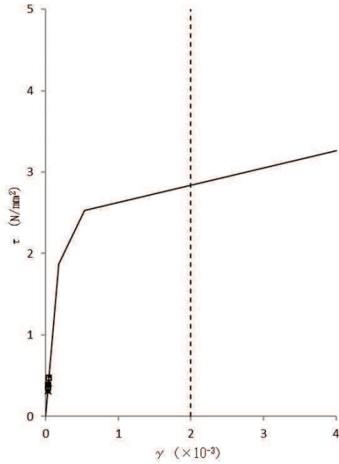
図 4-14 せん断スケルトンカーブ上の最大応答値 (基準地震動 S s , NS 方向)
