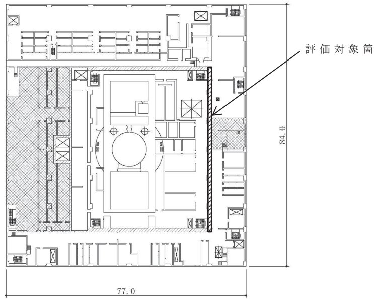
図 4-4 耐震壁の評価を記載する部材の位置 (2F, O.P. 22.5m)
