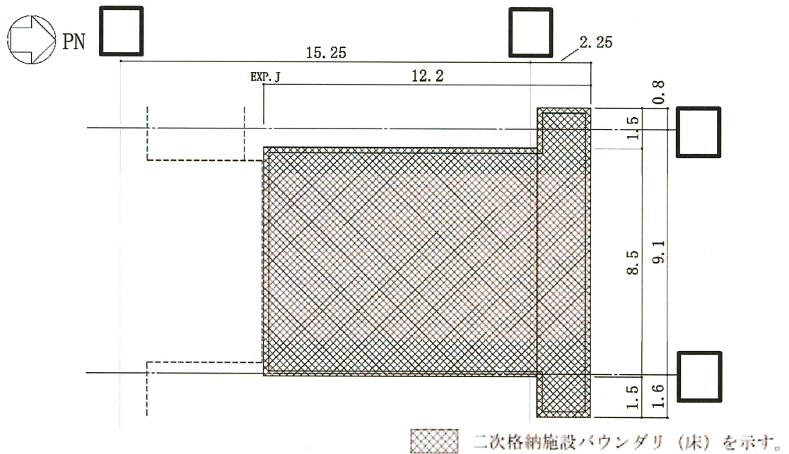
図 2-5(1) 原子炉建屋原子炉棟（二次格納施設）の範囲の平面図 (1F, O.P. 15.0m) (1/2)
