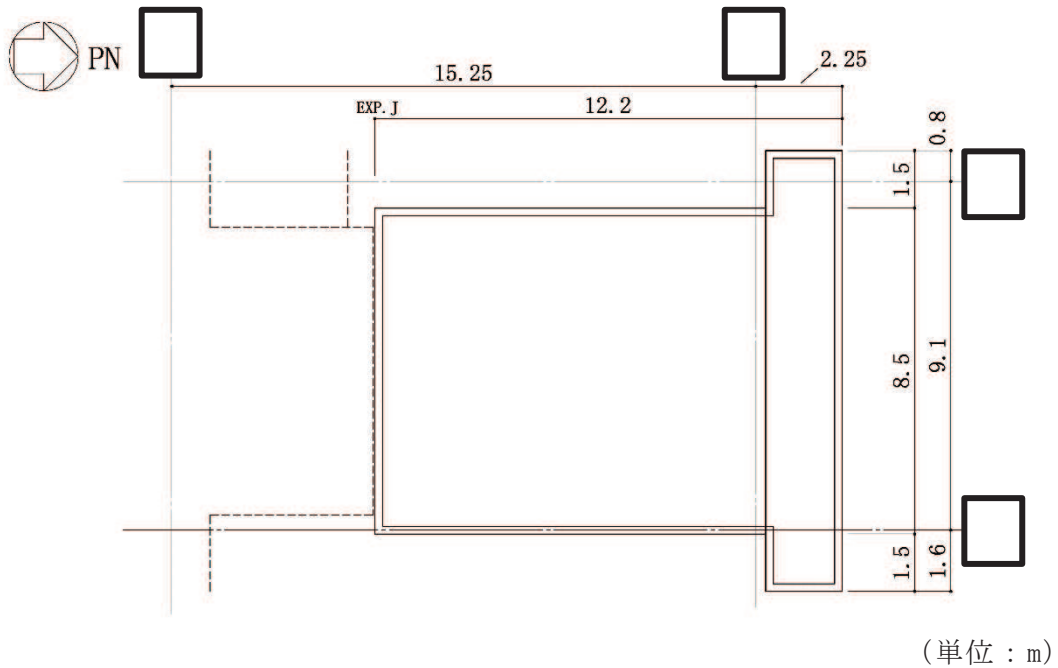
図 2-7(2) 2次しゃへい壁の範囲の平面図 (RF, 0.P. 22.6m)
