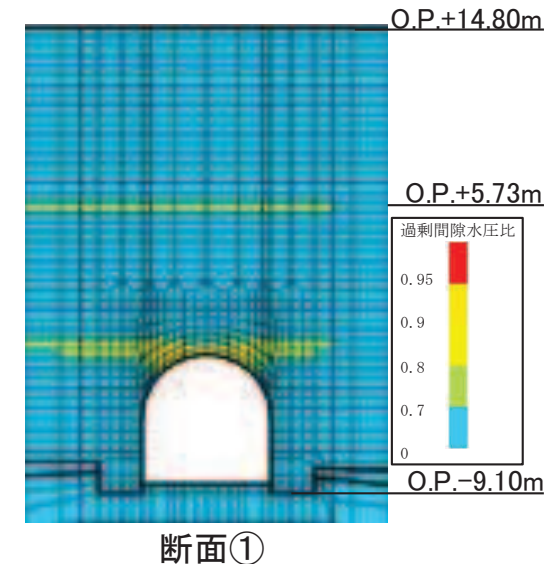
断面① 最大過剰間隙水圧比分布図
