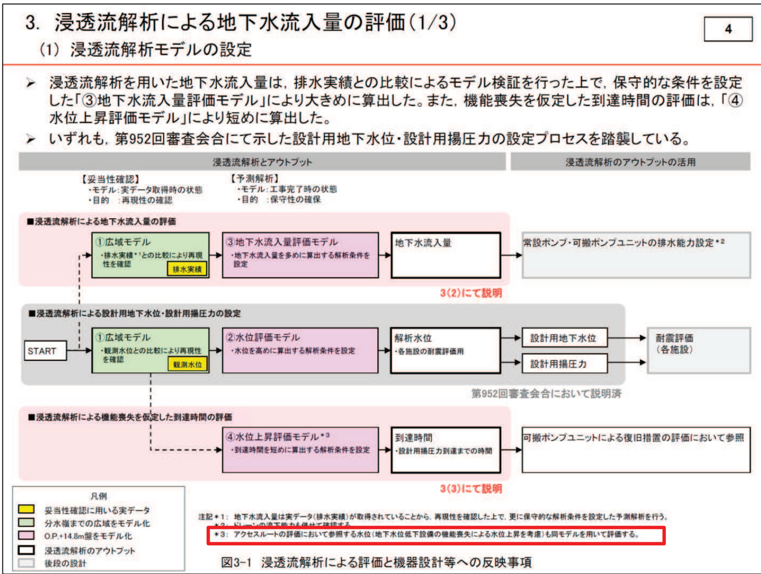
屋外アクセスルート評価において参照する浸透流解析モデル(第988回審査会合資料 一部加筆)
