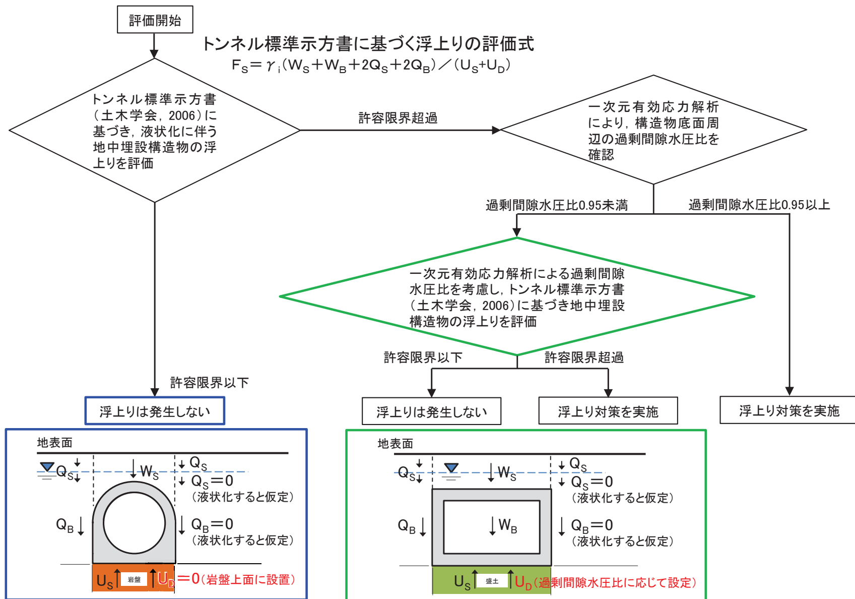
浮上り評価の概念図(排気筒連絡ダクト)
