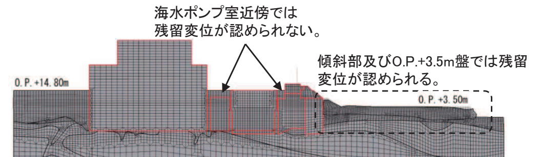
B-B断面の残留変形図(Ss-D1(++), 変形倍率2倍)
