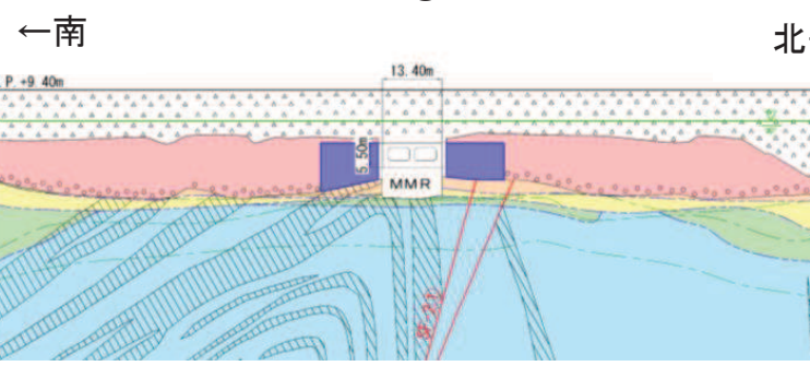
断面③
