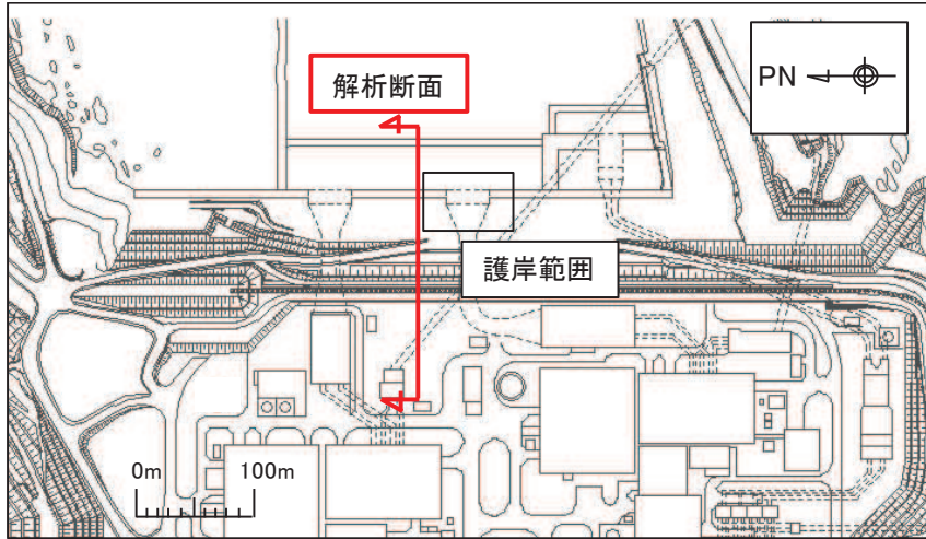
平面図*1
