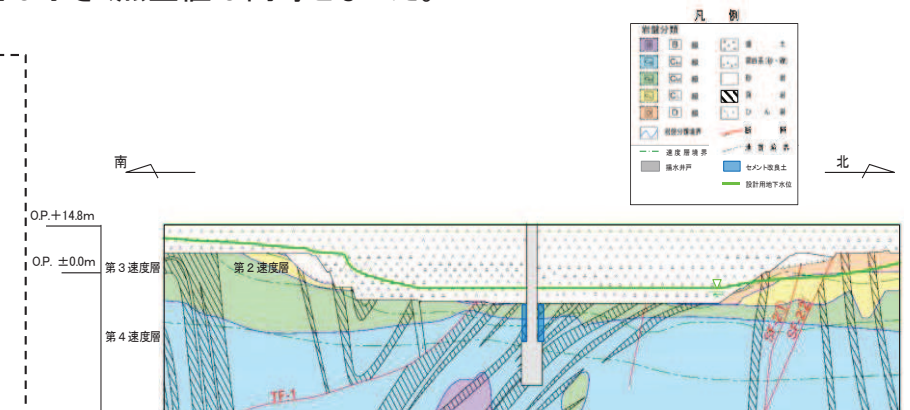
No.2揚水井戸地質断面図
