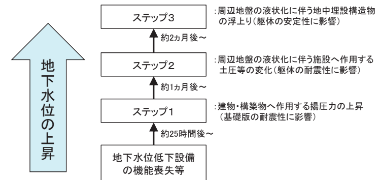
地下水位上昇時に施設に段階的に生じる影響(時間軸) (第98回審査会合(令和3年7月6日)資料 一部加筆)
