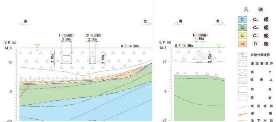
A-A' 断面
