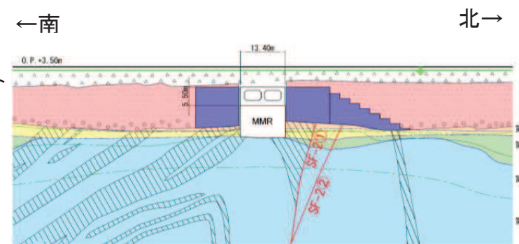
断面②
