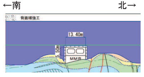
断面⑤
