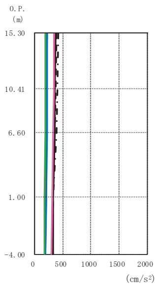
図 4-17 最大応答加速度 (弾性設計用地震動 S d (++) , ケース①, NS 断面)
