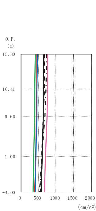
図 4-3 最大応答加速度 (基準地震動 S s (++) , ケース②, NS 断面)
