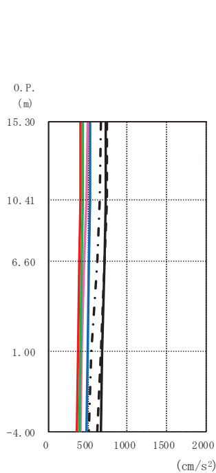
図 4-13 最大応答加速度 (基準地震動 S s (++) , ケース③, EW 断面)
