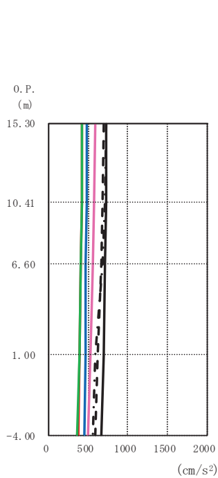
図 4-9 最大応答加速度 (基準地震動 S s (++) , ケース①, EW 断面)
