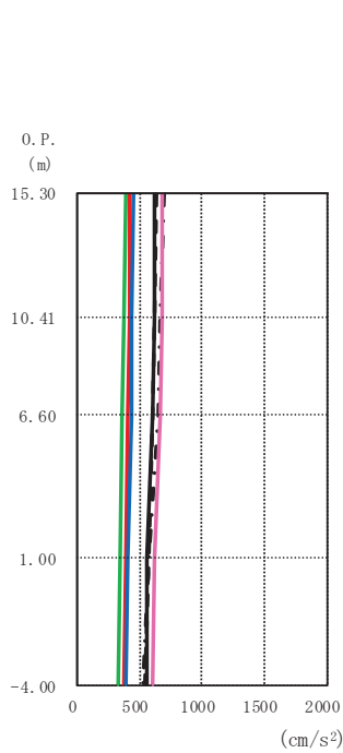
図 4-7 最大応答加速度 (基準地震動 S s (++), ケース④, NS 断面)
