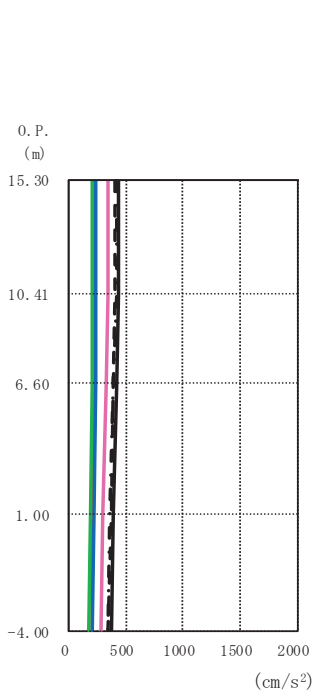
図 4-27 最大応答加速度 (弾性設計用地震動 S d (++) , ケース②, EW 断面)
