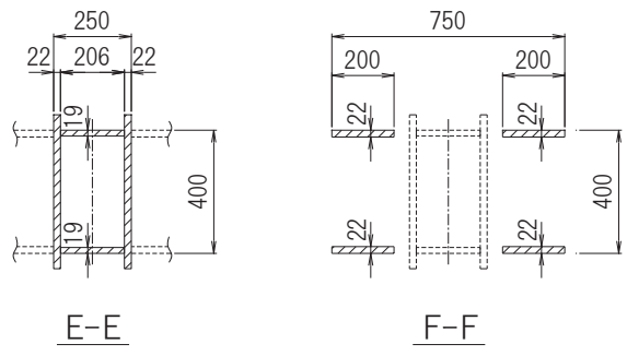
図 2-3(4) 筒身連結材の構成断面
