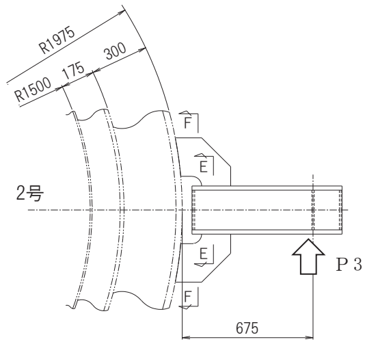
筒身連結材詳細
