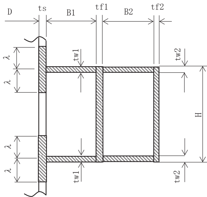
C-C 断面
