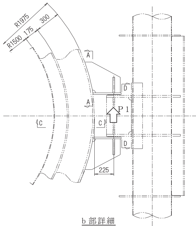
図 2-2(2) 第 2 支持点部の支持金物の平面図及び支持点荷重
