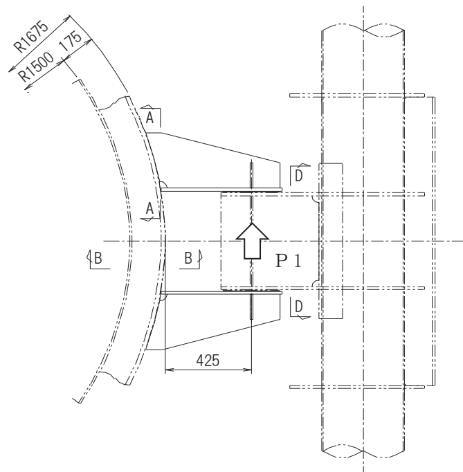
a 部詳細
