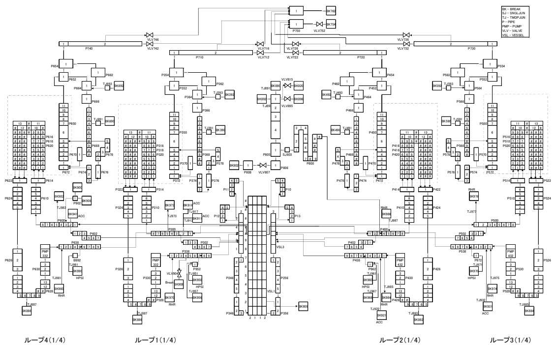
図 2 PKL を模擬するコンポーネント構成の例
