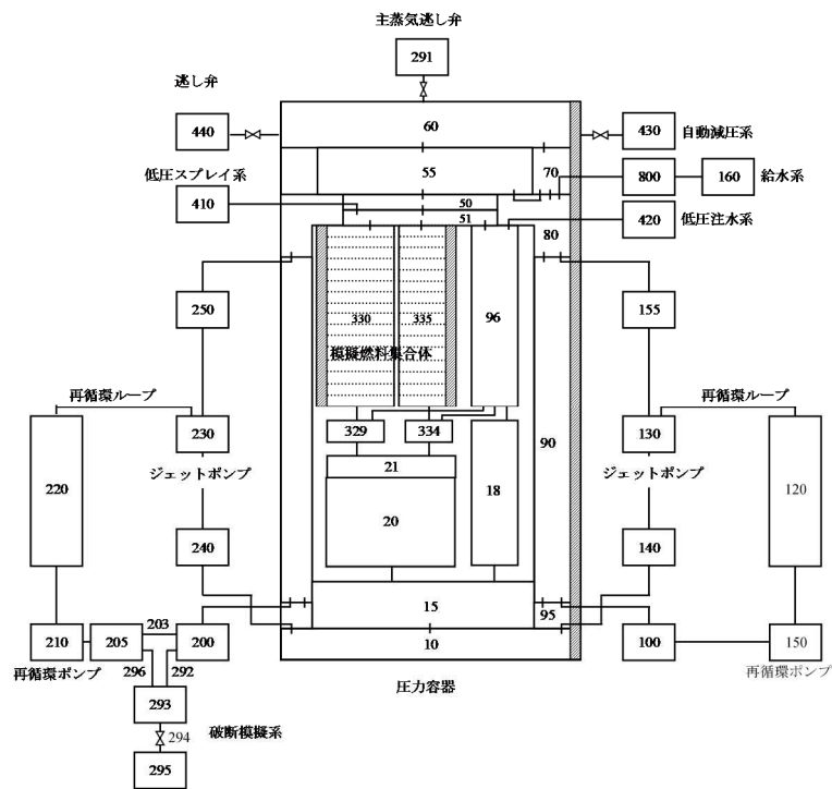
図 1 ROSA-III を模擬するコンポーネント構成の例
