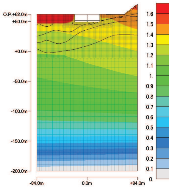
最大変位分布 (最大値: 8.8681cm)
