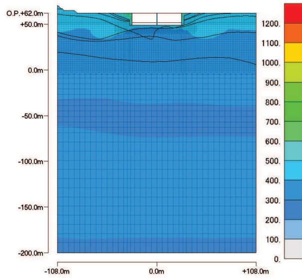
最大加速度分布 (最大値:922.55 cm/s 2 )
