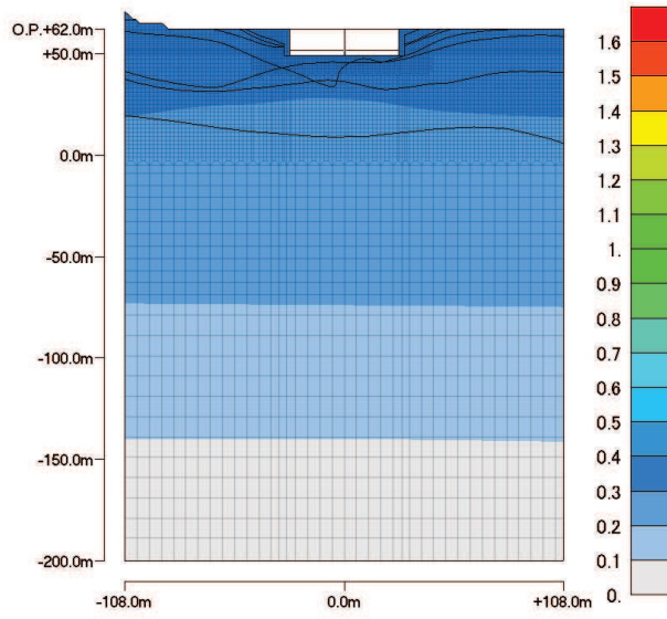
最大変位分布 (最大値:0.3321cm)
