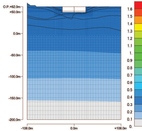
最大変位分布 (最大値:0.4103cm)
