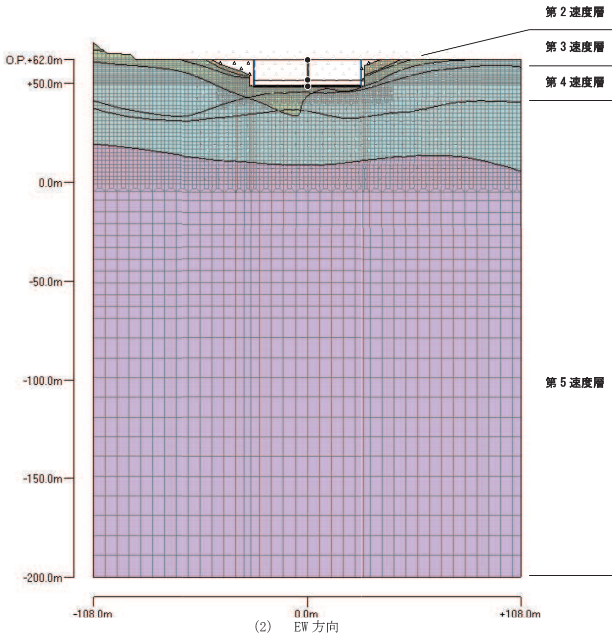
図 2-9 (2) 二次元 FEM 地盤モデル及び地盤の物性値
