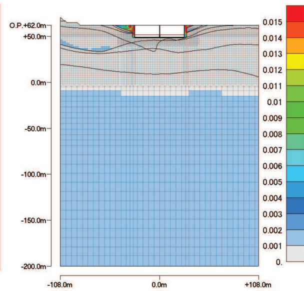
最大ひずみ分布 (最大値:0.03374%)
