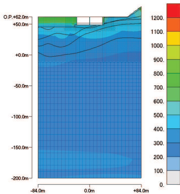
最大加速度分布 (最大値:1188.4 cm/s 2 )
