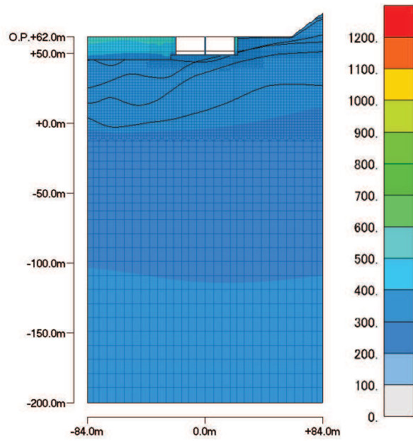
最大加速度分布 (最大値:713.4 cm/s 2 )
