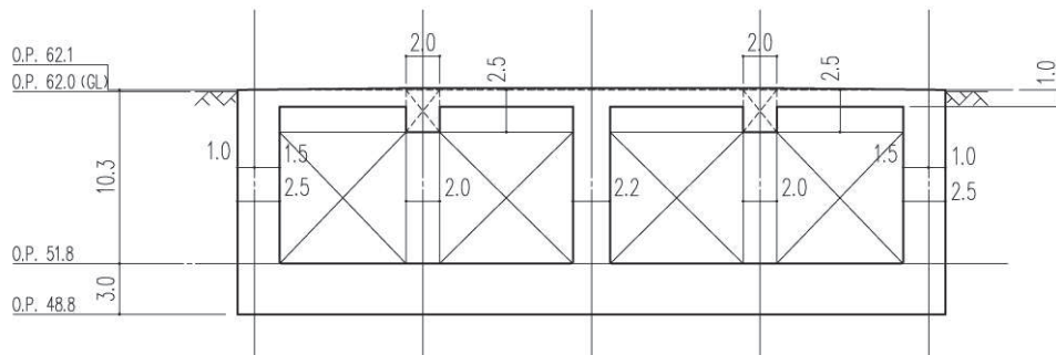
図 2-3 (2) 淡水貯水槽の概略断面図 (B-B 断面 NS 方向)
