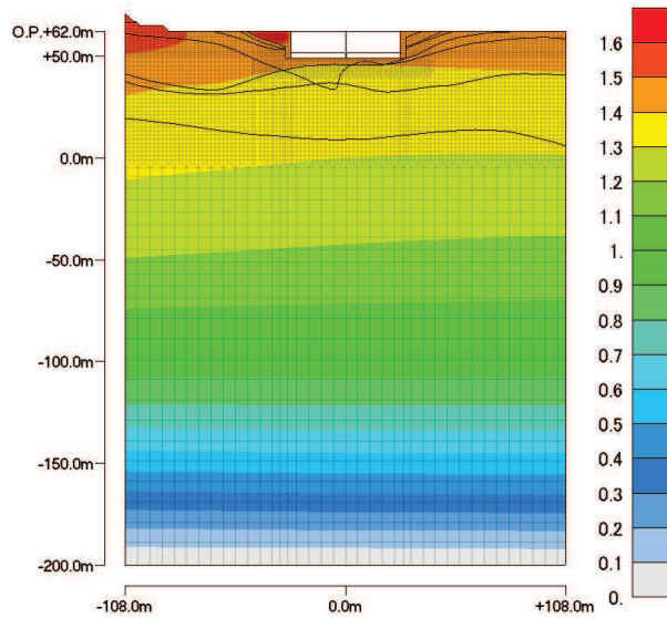
最大変位分布 (最大値:2.27521cm)
