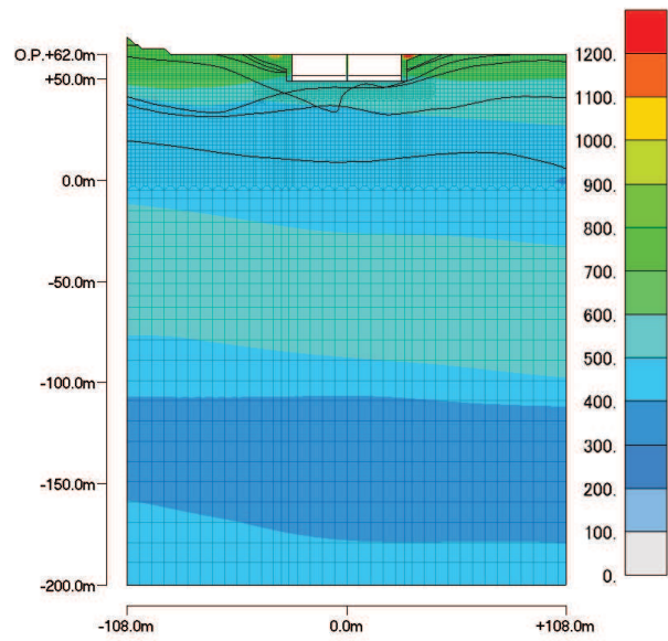
最大加速度分布 (最大値:1390.5 \text{cm/s}^2 )
