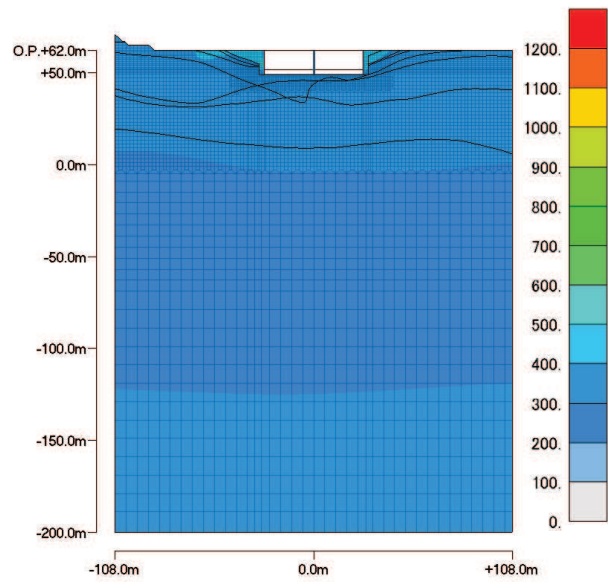
最大加速度分布 (最大値:613.17 cm/s 2 )
