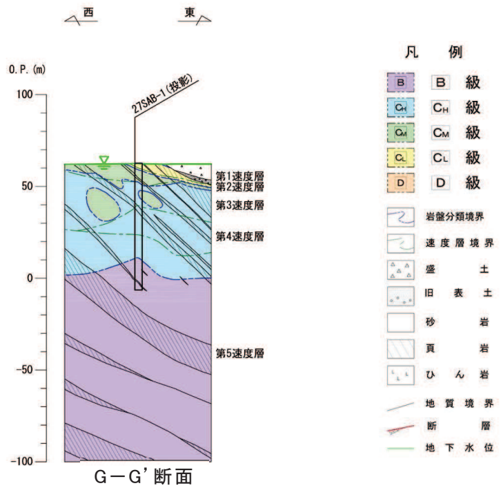
図 2.3.3-6 緊急時対策建屋北側の地質断面図
