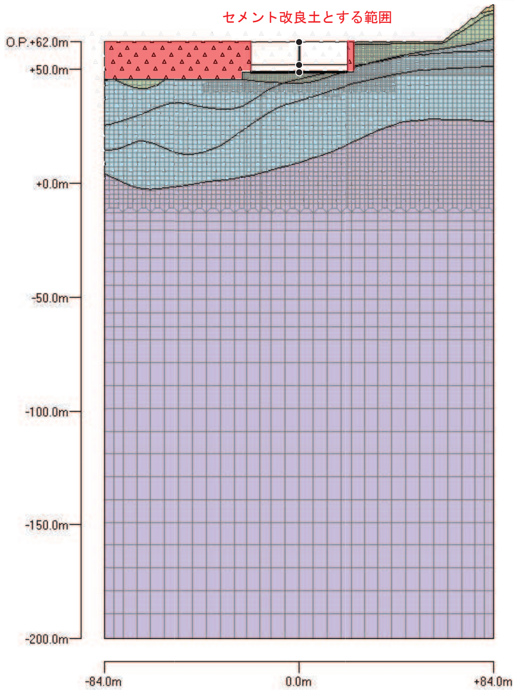
図 3-1 (1) 第 2 保管エリアの地震応答解析モデル (二次元)
