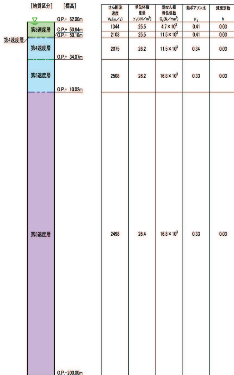
図 2.3.3-11(2) 第4保管エリア②の地震応答解析モデル(一次元)
