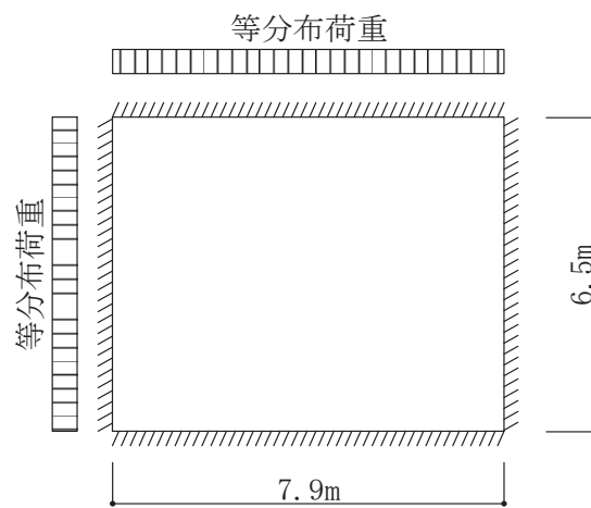
図 2-13 頂版の解析モデル
