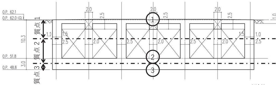
図 2-8 (2) 淡水貯水槽の概略断面図 (EW 方向)
