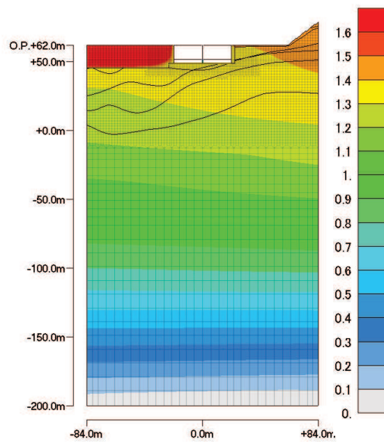
最大変位分布 (最大値:7.705cm)
