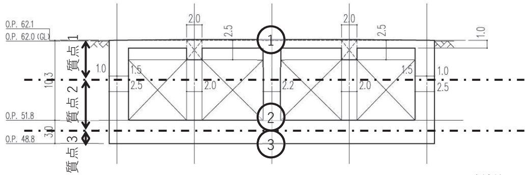
図 2-8 (1) 淡水貯水槽の概略断面図 (NS 方向)
