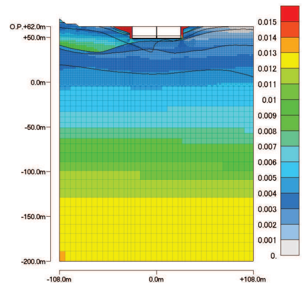
最大ひずみ分布 (最大値:0.2978%)
