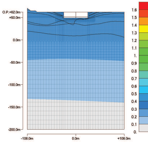
最大変位分布 (最大値:0.3252cm)
