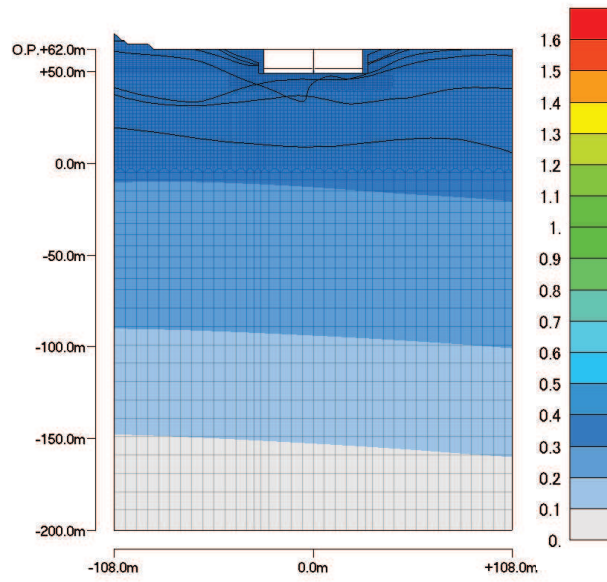
最大変位分布 (最大値:0.3637cm)
