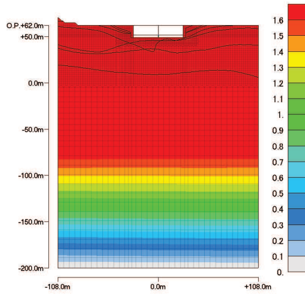
最大変位分布 (最大値: 3.0602cm)
