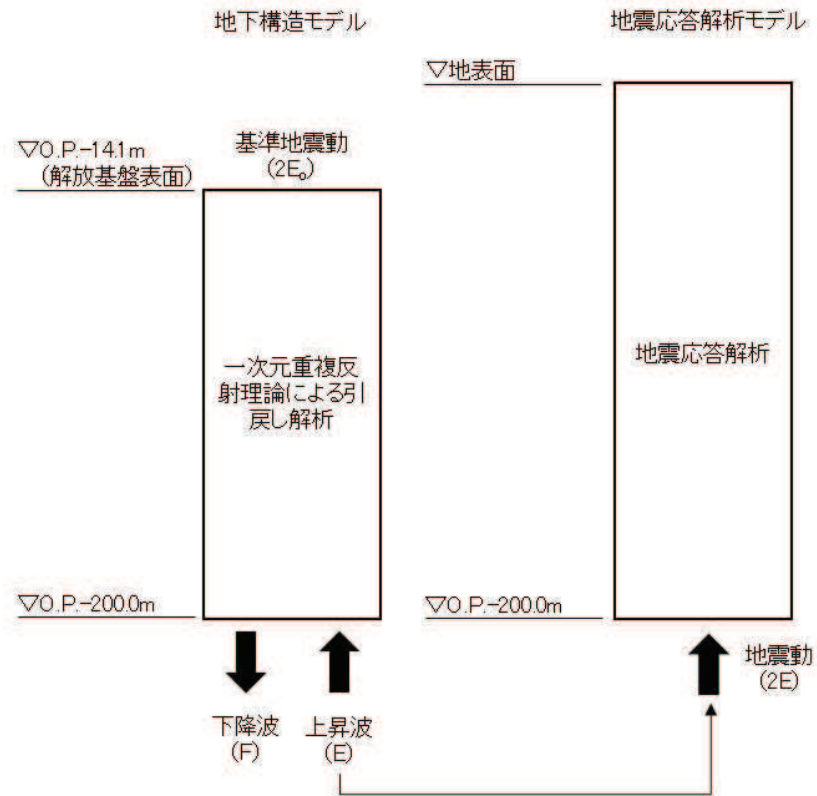
図 2.3.4-1 地震応答解析に用いる地震動算定の概念図
