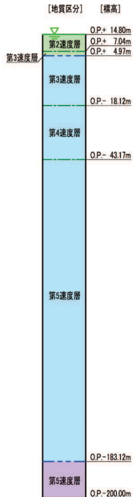
図 2.3.3-10(1) 第3保管エリア①の地震応答解析モデル(一次元)
