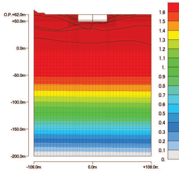
最大変位分布 (最大値:2.6121cm)
