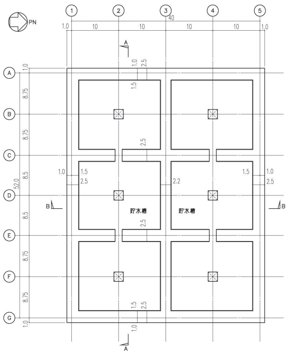
図 2-2 淡水貯水槽の概略平面図 (O.P. 51.8m)
