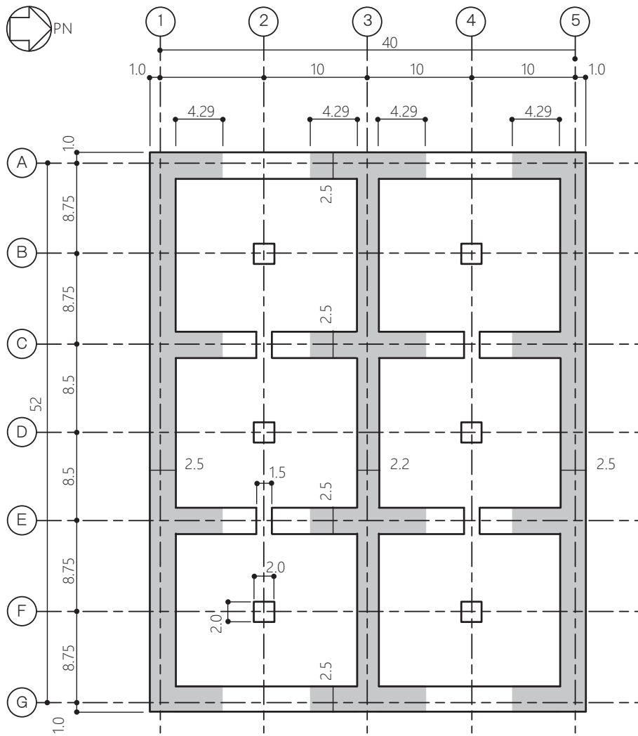
図 2-6 耐震壁の剛性評価範囲 (EW 方向)
