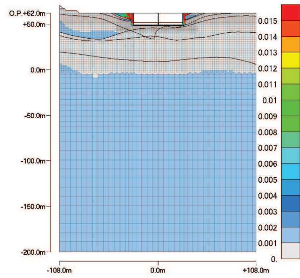
最大ひずみ分布 (最大値:0.03716%)
