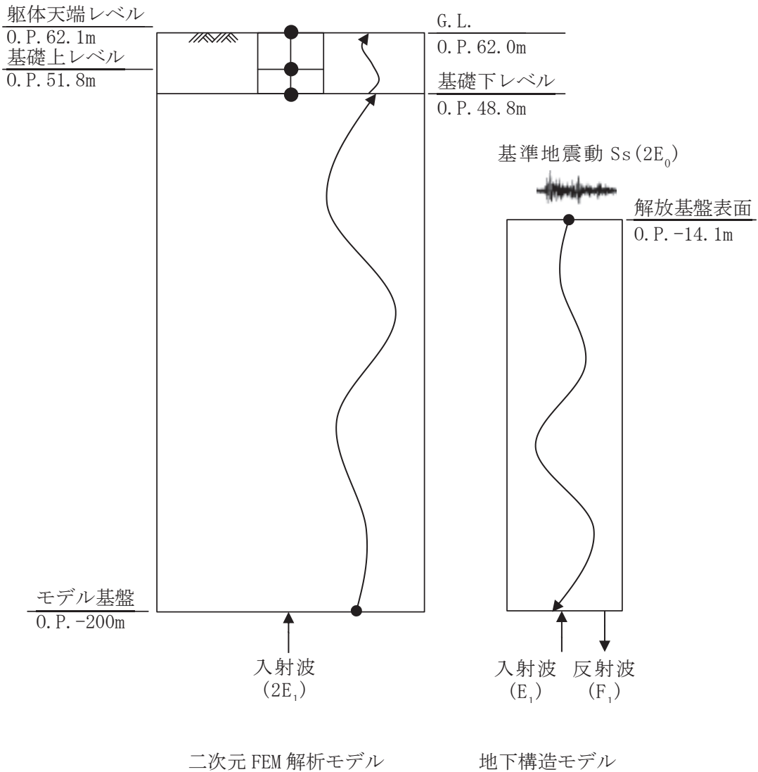
図 2-12 地震応答解析モデルに入力する地震動の概念図
