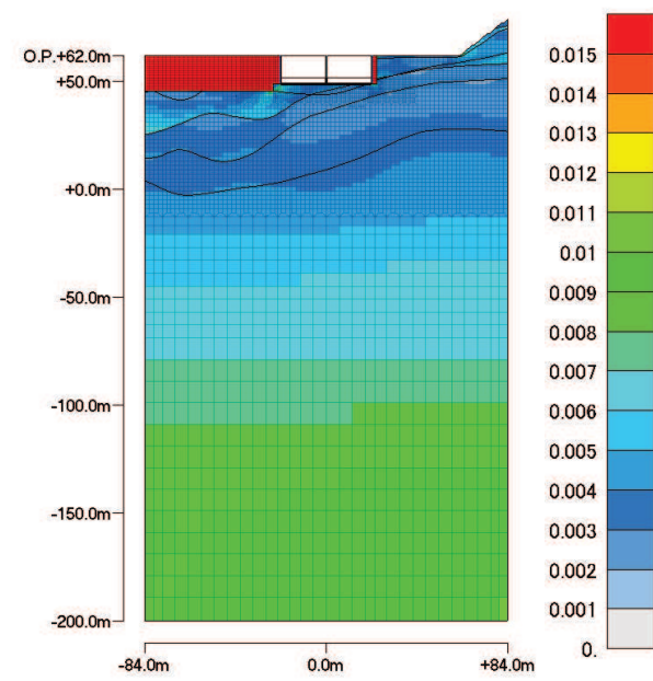
最大ひずみ分布 (最大値:0.7476%)
