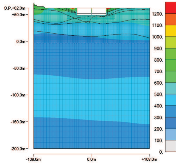
最大加速度分布 (最大値:2018.7 \text{cm/s}^2 )
