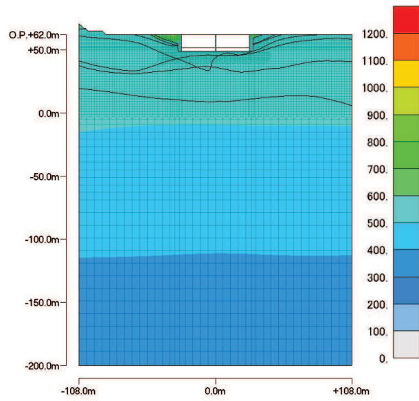
最大加速度分布 (最大値: 908.06 cm/s 2 )
