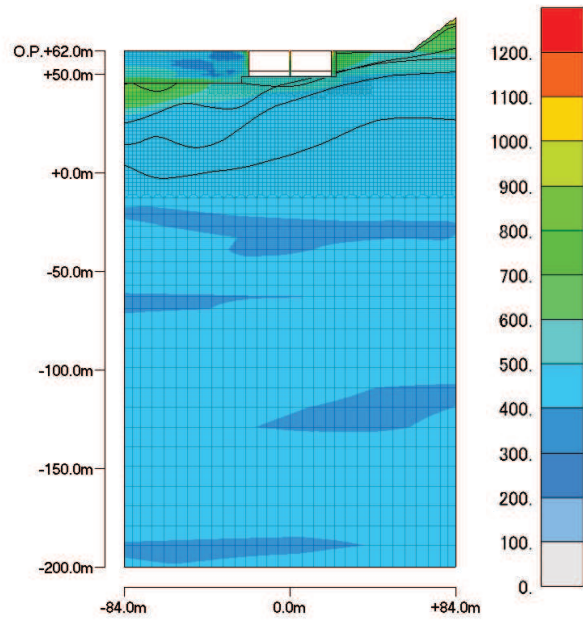
最大加速度分布 (最大値:1149.4 \text{cm/s}^2 )
