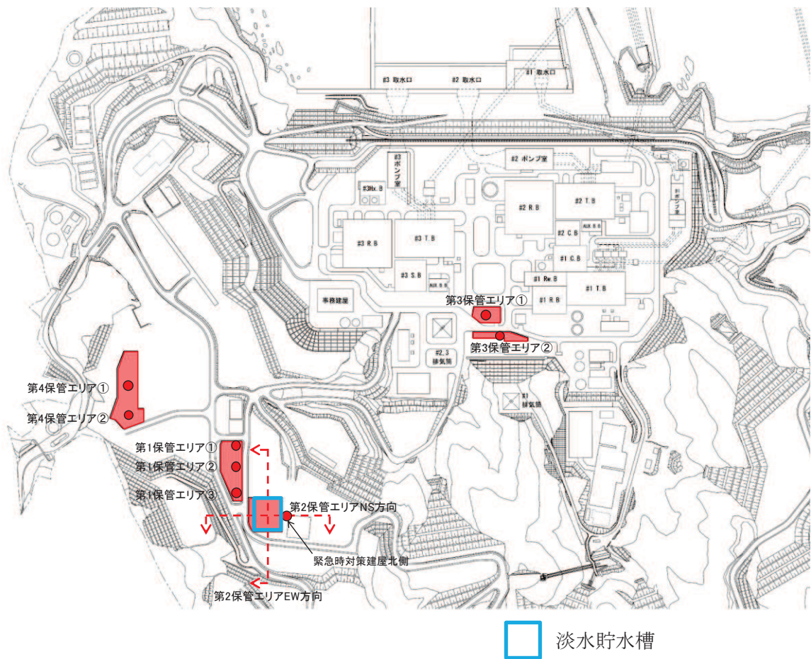
図2-1 淡水貯水槽の設置位置
