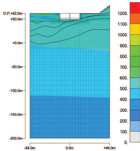
最大加速度分布 (最大値:779.97 cm/s 2 )
