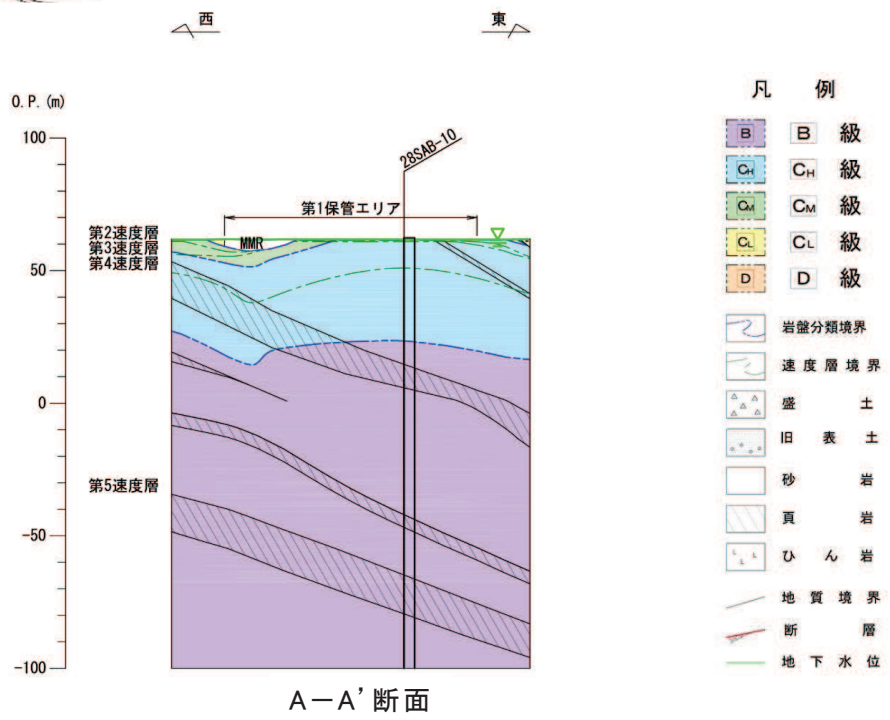
図 2.3.3-2 第1保管エリアの地質断面図
