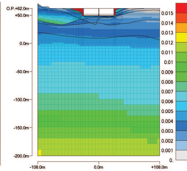
最大ひずみ分布 (最大値:0.3949%)
