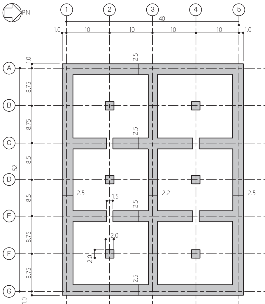
図 2-7 耐震壁の剛性評価範囲 (UD 方向)
