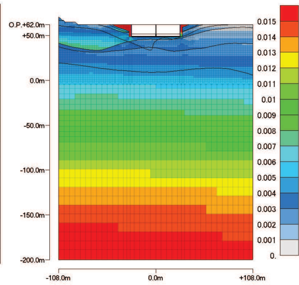
最大ひずみ分布 (最大値: 0.286%)
