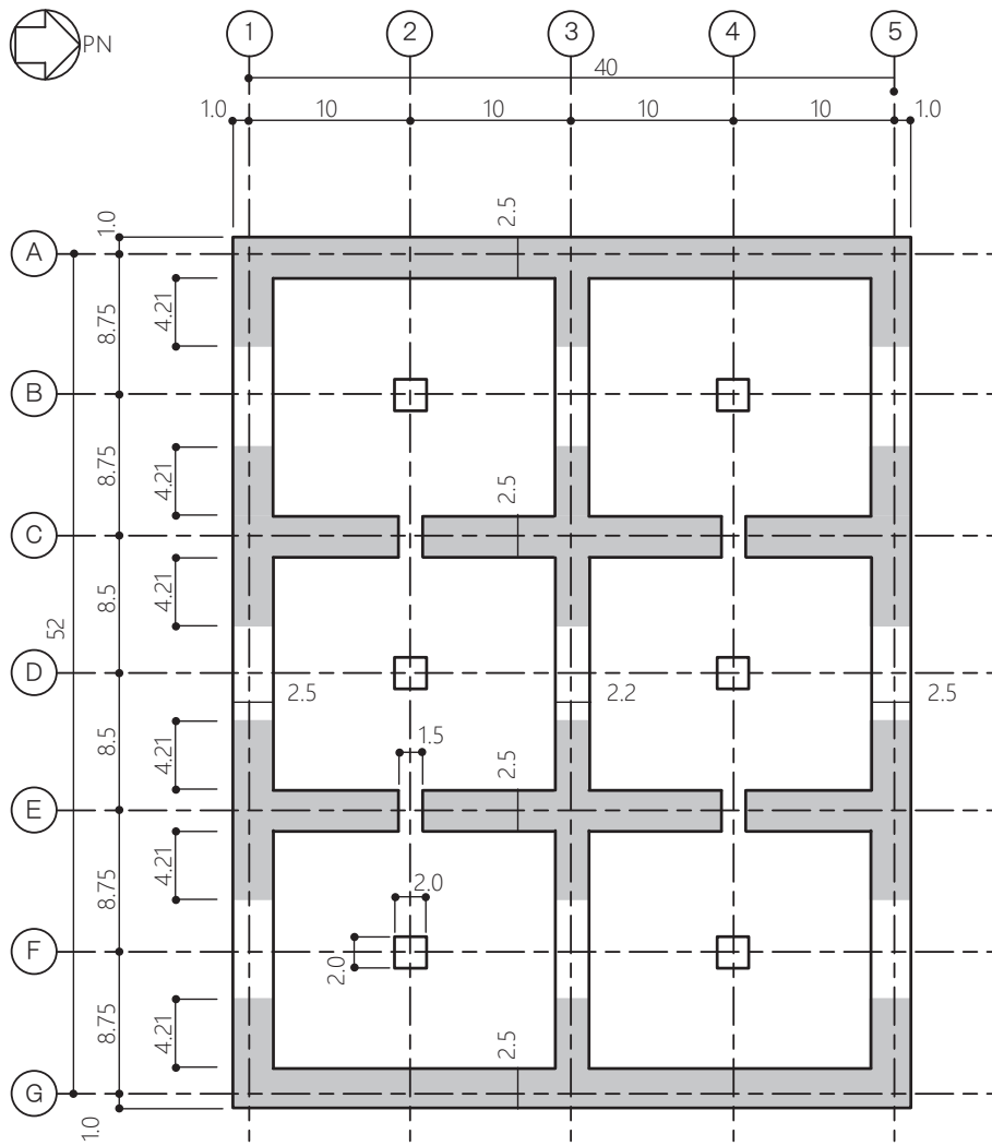
図 2-5 耐震壁の剛性評価範囲 (NS 方向)
