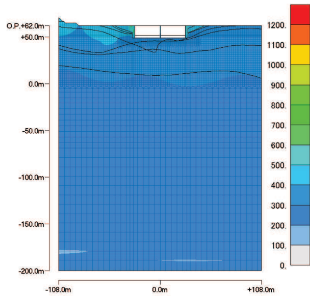
最大加速度分布 (最大値:808.28 cm/s 2 )
