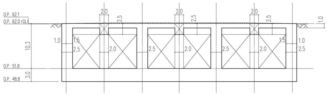
図 2-3 (1) 淡水貯水槽の概略断面図 (A-A 断面 EW 方向)
