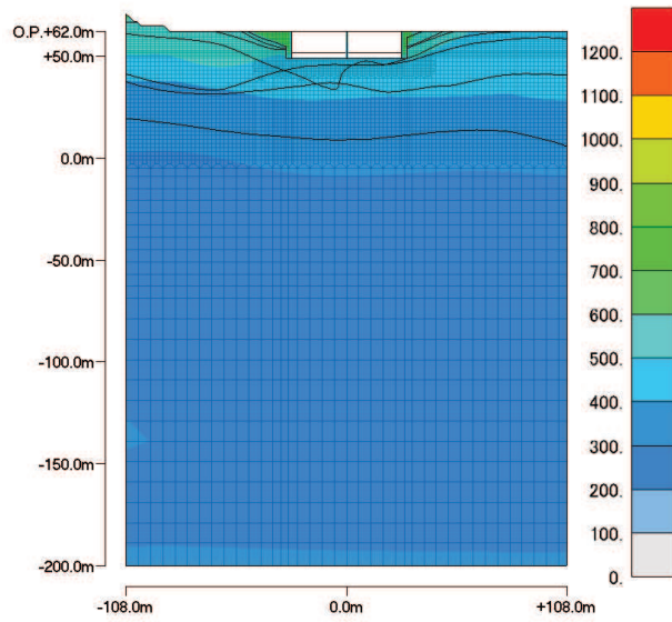
最大加速度分布 (最大値:921.23 cm/s 2 )
