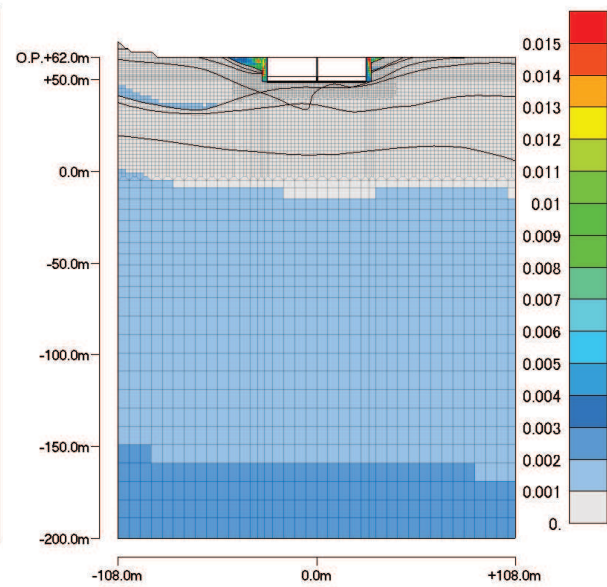
最大ひずみ分布 (最大値:0.01964%)
