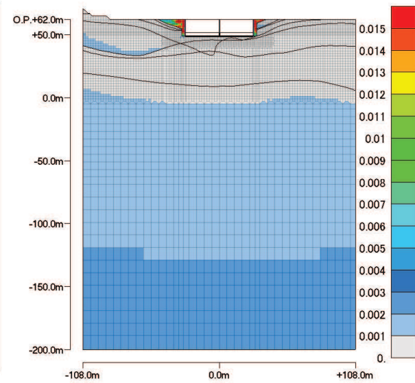
最大ひずみ分布 (最大値:0.04062%)
