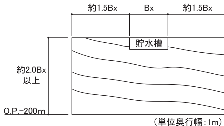
図 2-4 地盤の FEM モデル化範囲
