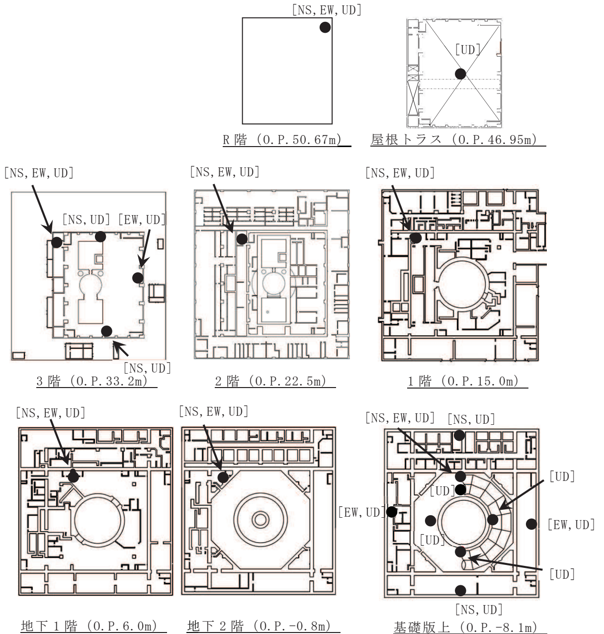
(1) 平面図
