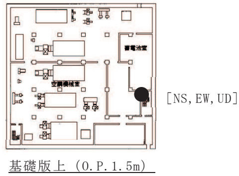
(1) 平面図
