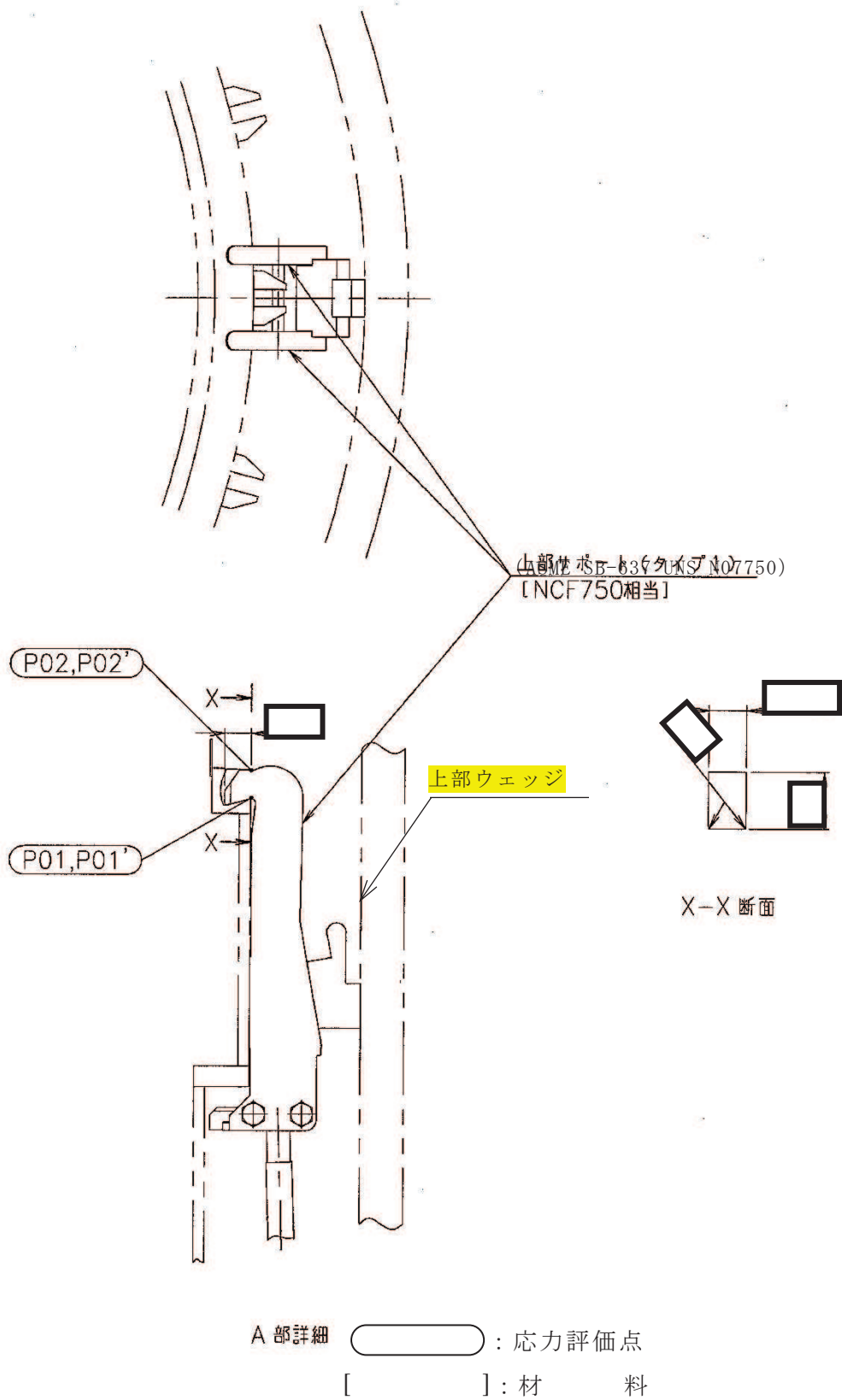
図 1-1(2) 形状・寸法・材料・応力評価点 (単位: mm)
