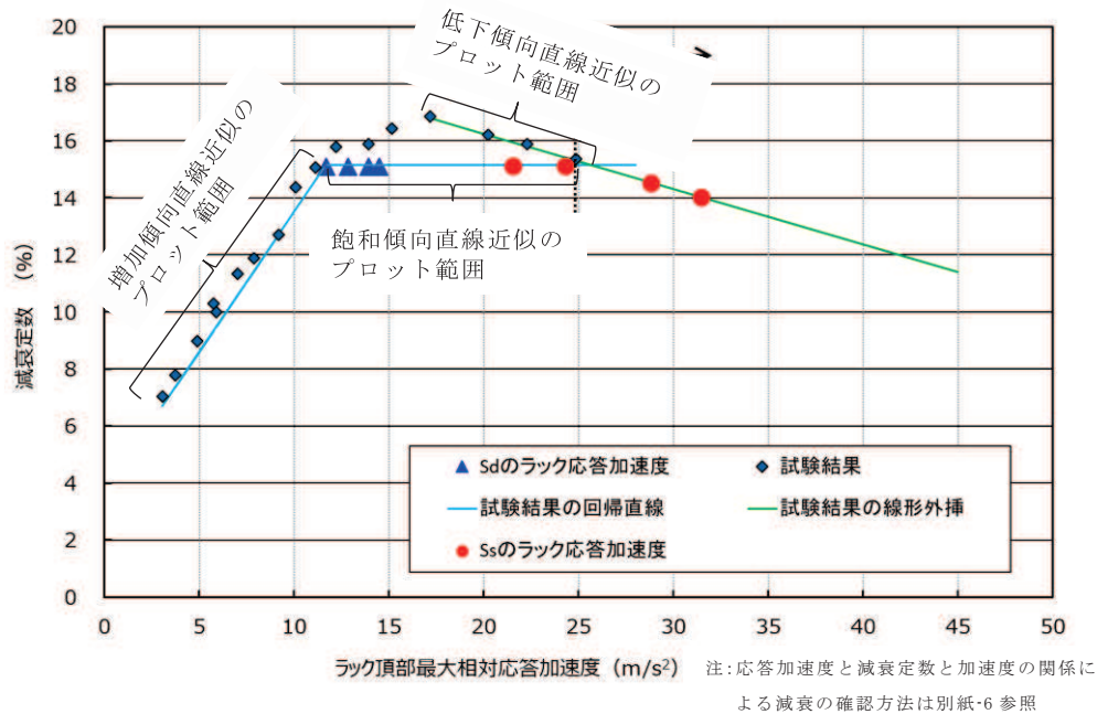
図 5-1 燃料ラック頂部の最大相対応答加速度と減衰定数の関係
