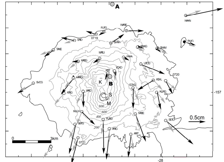
黒矢印: 観測値 灰色矢印: 再現計算結果 (圧力源をA及びBに仮定)
