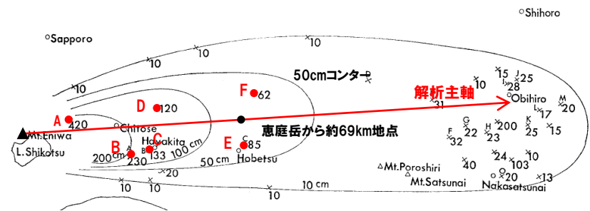
等層厚線図(春日井ほか(1968)に加筆)
