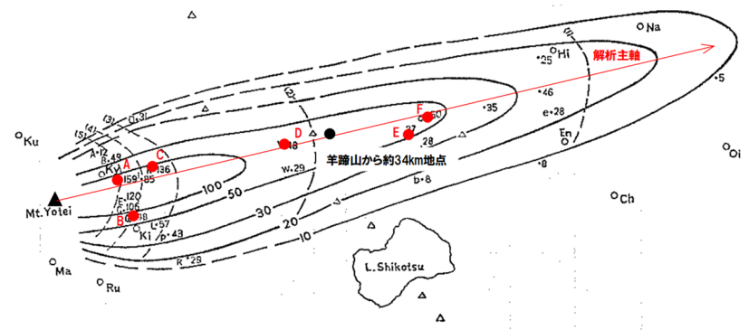
等層厚線図(柏原ほか(1976)に加筆)
