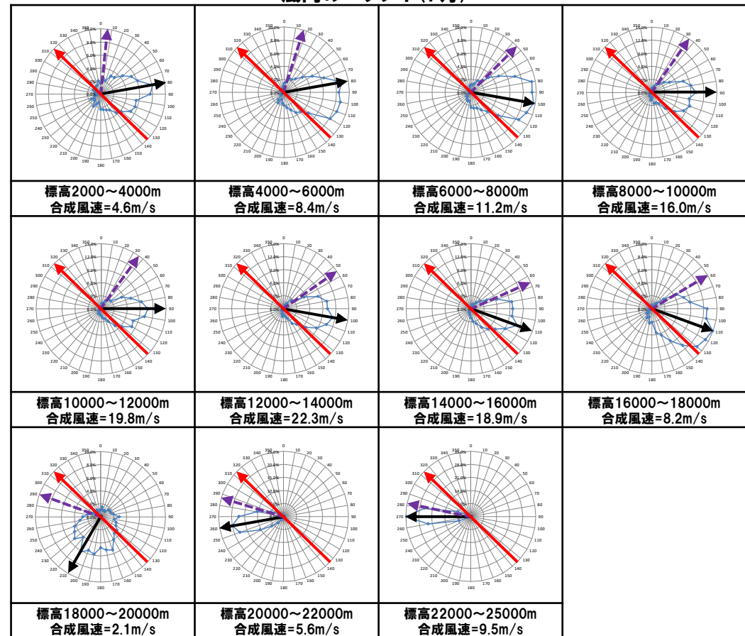
風向のバラツキ (7月)
