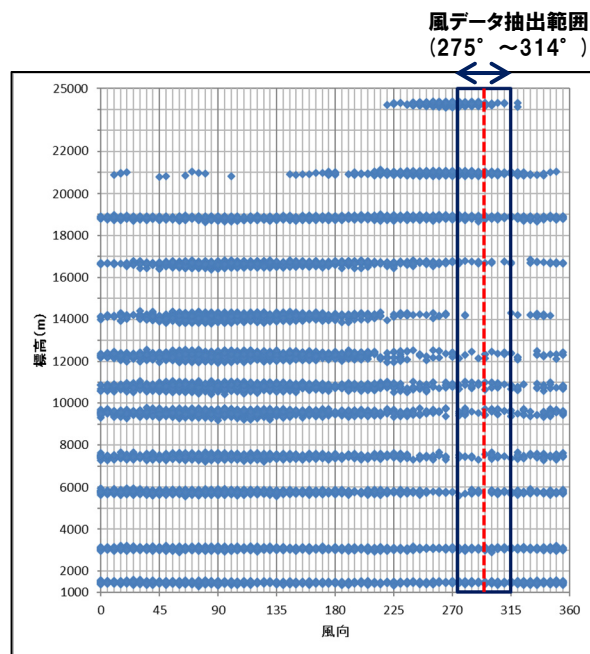
風向データ (7月)
