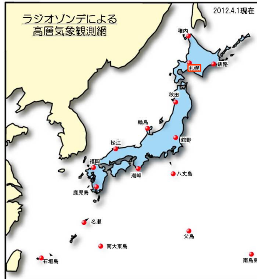
ラジゾンデ打ち上げ位置(気象庁HPより)
