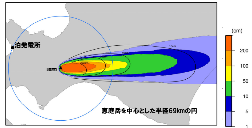
春日井ほか(1968)の等層厚線及び最適ケースの結果
