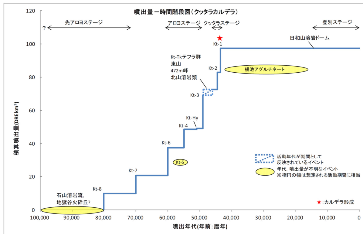
噴出量-年代階段ダイアグラム(山元, 2014)
