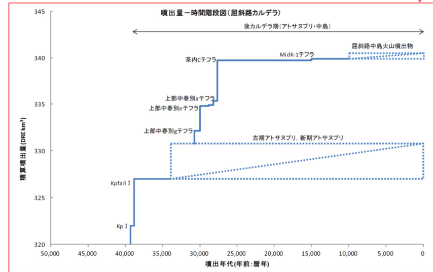
噴出量-年代階段ダイアグラム(山元, 2014)
