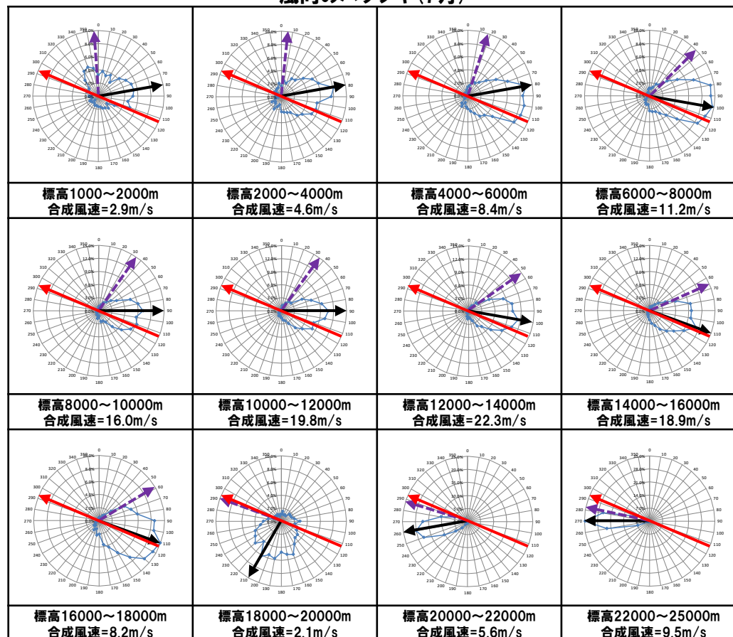
風向のバラツキ(7月)
