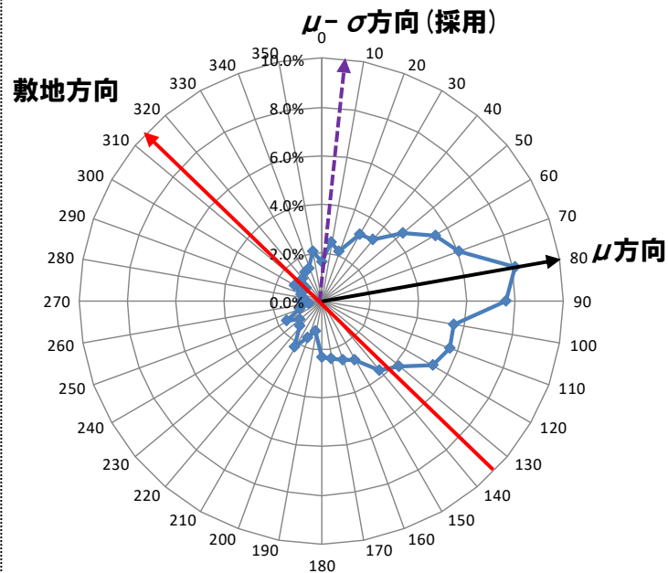
標高2000~4000mの風向頻度分布 (7月)
