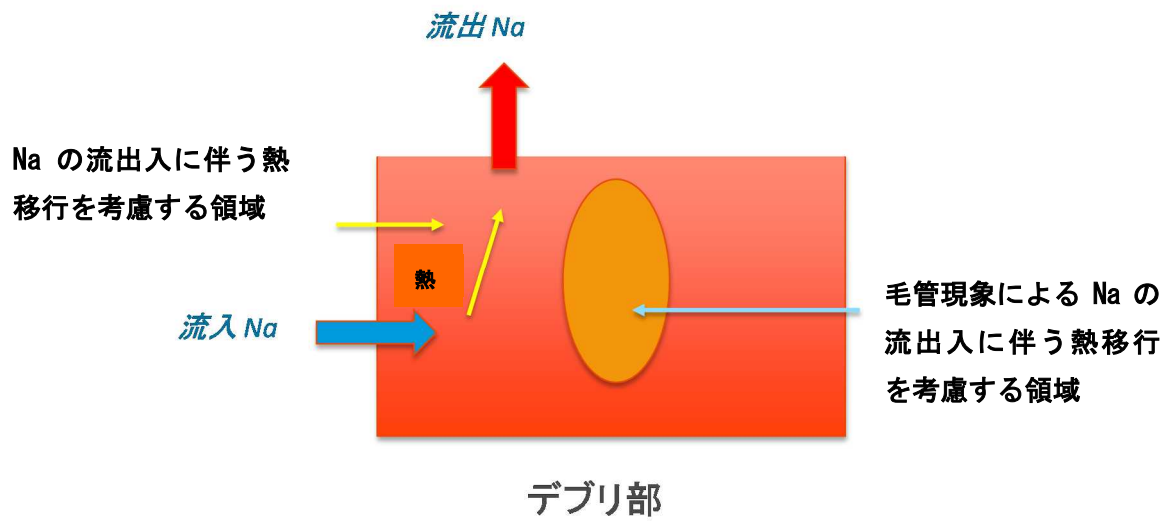
図2 デブリ部の熱流動評価モデル概念
