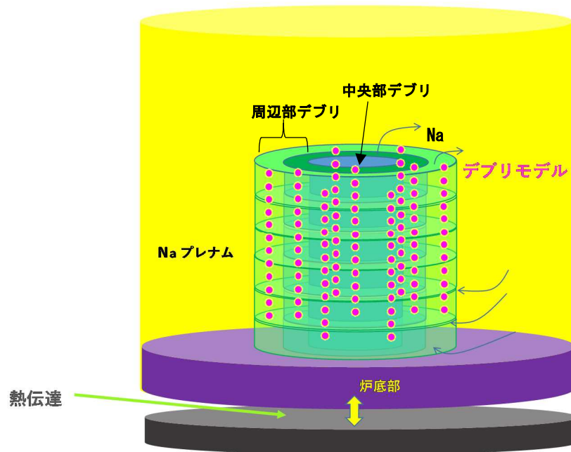
図3 3次元デブリベッド冷却評価モデルの概念
