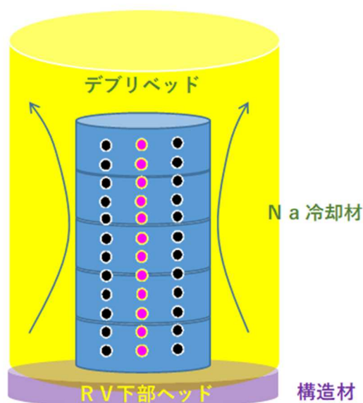
図1 1次元デブリベッド冷却モデルと3次元ナトリウム流動の連成解析モデル
