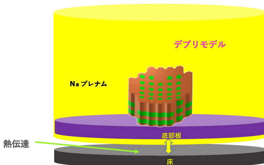
図4 D10 試験の FEM 解析モデル概念
